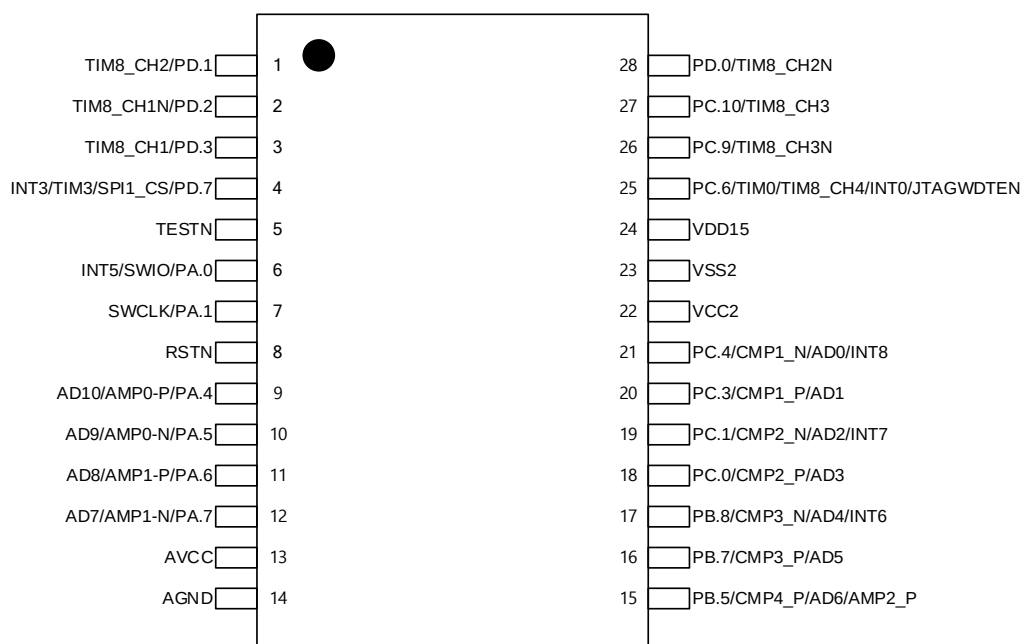
TSSOP28
