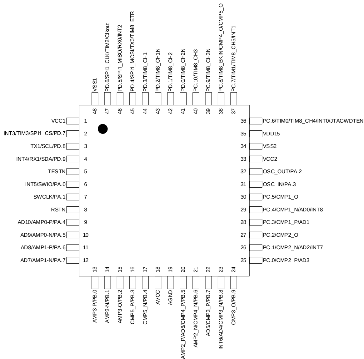
LQFP48
