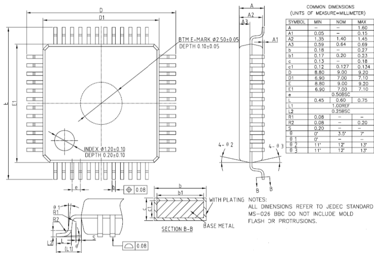
LQFP48
