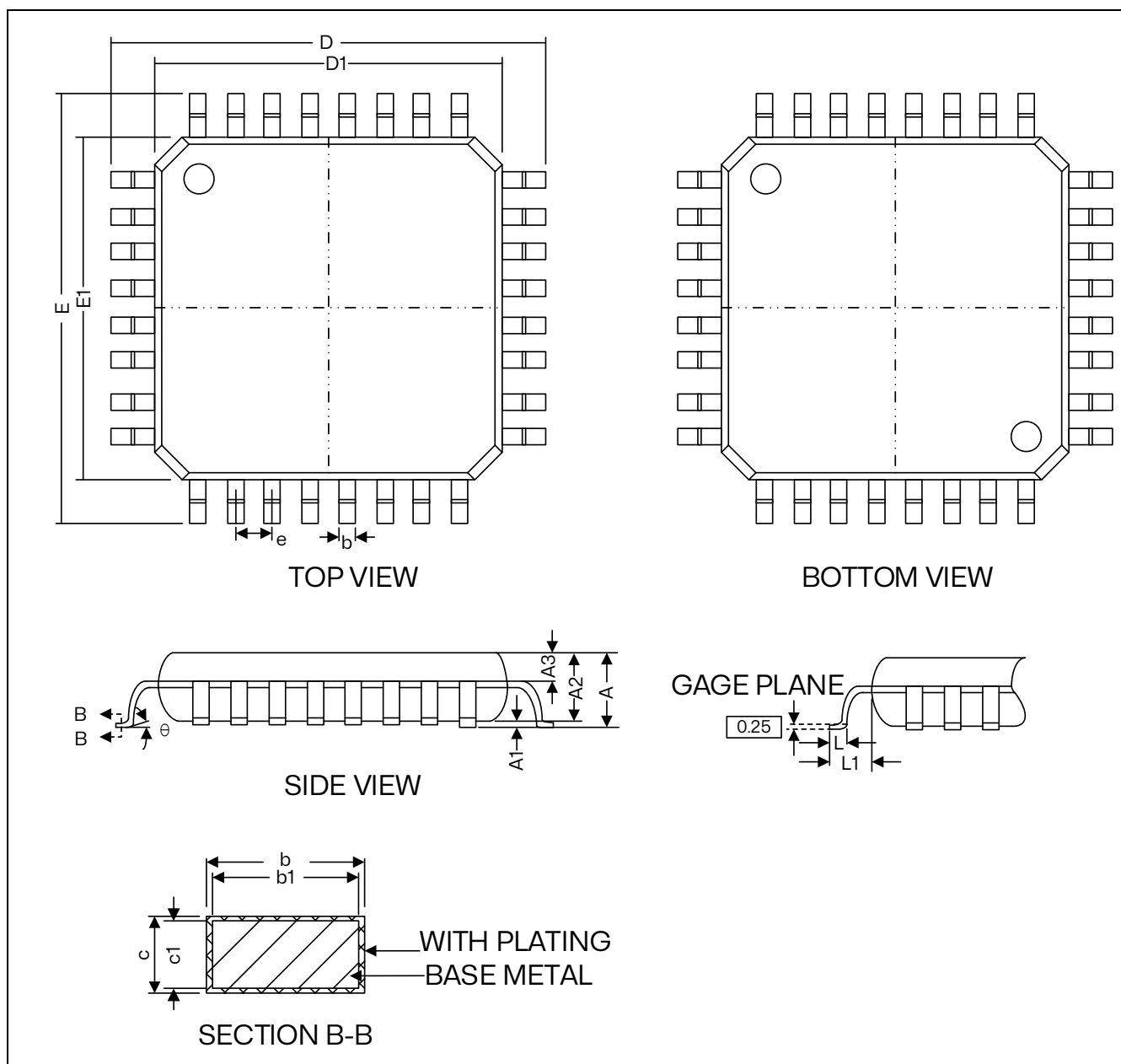
图 6.2 轮廓图
