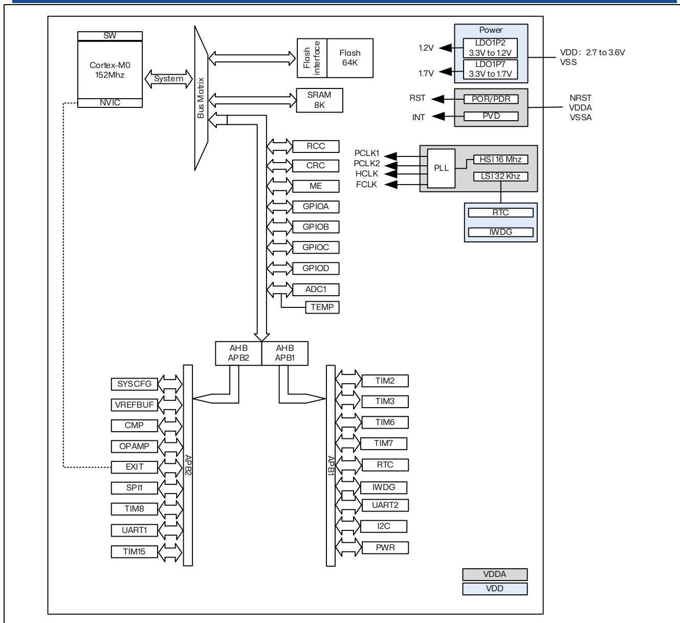
图 2.1 RX32H610 架构图
