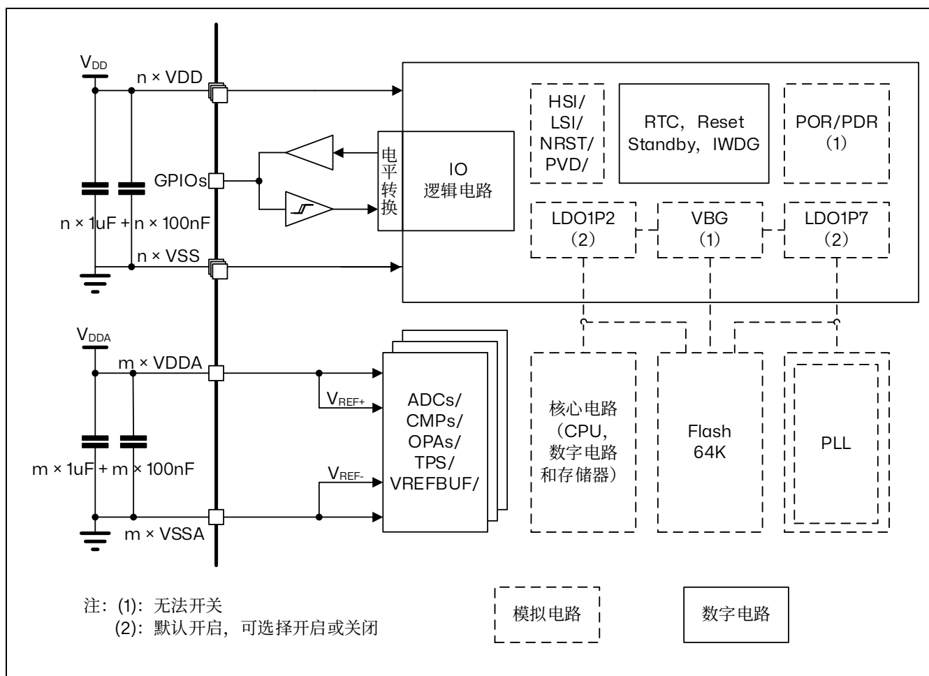
图 5.3 供电方案
