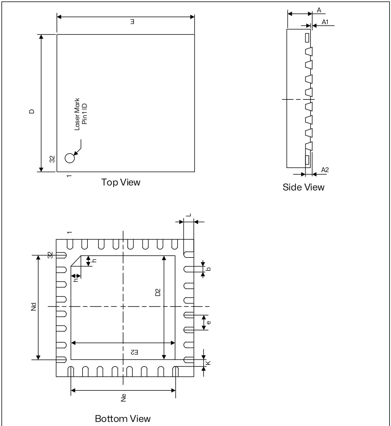
图 6.1 轮廓图
