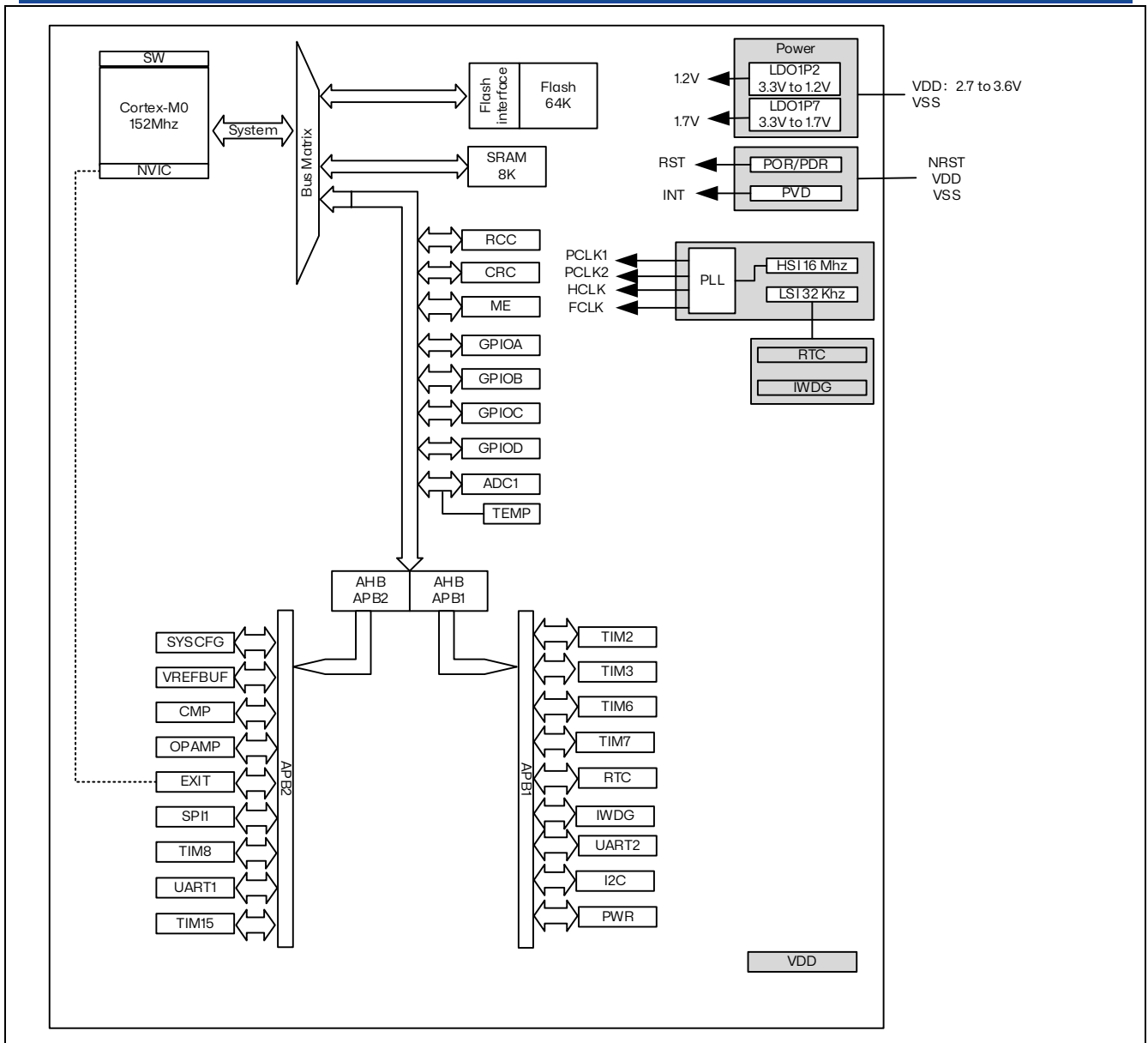
图 2.1 RX32S610 架构图
