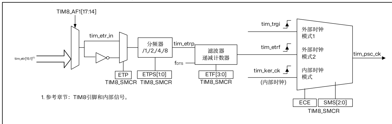
图 14.24 外部触发输入框图
