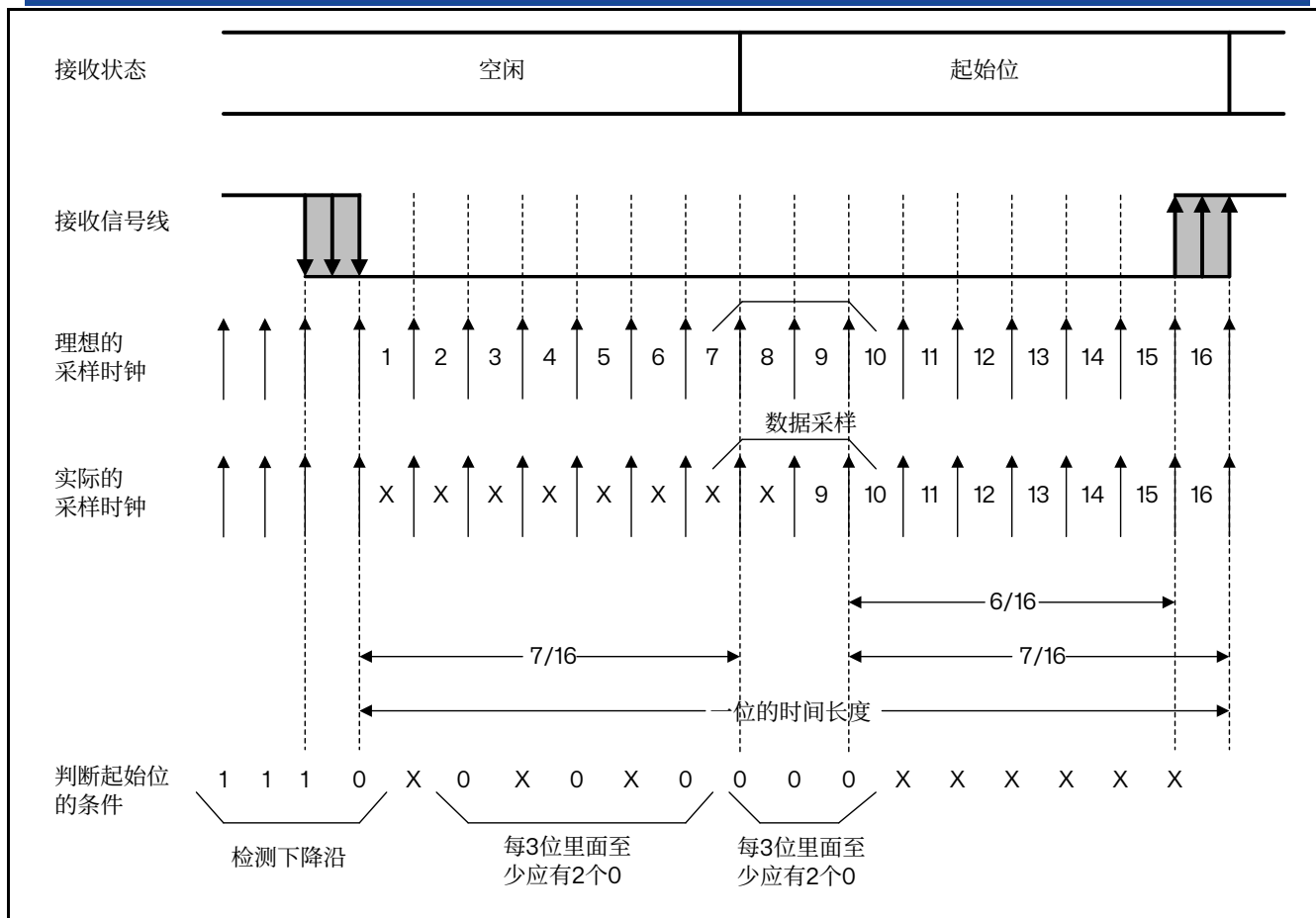
图 25.5 起始位侦测
