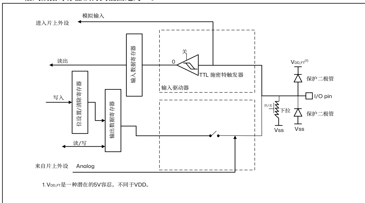
图 8.5 模拟引脚框图
