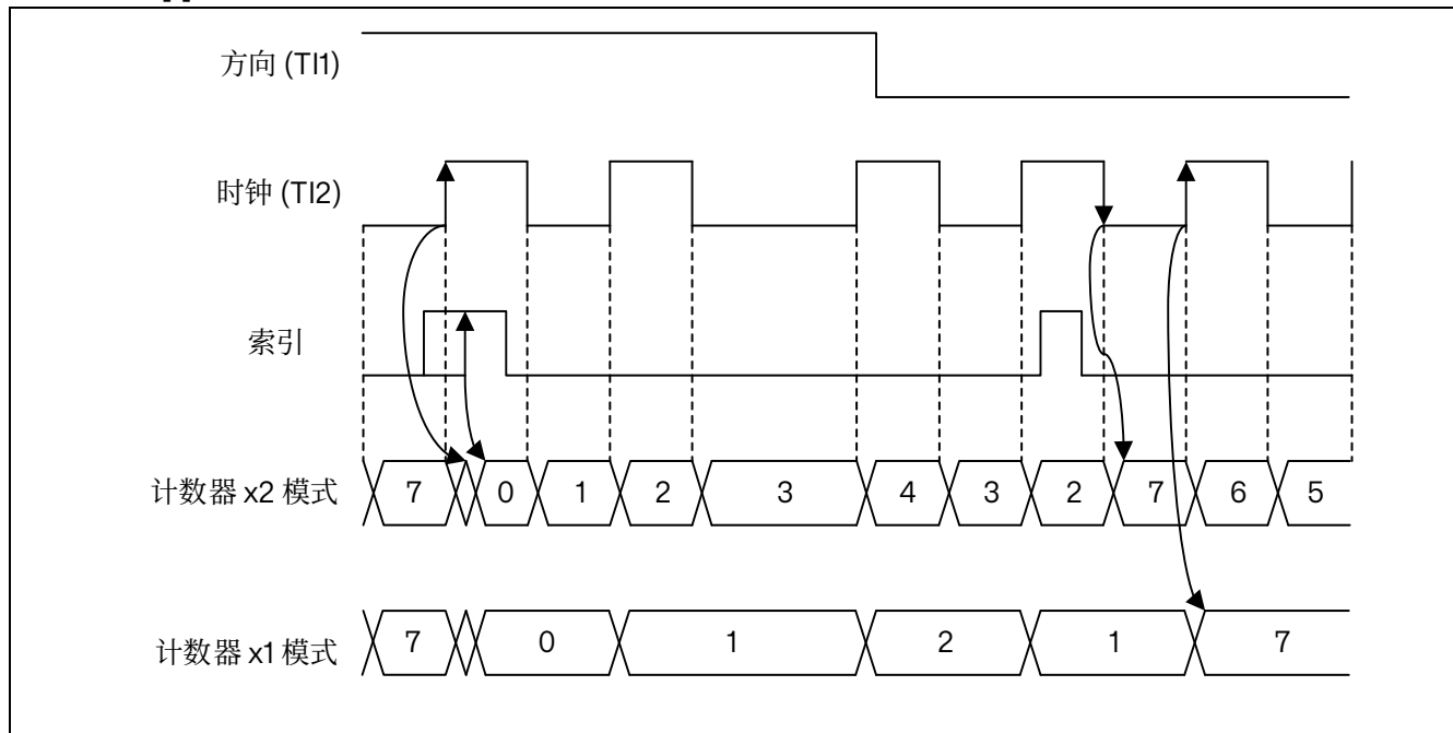
图 15.68 时钟+方向模式下的索引行为, IPOS[0] = 1
