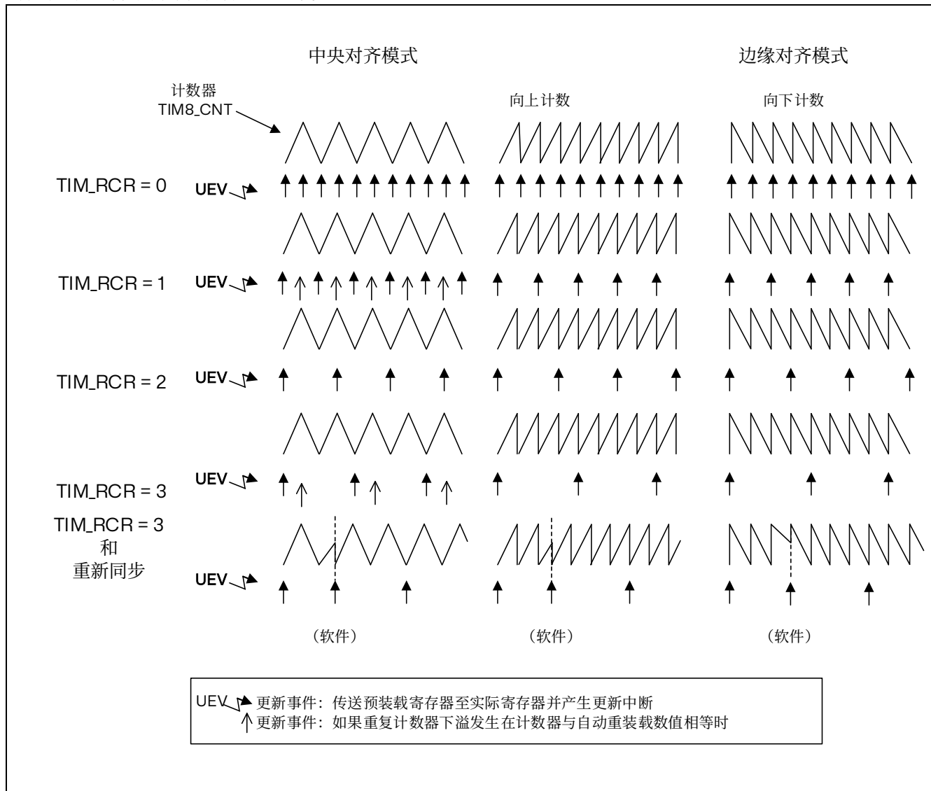
图 14.21 不同模式下更新速率的例子，及 TIM8_RCR 的寄存器设置
