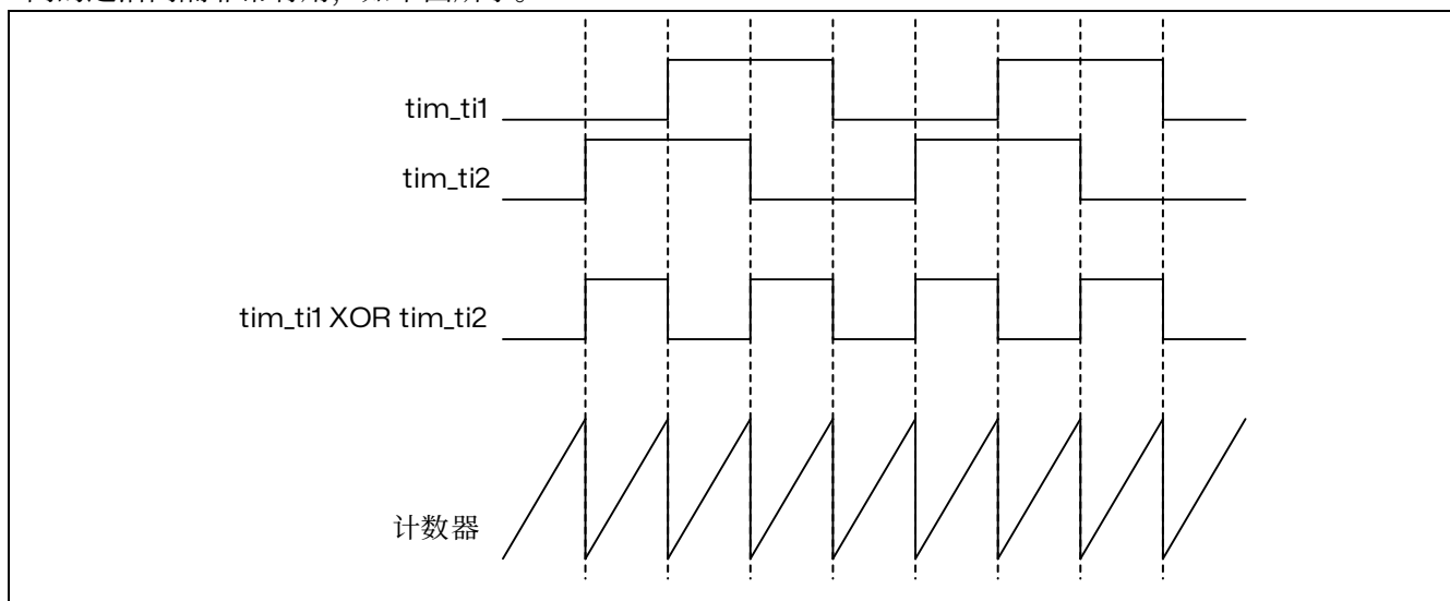
图 16.37 测量两个信号边沿之间的间隔时间
