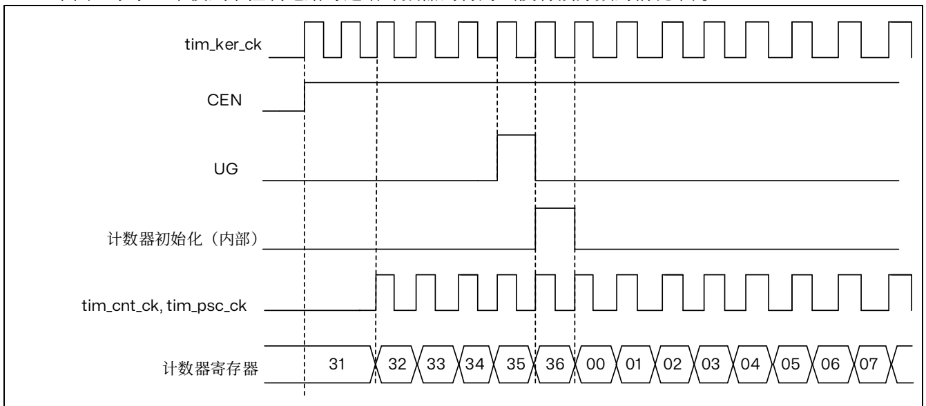
图 14.23 一般模式下的控制电路，内部时钟分频因子为 1
