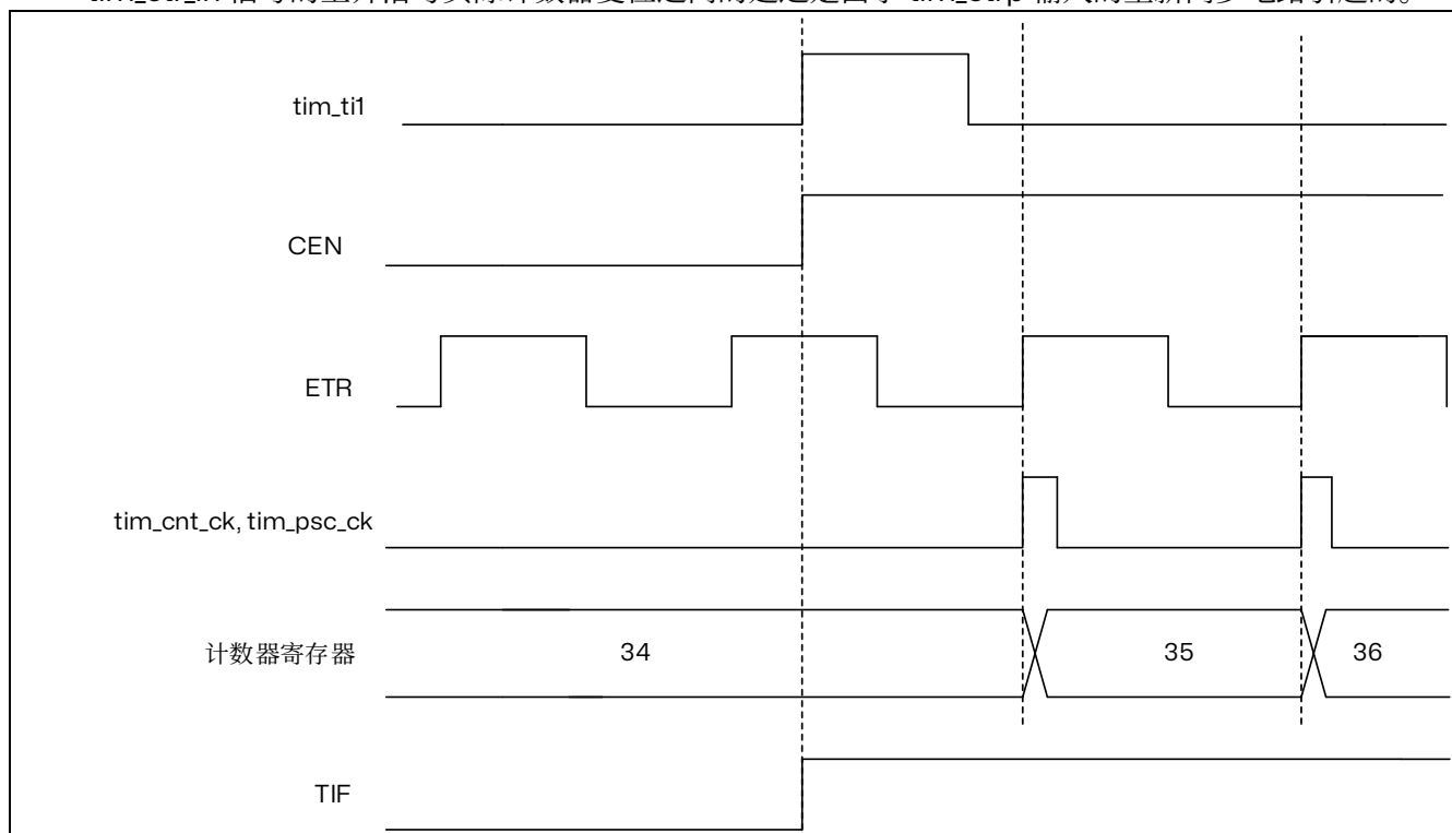
图 15.77 外部时钟模式 2+触发模式下的控制电路
