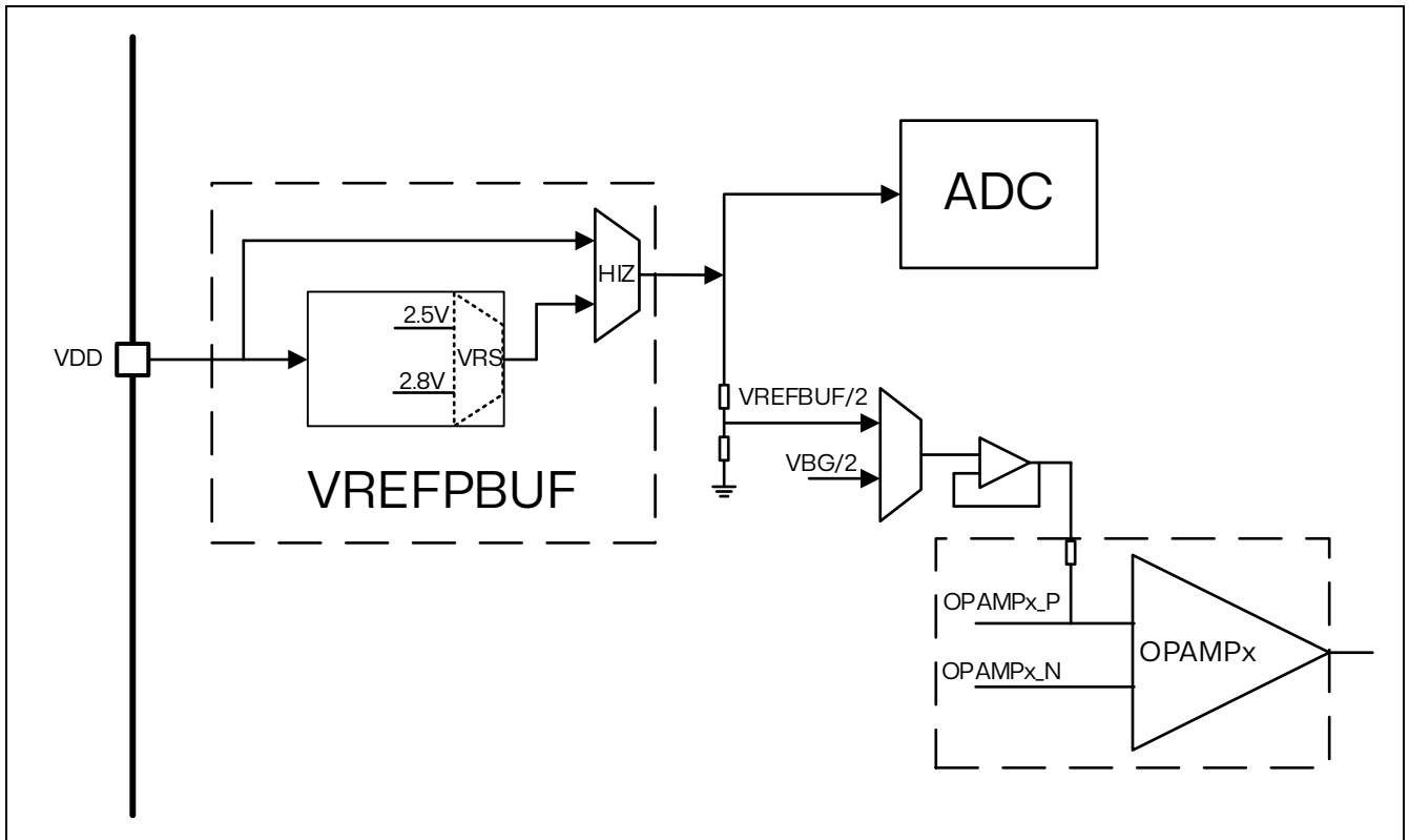
图 12.1 VREFBUF 框图
