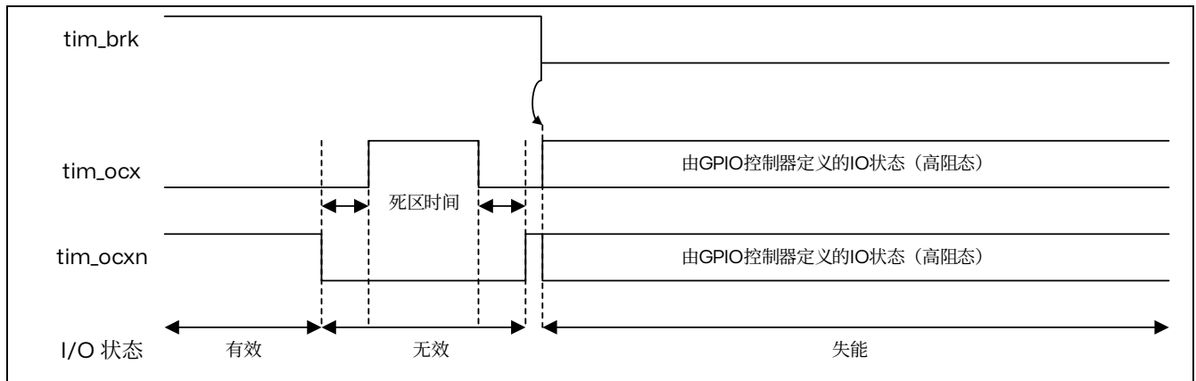
图 14.49 当 tim_brk/tim_brk2 有效 (OSS1=0) 时 PWM 输出状态
