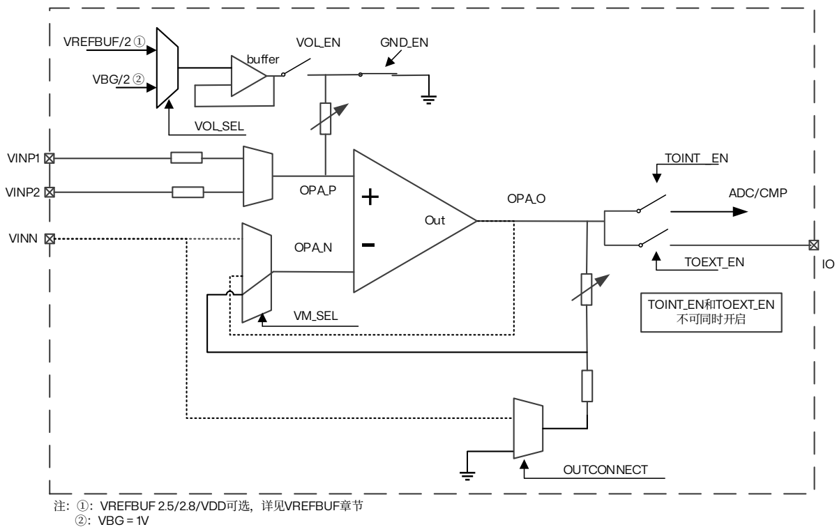
图 18.7 OPAMP3 PGA 模式 (P-IO, N-GND)
