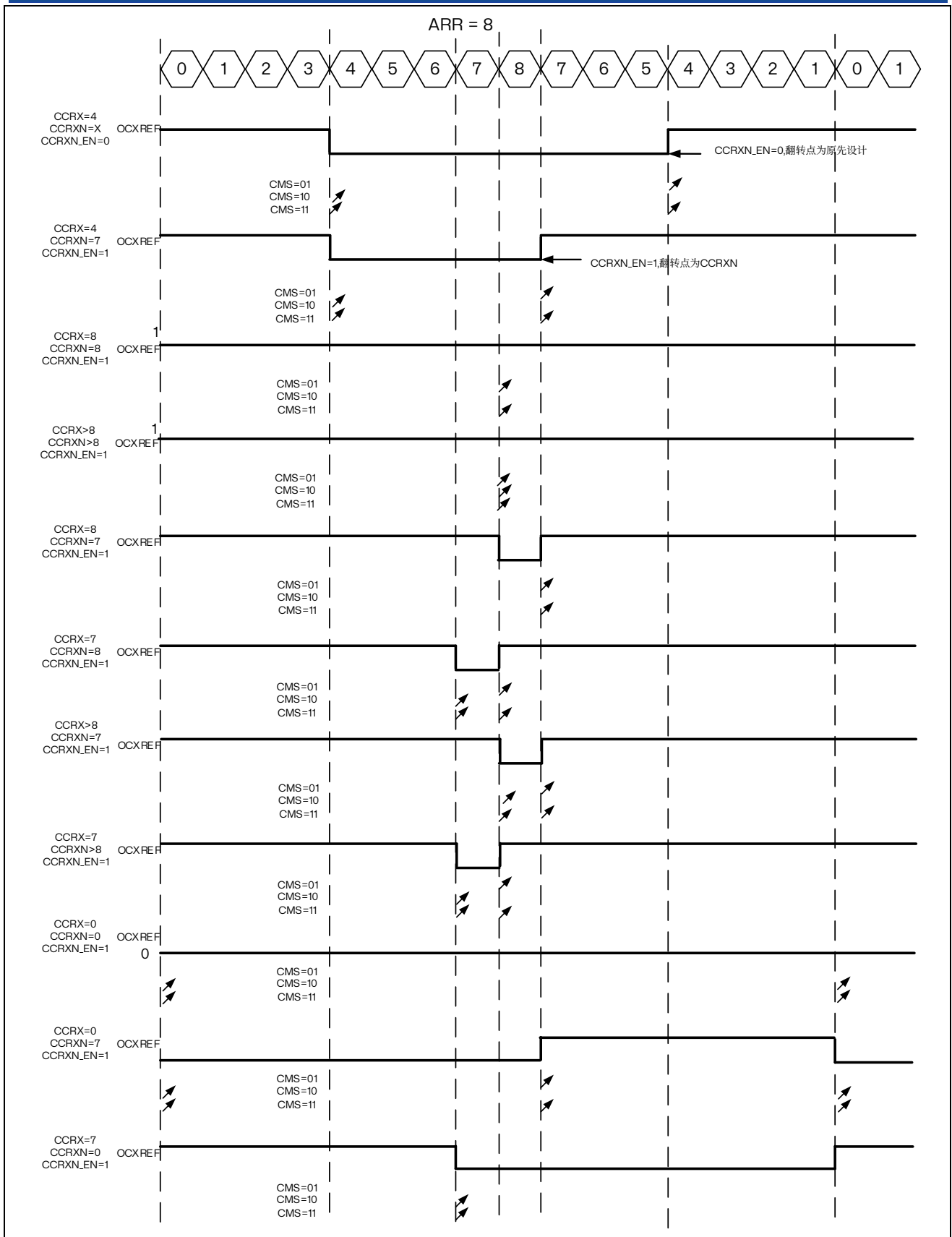
图 14.40 中央对齐的 PWM 波形 (ARR=8)
