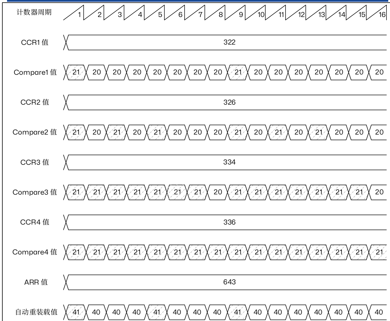
图 14.35 PWM 抖动模式
