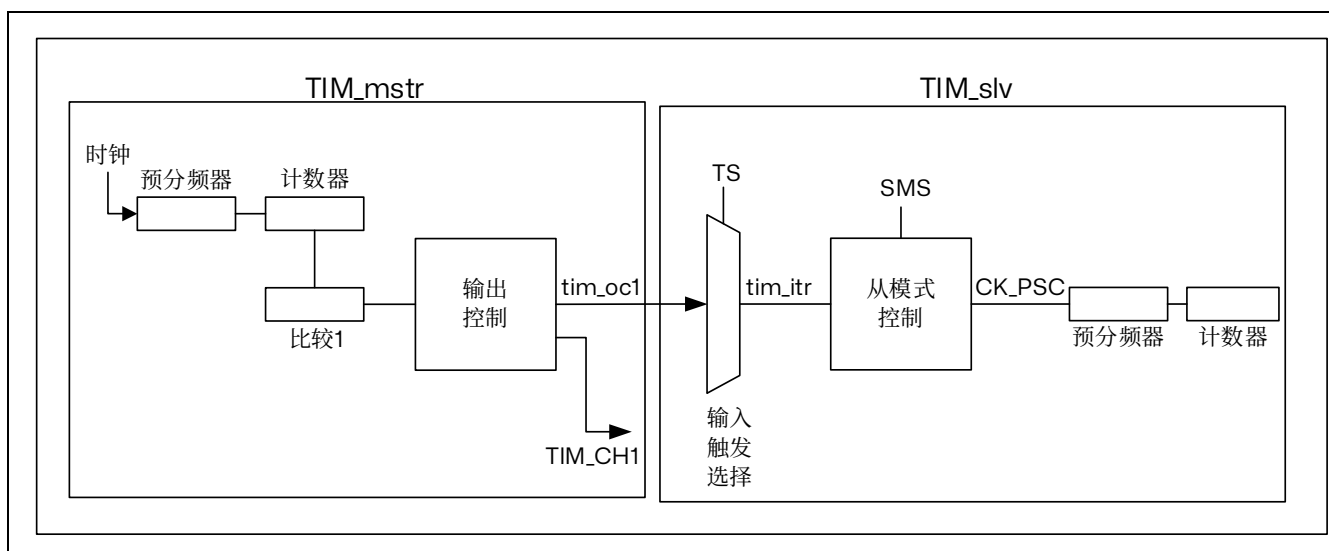
图 15.79 仅定时器通道 1 主/从连接示例
