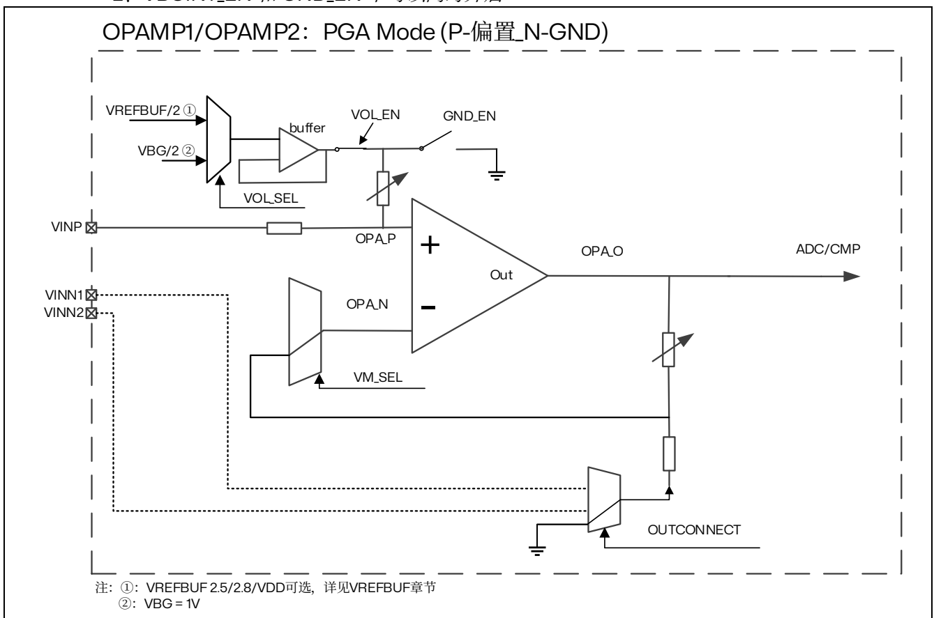
图 18.8 OPAMP1/OPAMP2 PGA 模式 (P-偏置, N-GND)
