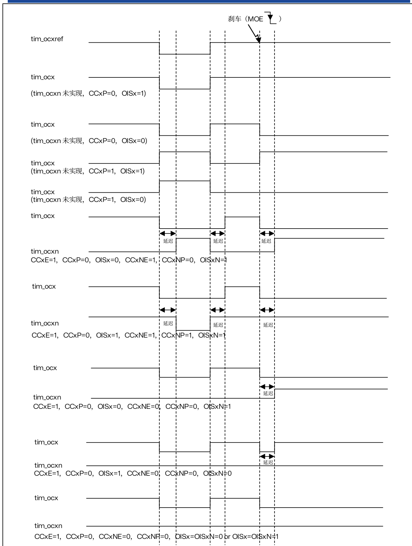
图 14.48 tim_brk 在发生刹车事件时的各种输出行为 (OSS1=1)
