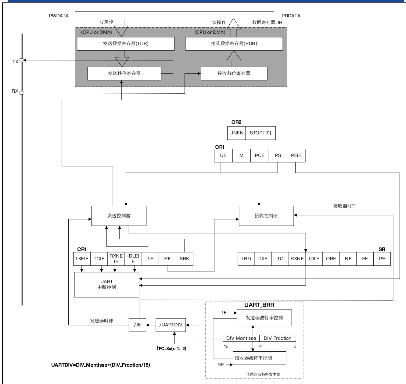
图 25.1 UART 框图
