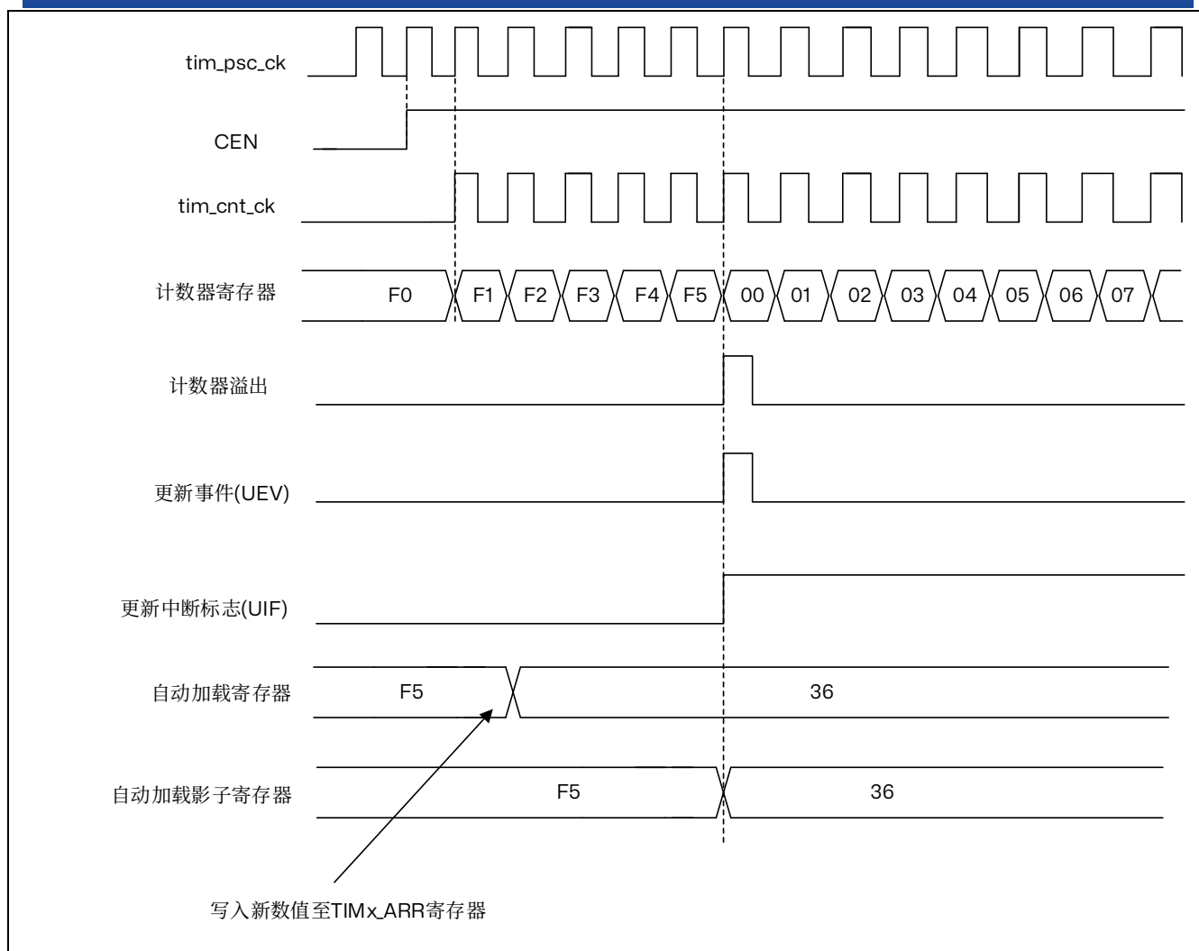
图 17.10 计数器时序图，当 ARPE=1 时的更新事件（预装入了 TIMx_ARR）
