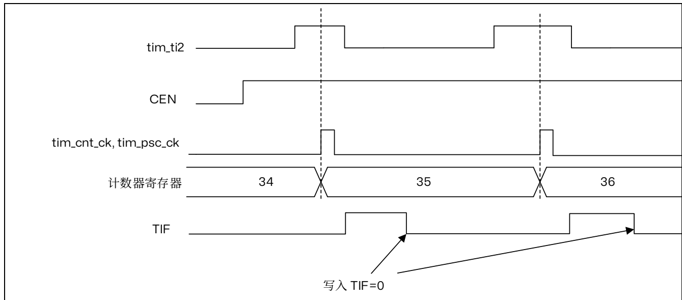
图 15.23 外部时钟模式 1 下的控制电路
