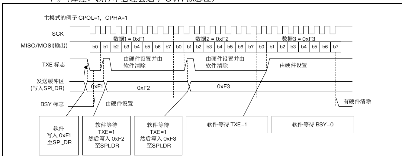
图 23.7 主设备只发送模式 (BIDIMODE=0 并且 RXONLY=0) 下连续传输时，TXE/BSY 变化示意图
