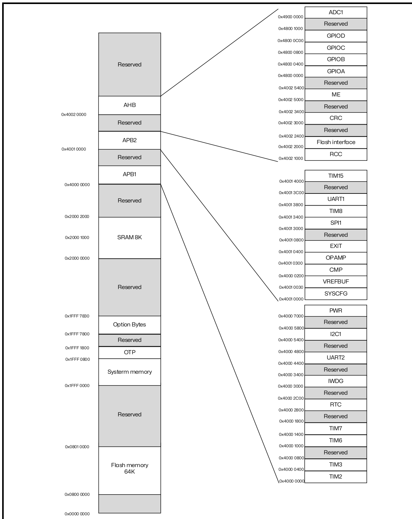
图 3.1 存储器映像
