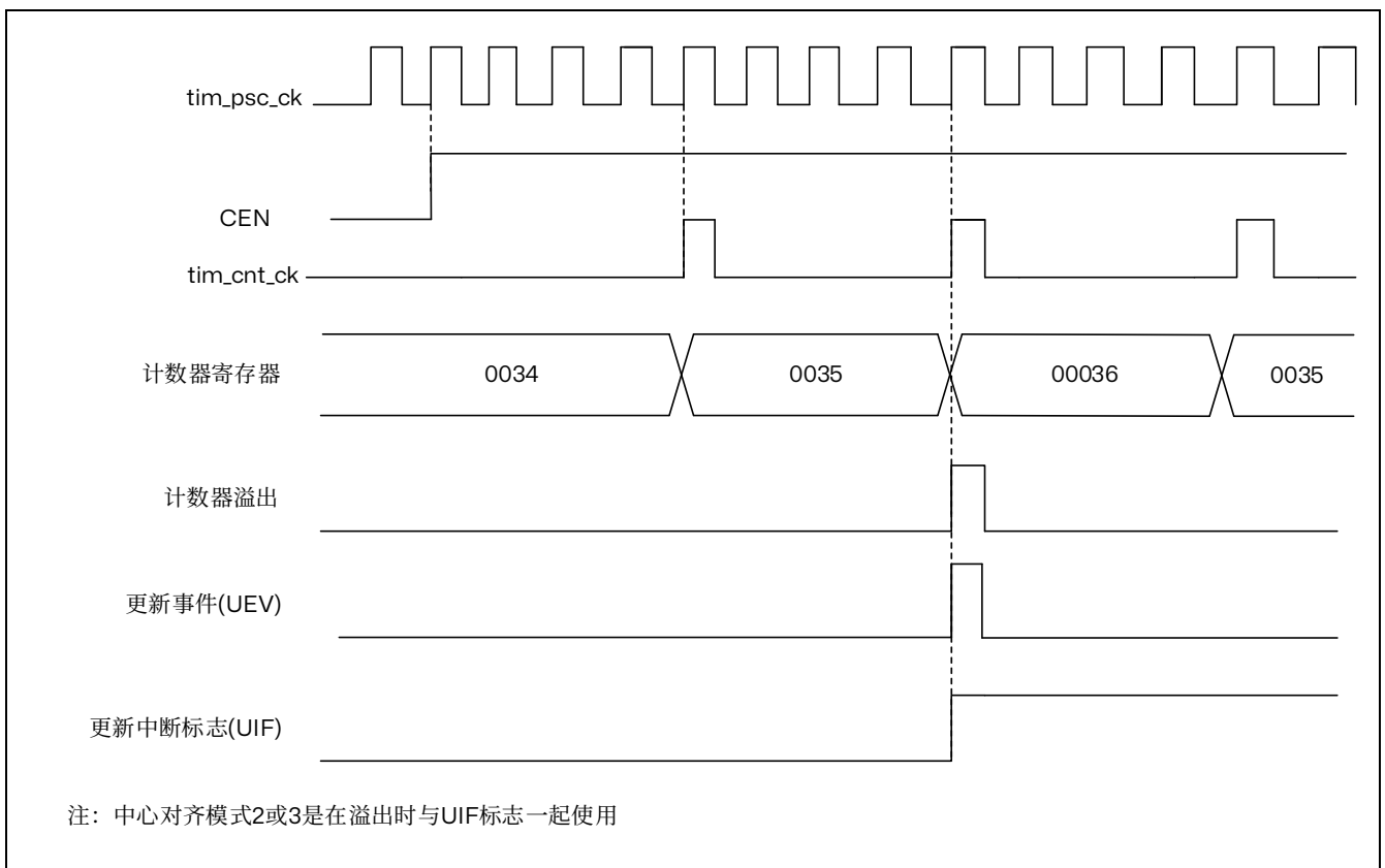
图 15.18 计数器时序图，内部时钟分频因子为 4，TIMx_ARR=0x36
