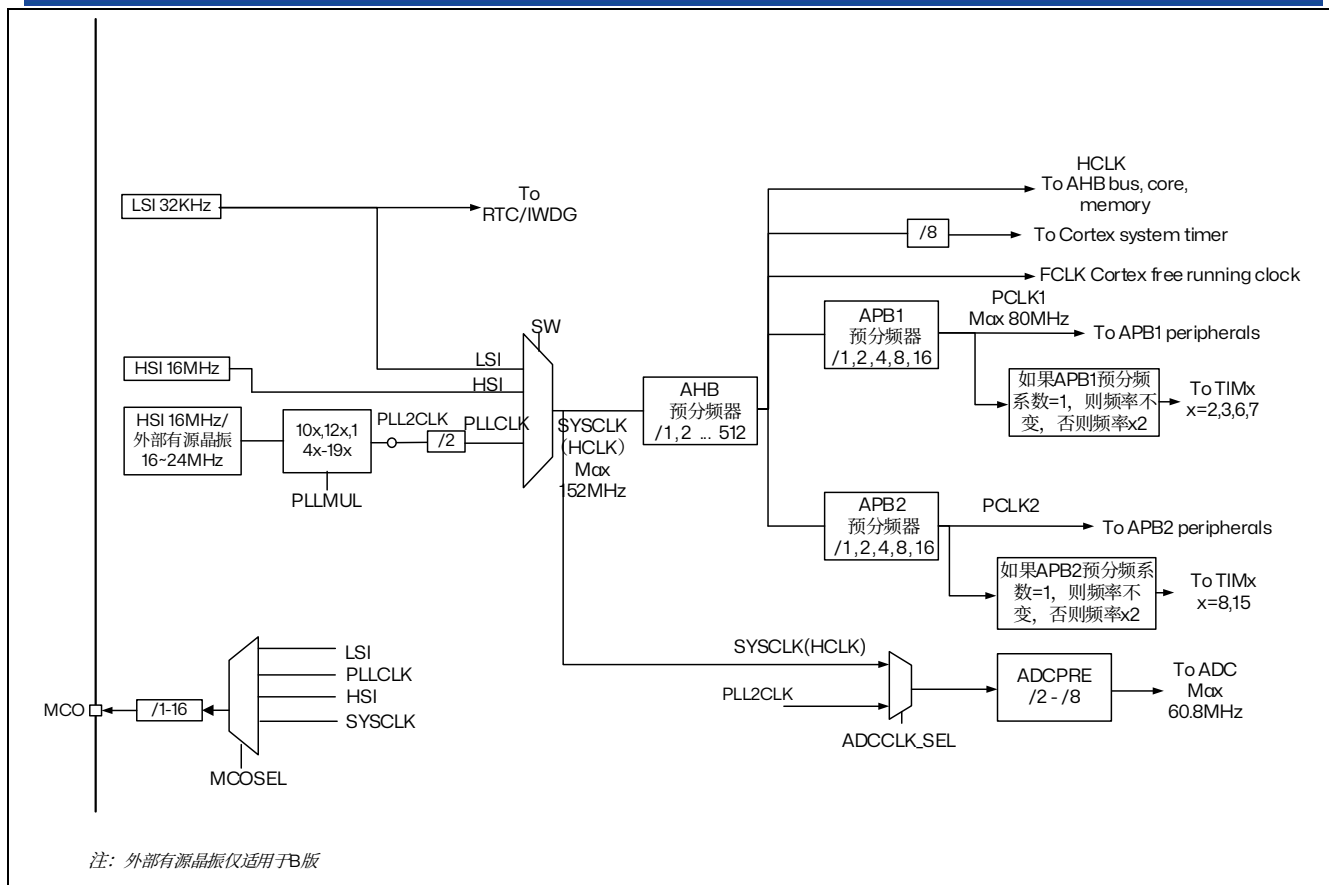
图 7.2 时钟树
