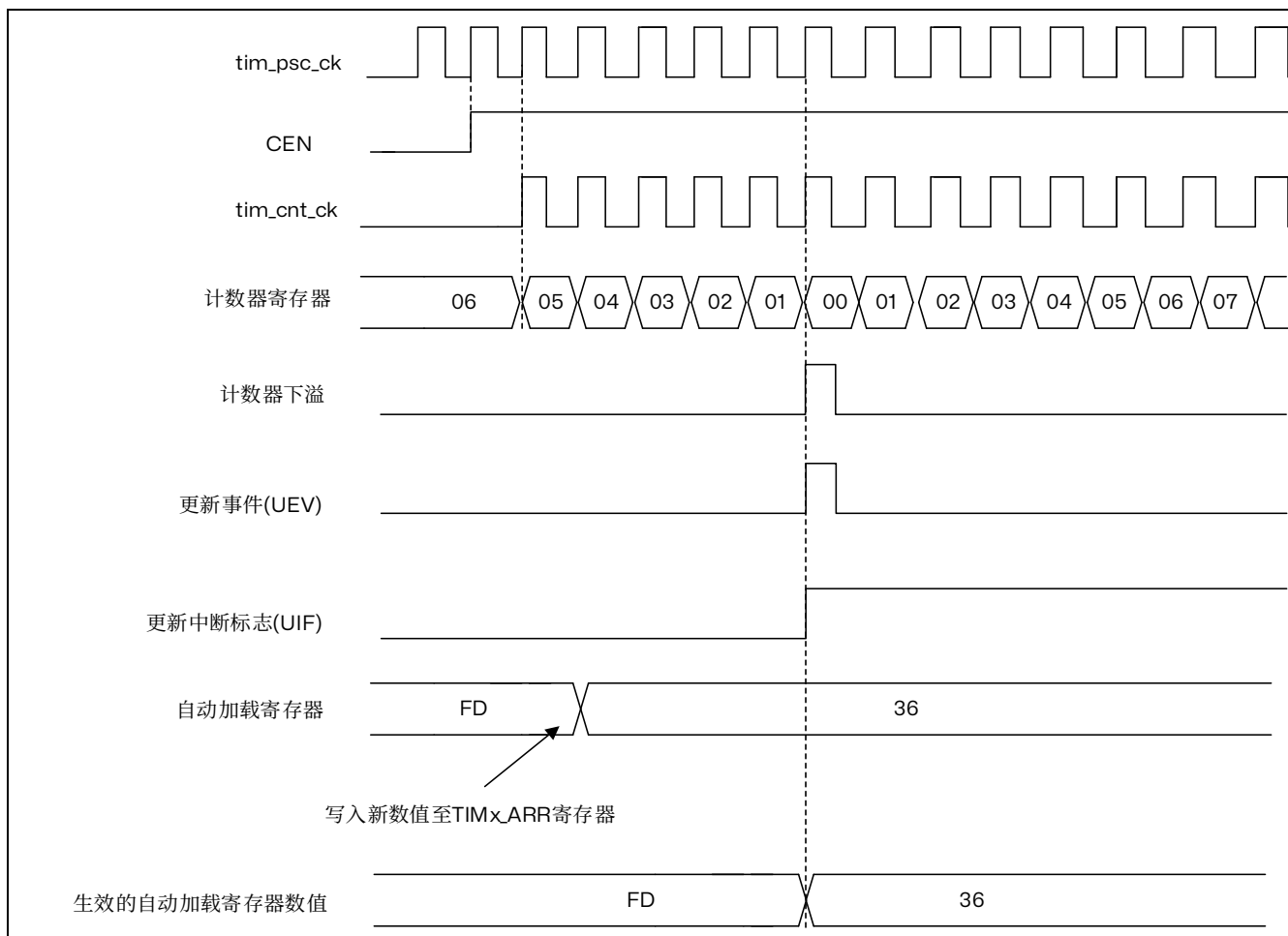
图 15.19 计数器时序图，内部时钟分频因子为 N
