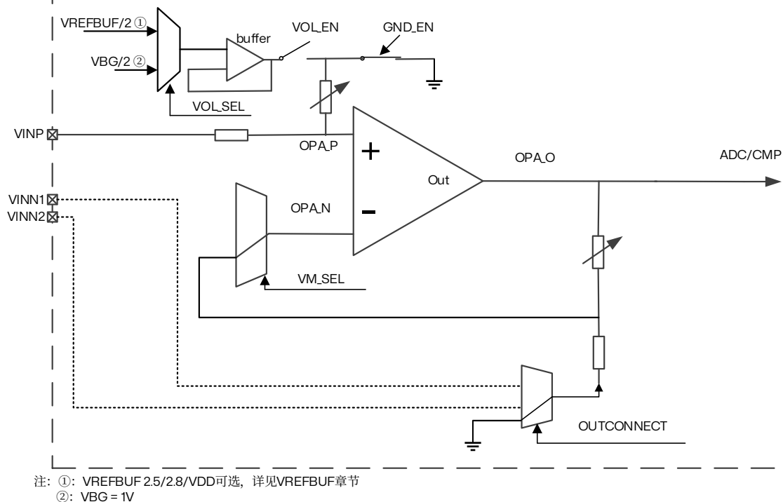
图 18.6 OPAMP1/OPAMP2 PGA 模式 (P-IO, N-GND)
