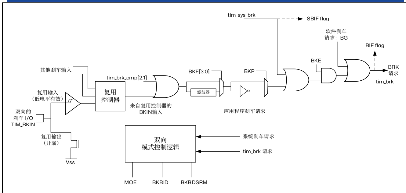
图 16.32 输出重定向
