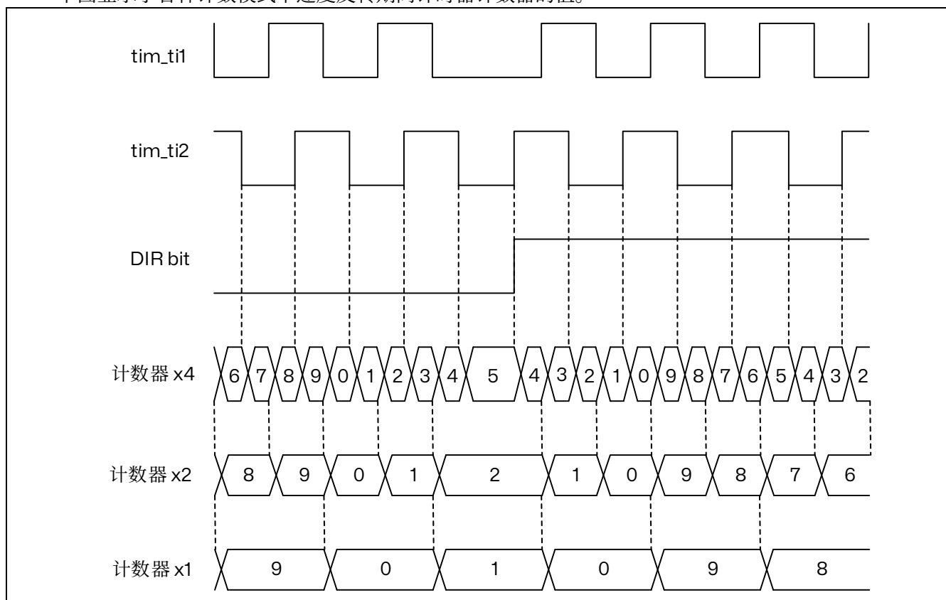
图 15.54 正交编码器的计数模式
