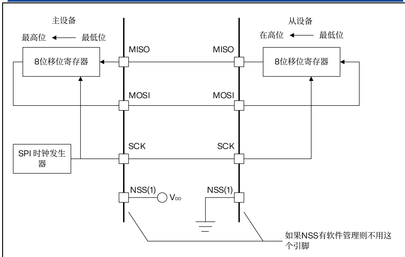
图 23.2 单主和单从应用
