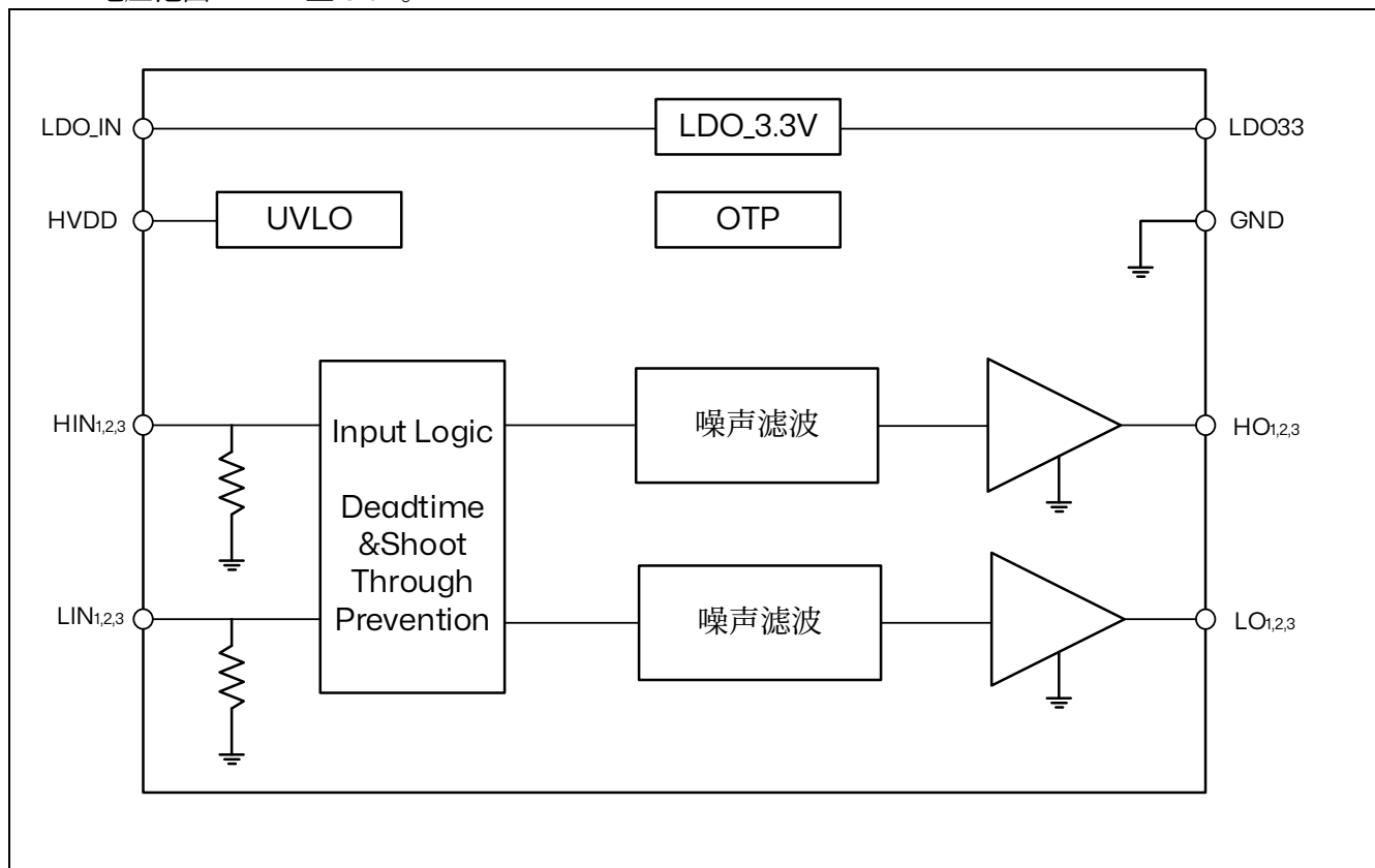
图 26.1 GateDriver 内部结构
