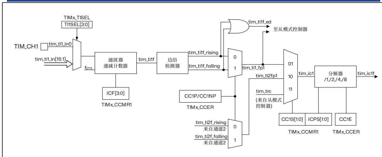
输出阶段生成一个中间波形作为基准：OCxRef（高电平有效）。链的末端决定最终输出信号的极性。 图 15.27 捕获/比较通道（如：通道 1 输入部分）
