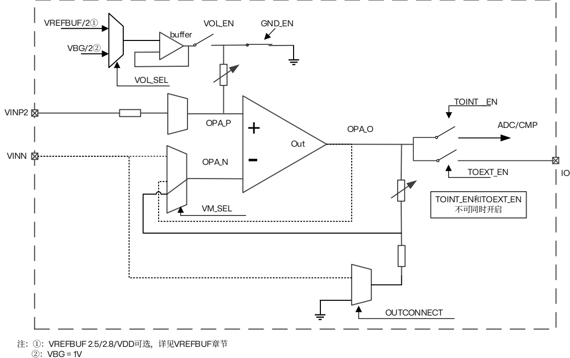
图 18.7 OPAMP3 PGA 模式 (P-IO, N-GND)
