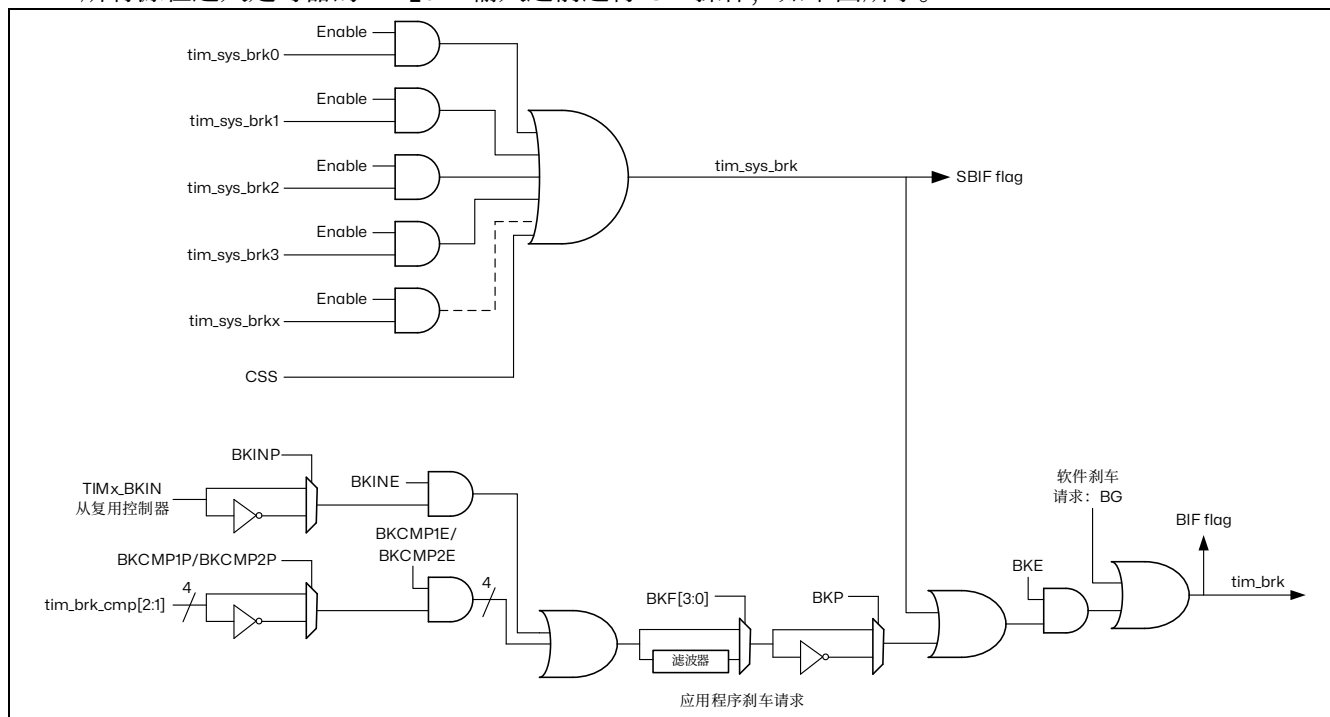
图 16.30 刹车电路概述
