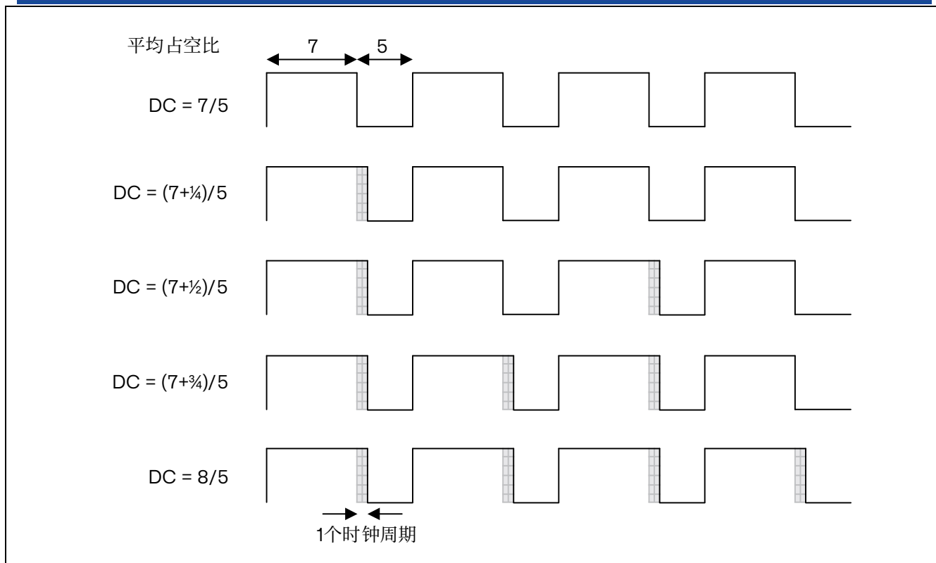
图 16.21 抖动原理
