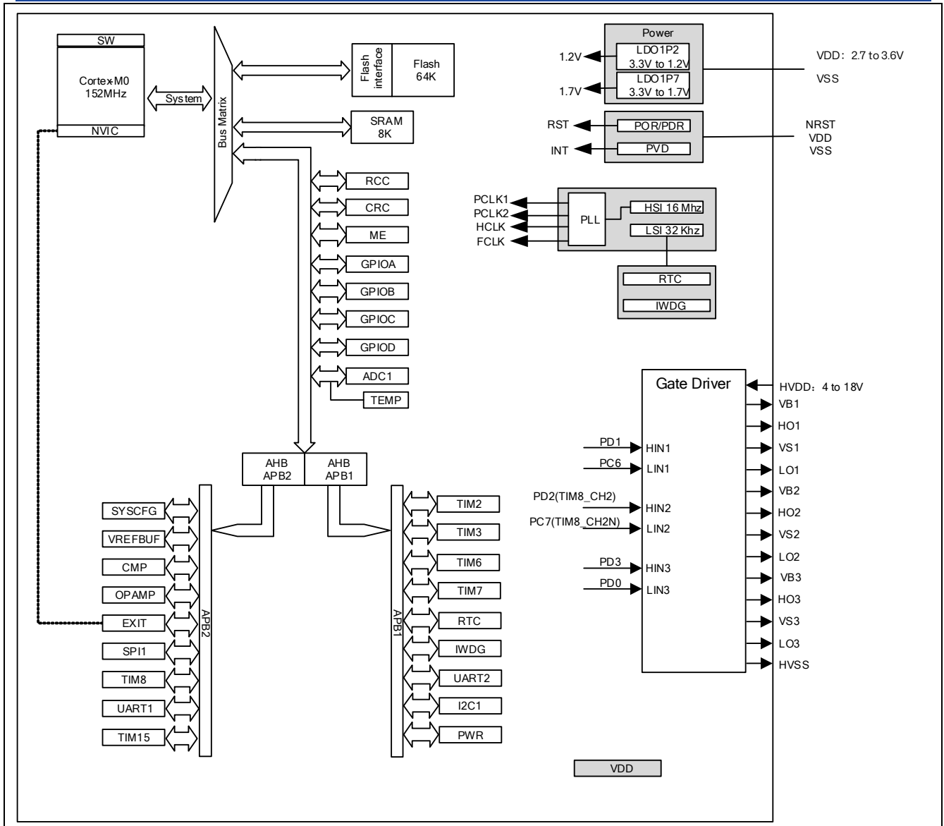
图 2.1 RX32S651 架构图
