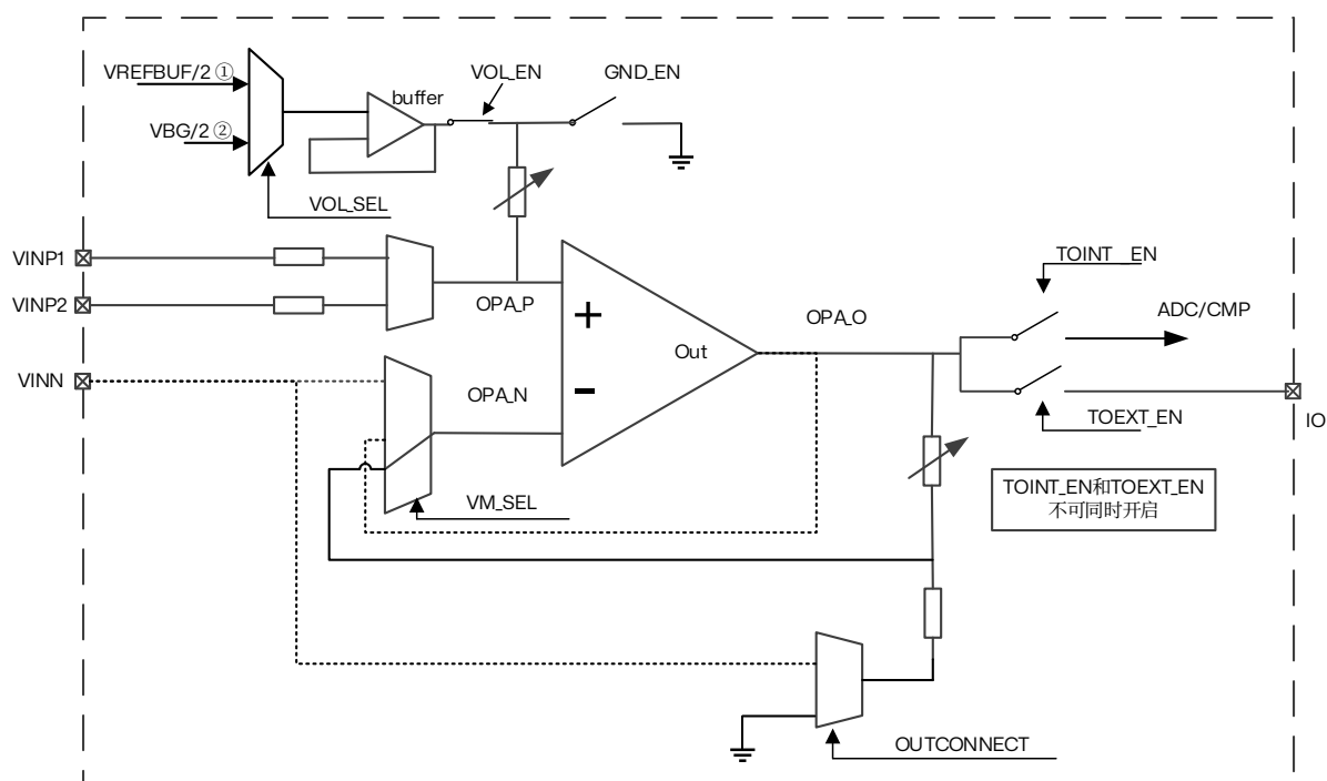
图 18.9 OPAMP3 PGA 模式 (P-偏置, N-GND)
