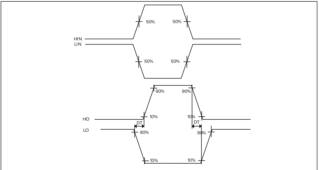
图 26.2 死区时间波形图
