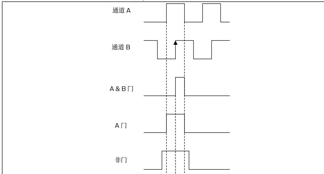
图 15.57 索引门控选项
