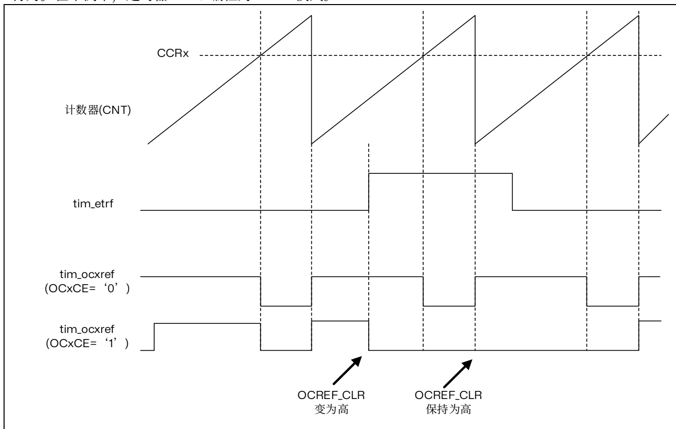
图 14.52 清除 TIM8 的 tim_ocxref
