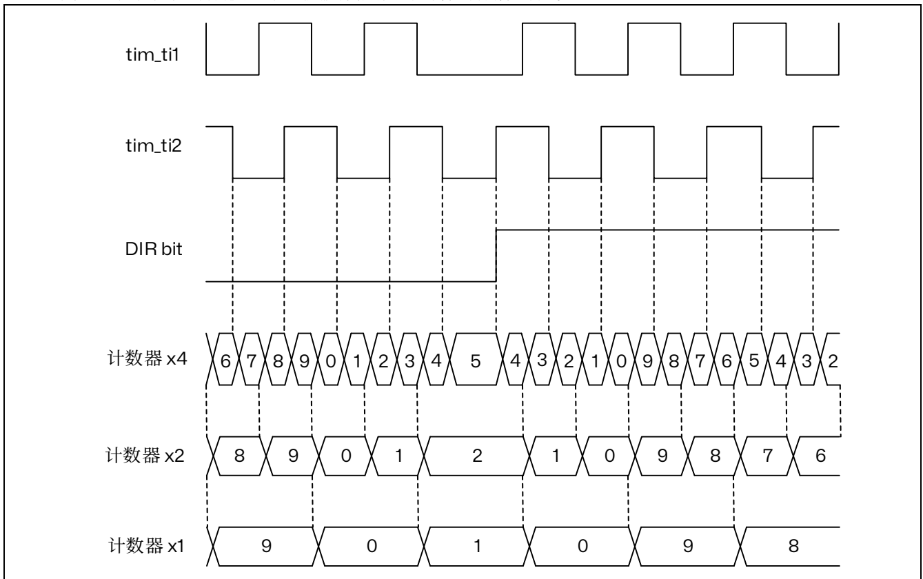
图 15.53 正交编码器的计数模式
