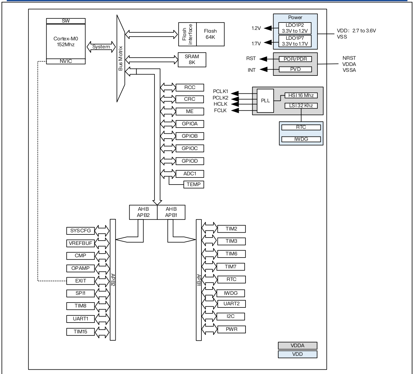
图 2.1 RX32H610 架构图
