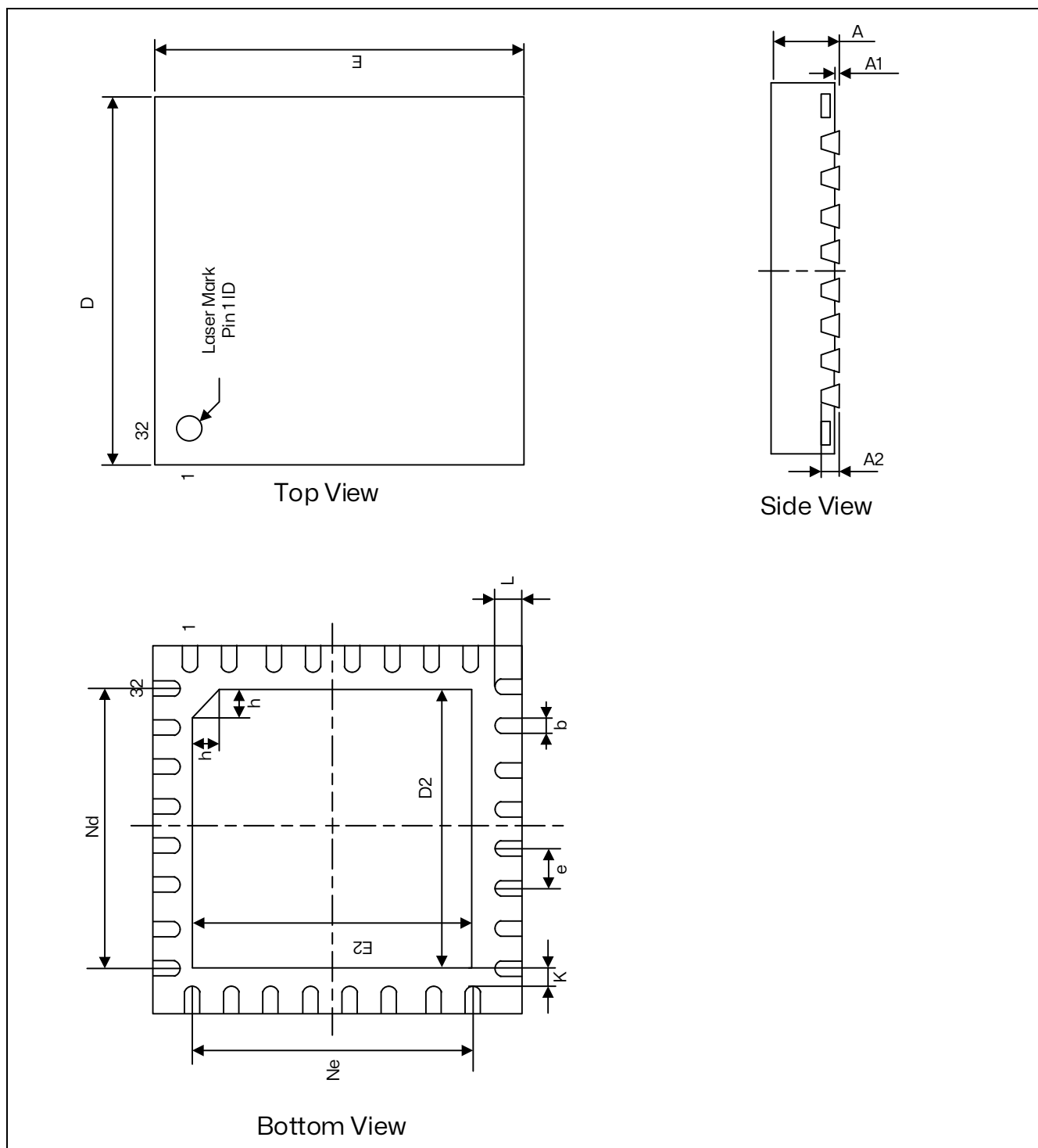
图 6.1 轮廓图
