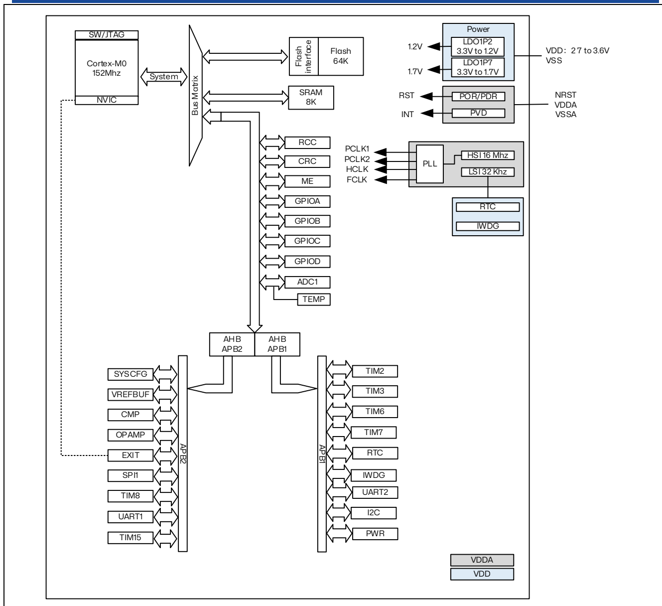
图 2.1 RX32H610 架构图
