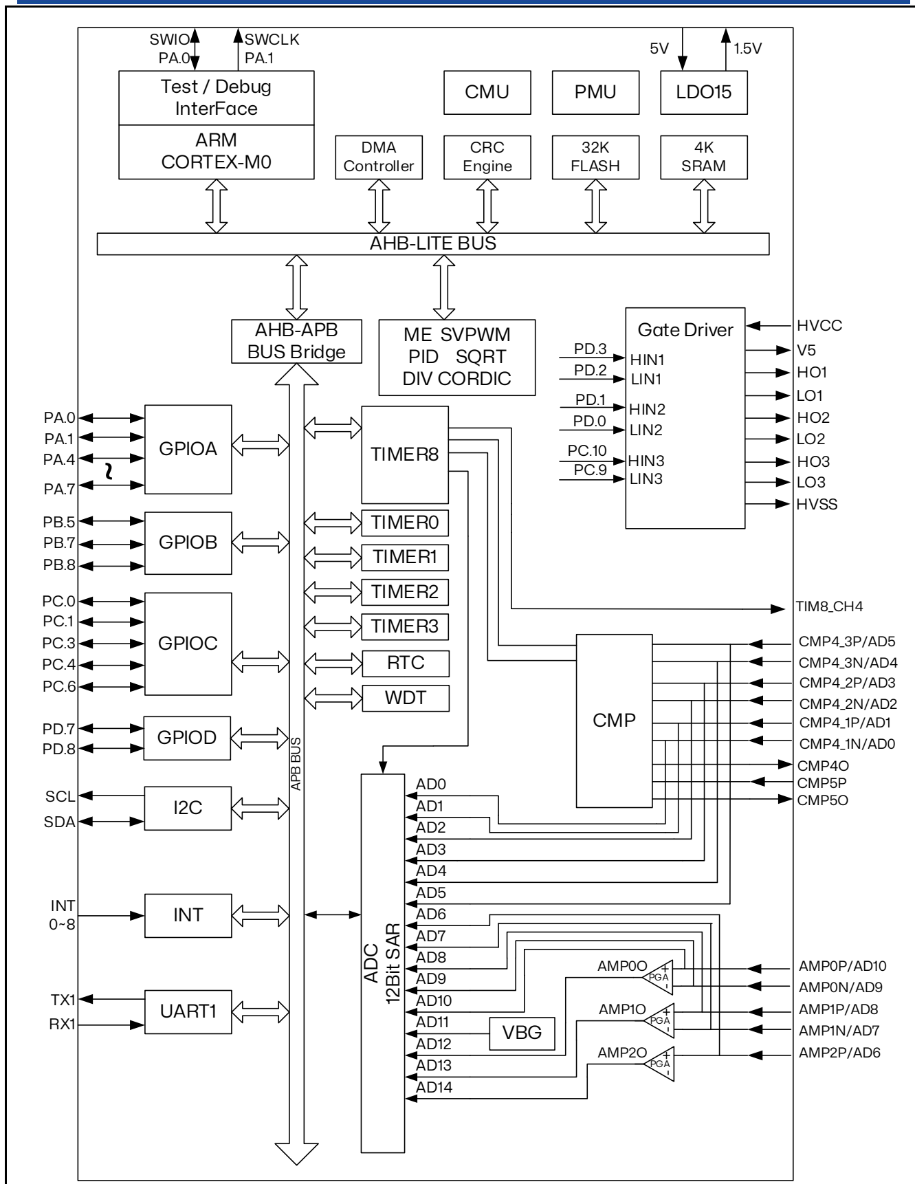
图 2.1 RX32SD22 架构图
