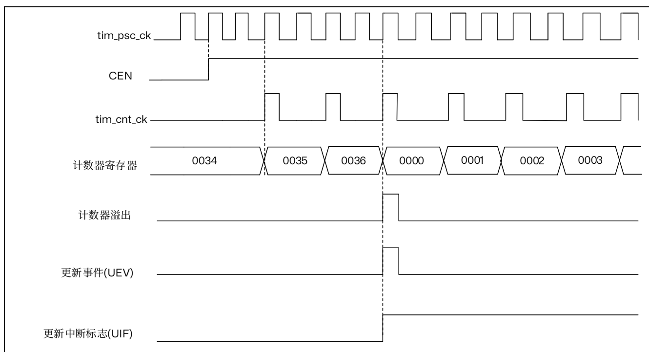
图 17.6 计数器时序图，内部时钟分频因子为 2
