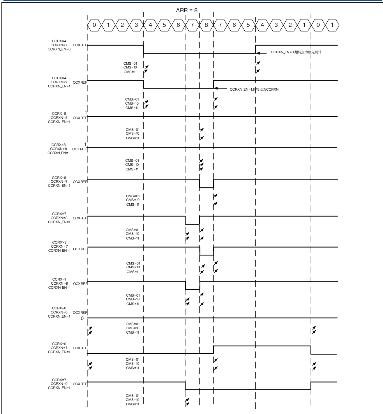
图 14.40 中央对齐的 PWM 波形 (ARR=8)
