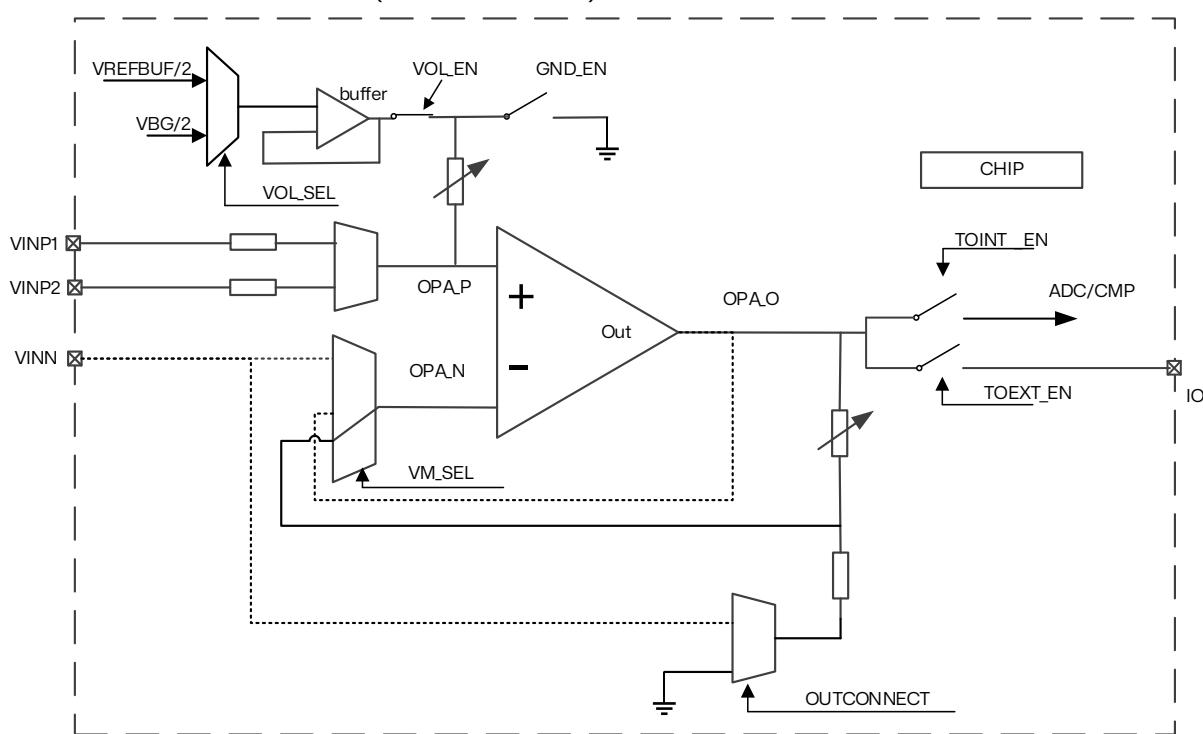
图 18.9 OPAMP3 PGA 模式 (P-偏置, N-GND)
