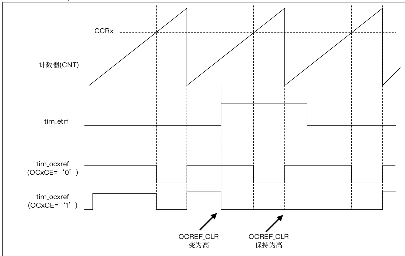
图 14.53 清除 TIM8 的 tim_ocxref
