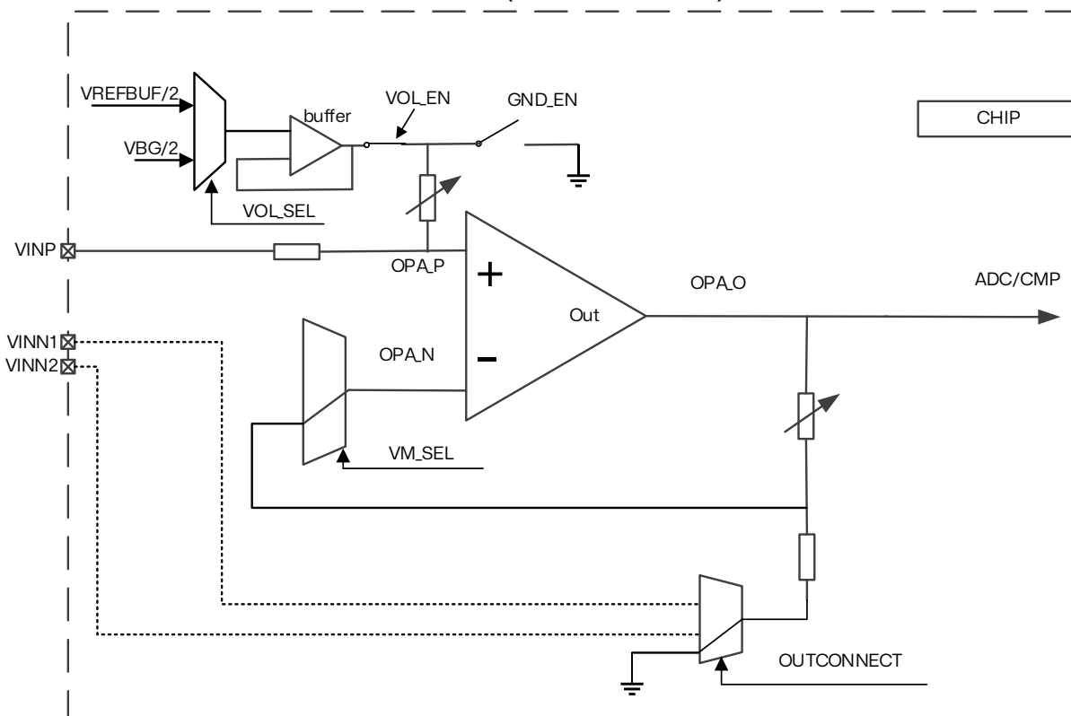
图 18.8 OPAMP1/OPAMP2 PGA 模式 (P-偏置, N-GND)
