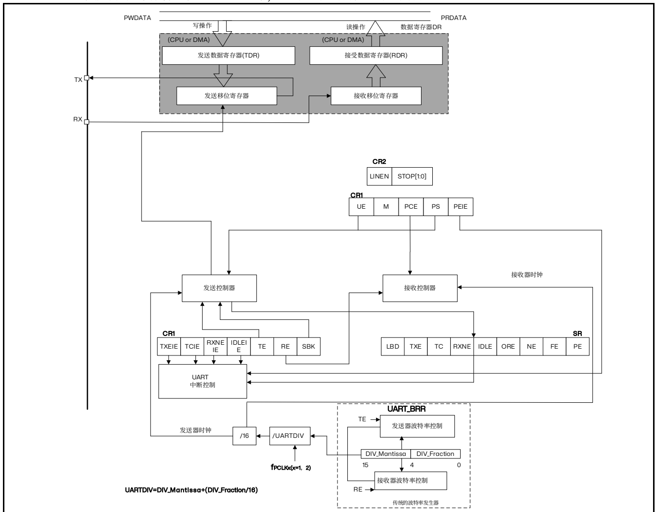
图 25.1 UART 框图
