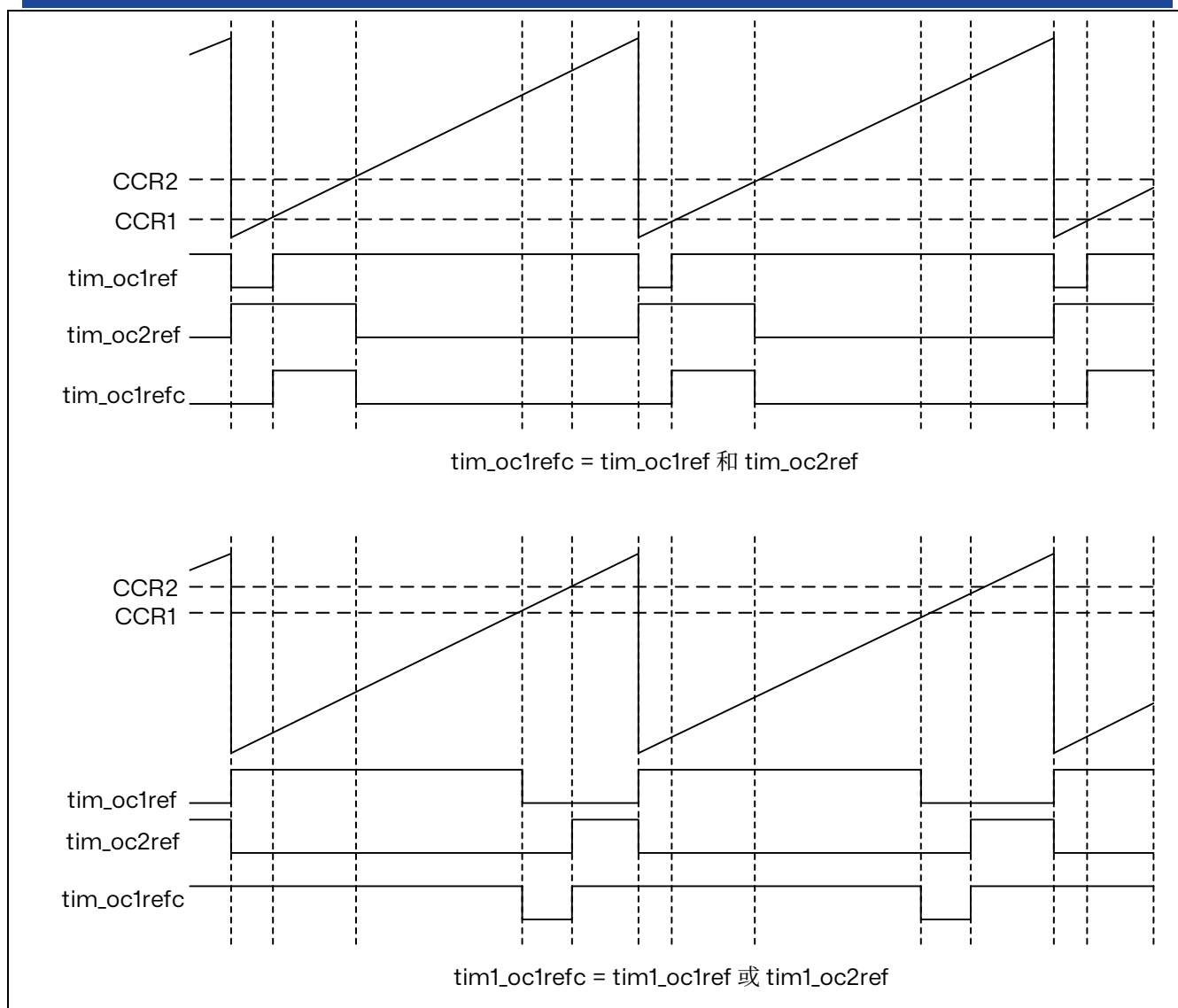
图 16.25 通道 1 和通道 2 的组合 PWM 模式
