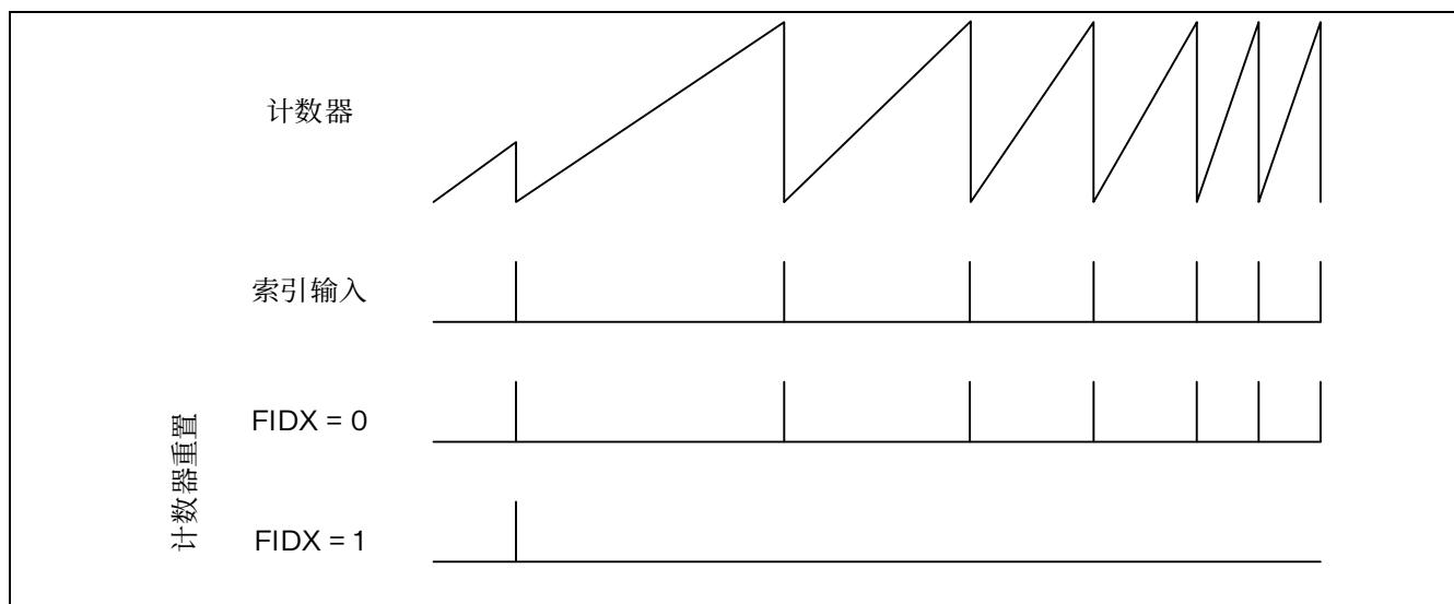
图 15.67 作为 FIDX 位设置的功能的计数器重置
