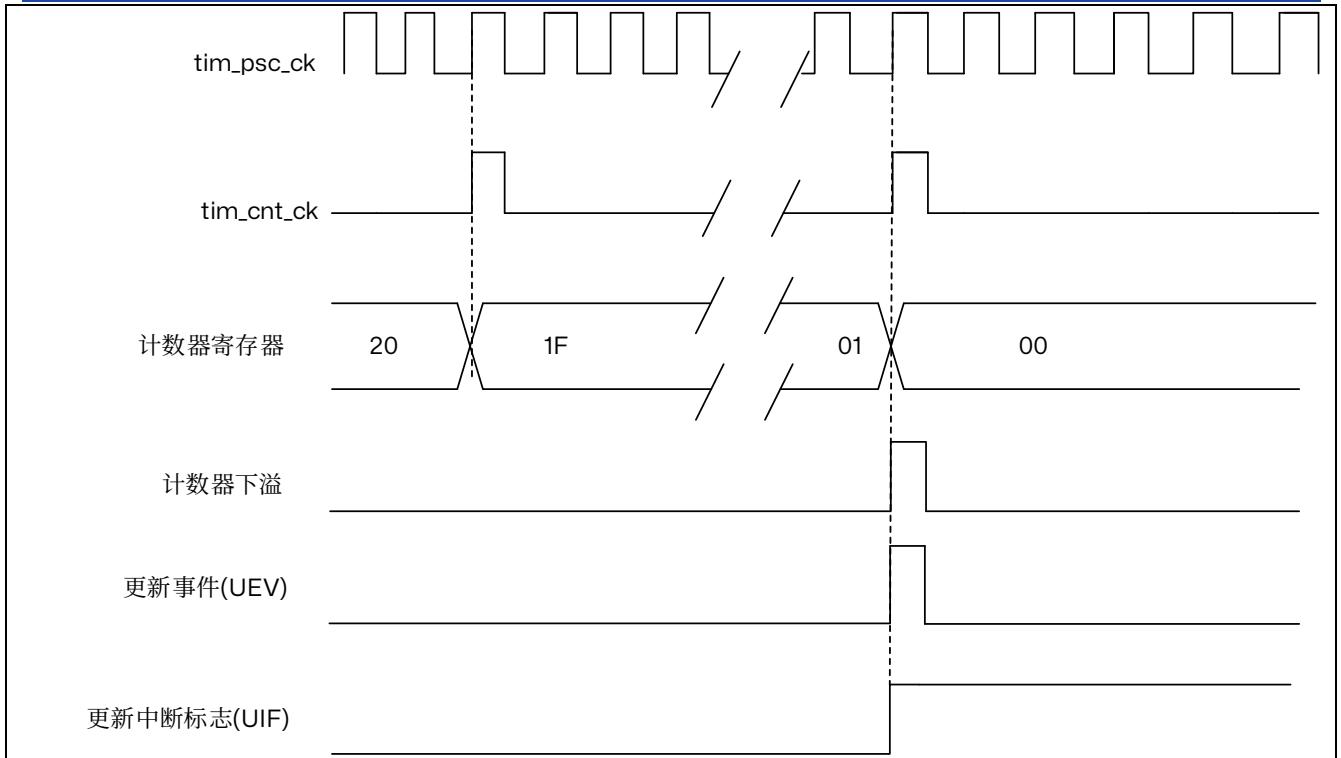
图 15.18 计数器时序图，内部时钟分频因子为 N
