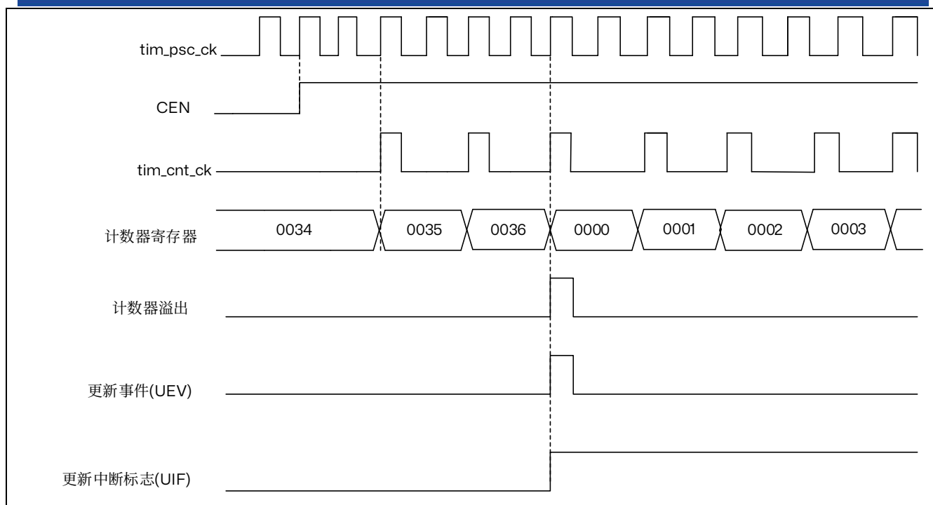
图 15.5 计数器时序图，内部时钟分频因子为 2
