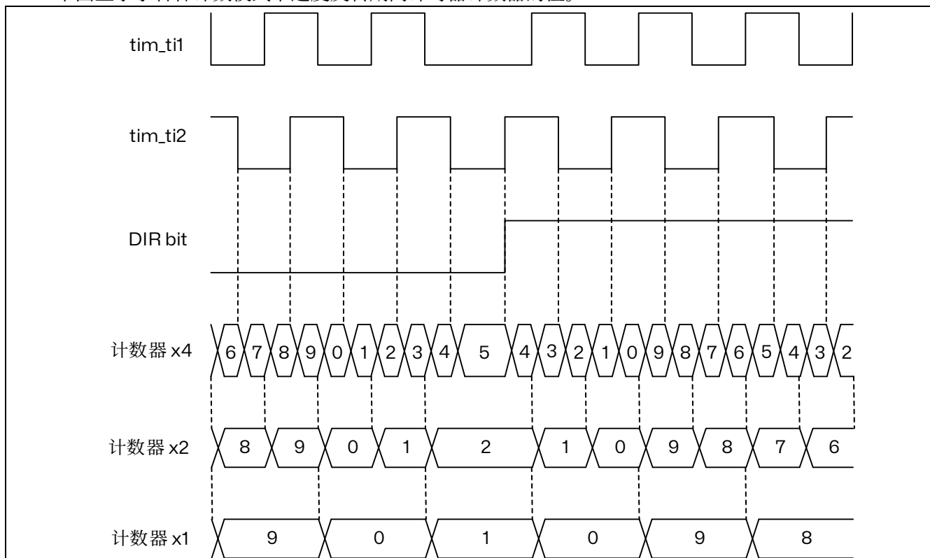
图 15.53 正交编码器的计数模式
