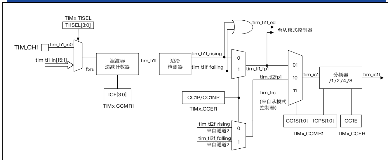
输出阶段生成一个中间波形作为基准：OCxRef（高电平有效）。链的末端决定最终输出信号的极性。 图 15.26 捕获/比较通道（如：通道 1 输入部分）
