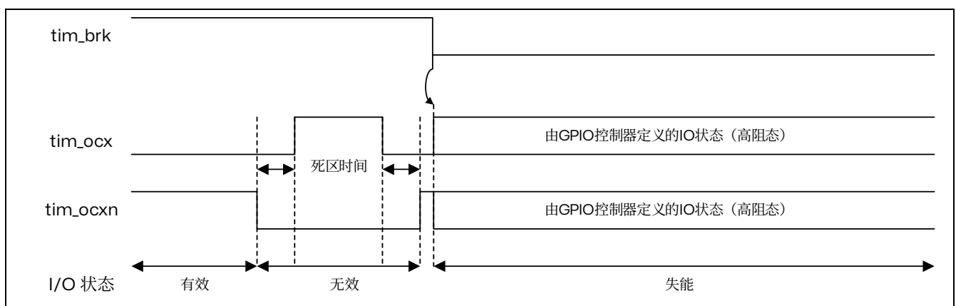
图 14.50 当 tim_brk 有效 (OSS1=0) 时 PWM 输出状态
