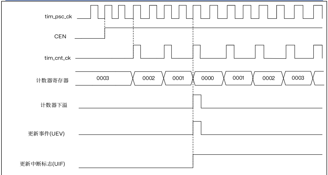
图 14.16 计数器时序图，内部时钟分频因子为 2
