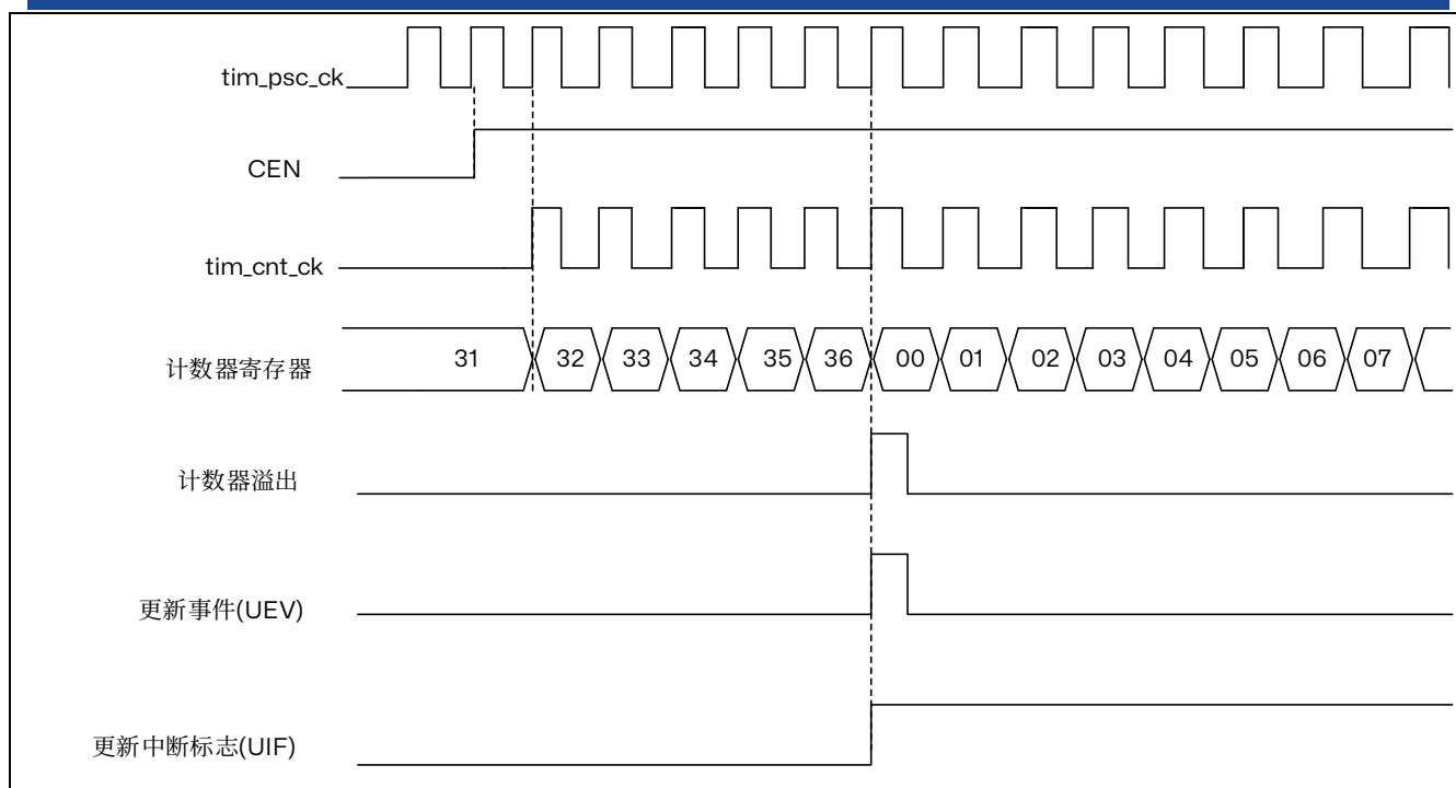
图 17.5 计数器时序图，内部时钟分频因子为 1
