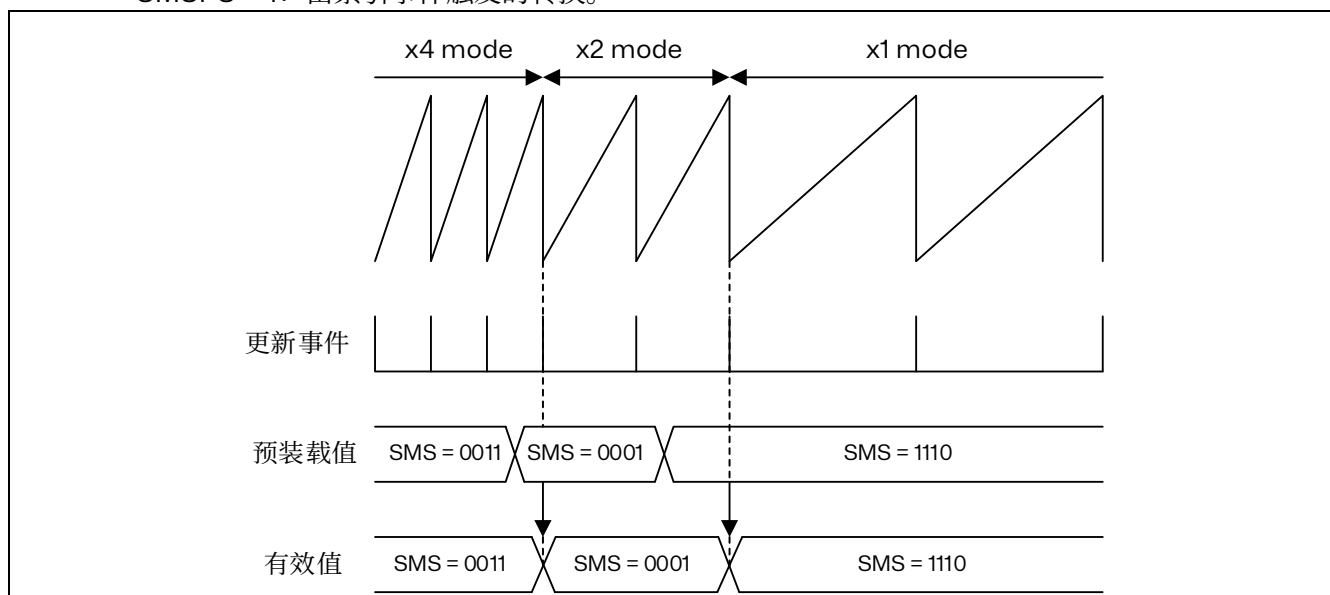
图 15.73 更新时带有预加载转移的编码器模式更改 (SMSPS = 0)
