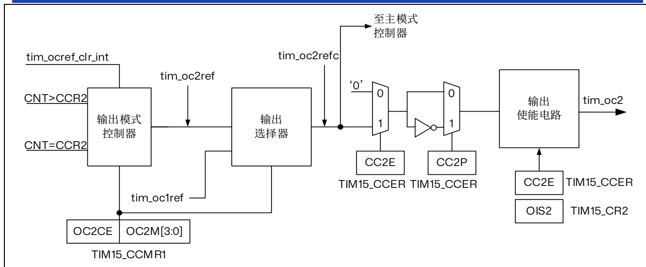
图 16.17 捕获比较通道的输出阶段（通道 2，通道 3 同上）
