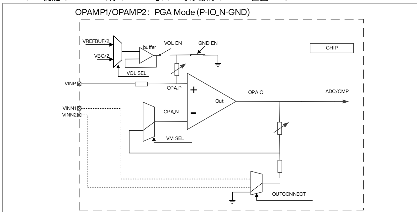
图 18.6 OPAMP1/OPAMP2 PGA 模式 (P-IO, N-GND)
