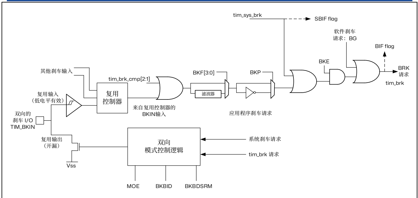
图 14.51 输出重定向（未表示 tim_brk2 请求）
