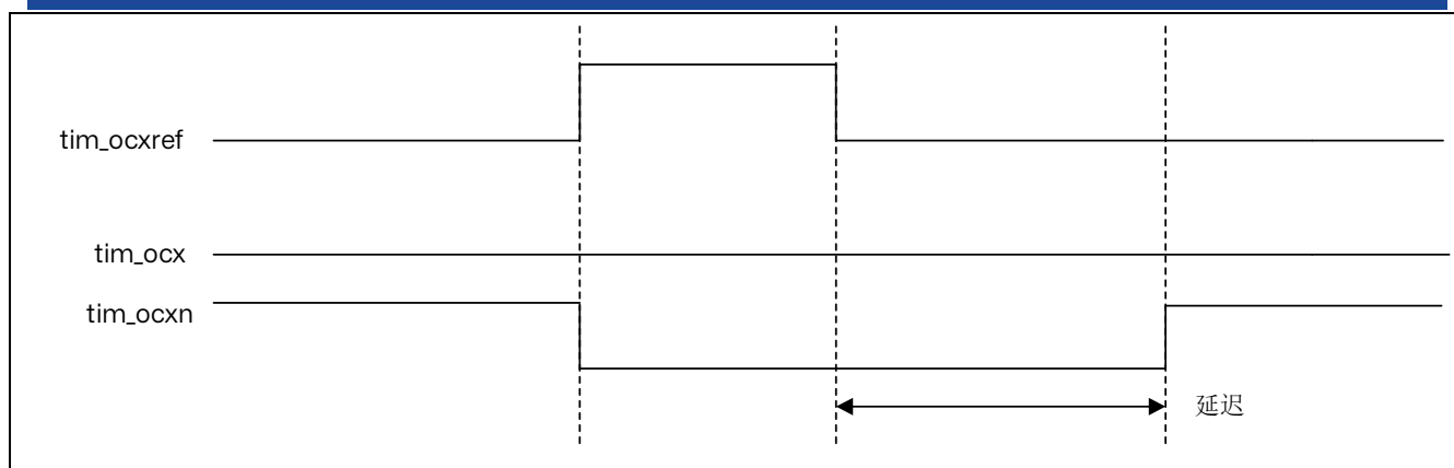
图 16.29 死区波形延迟大于正脉冲
