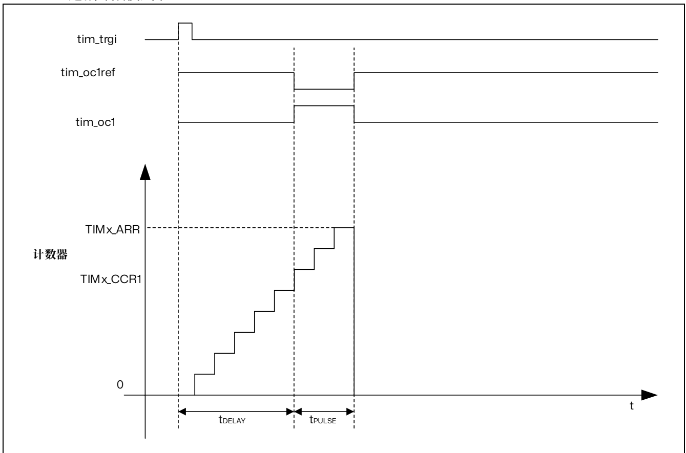
图 14.55 单脉冲模式的例子
