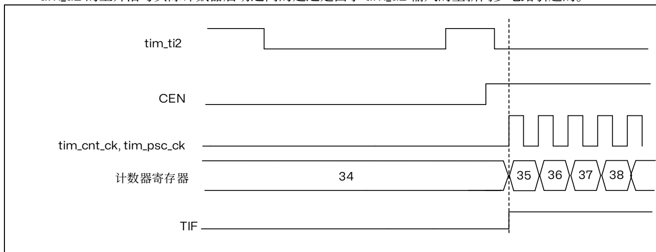
图 15.76 触发器模式下的控制电路
