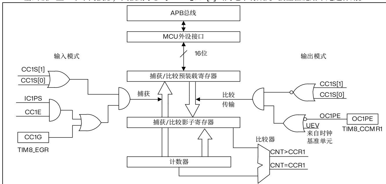
图 14.26 捕获/比较通道 1 的主电路
