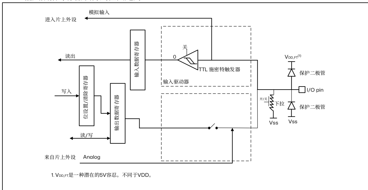
图 8.5 模拟引脚框图
