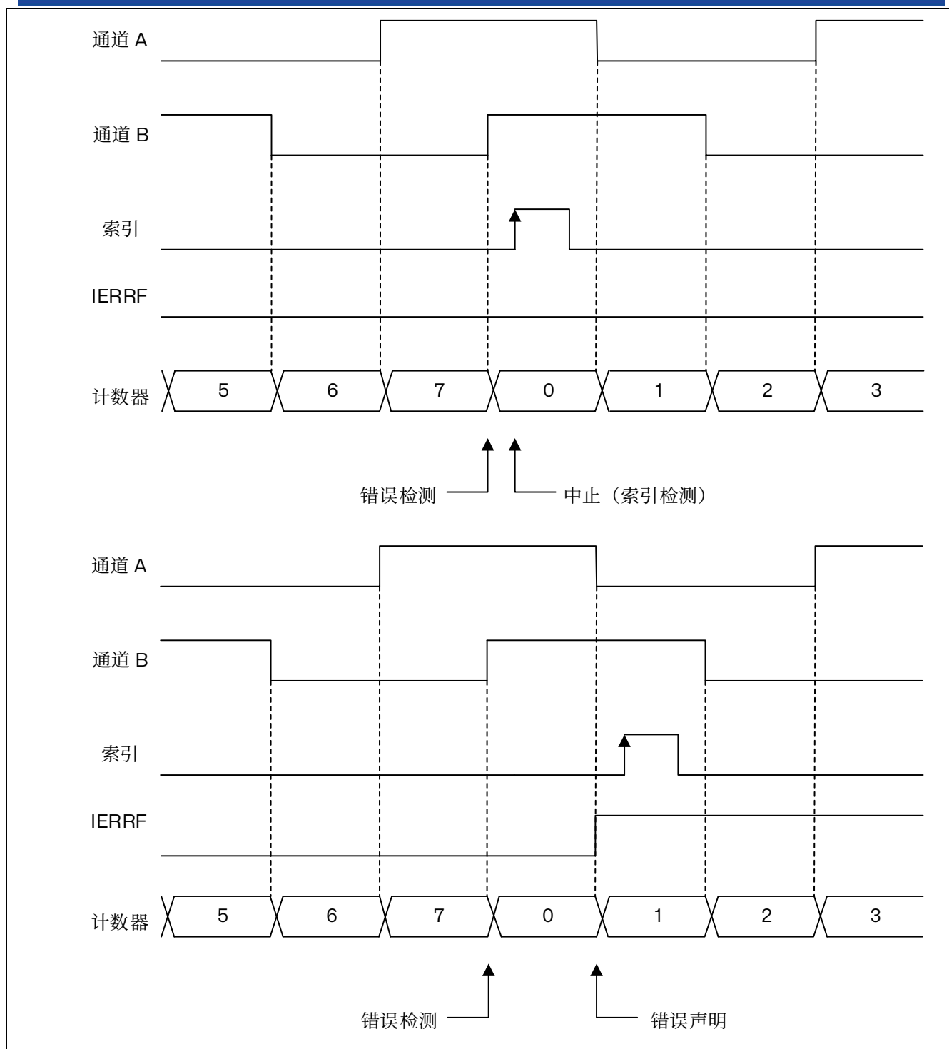
图 15.71 递增计数编码器错误检测
