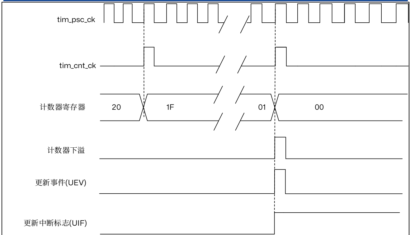
图 14.18 计数器时序图，内部时钟分频因子为 N
