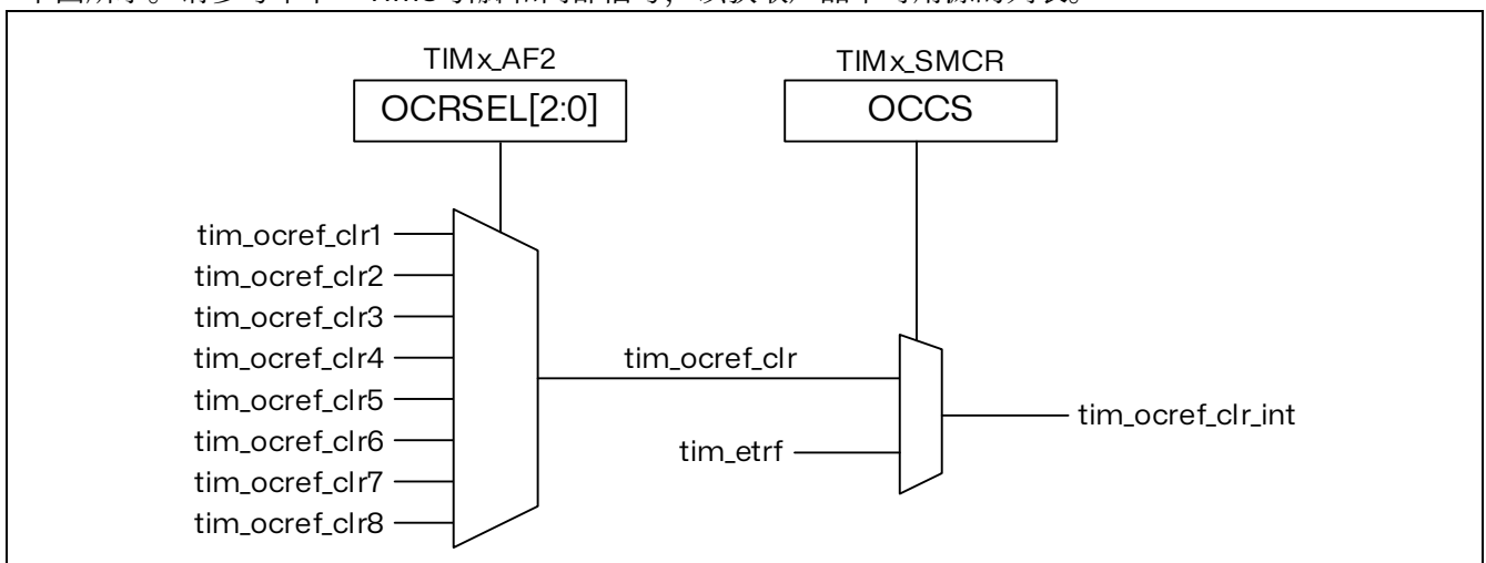
图 14.52 tim_ocref_clr 输入选择复用器
