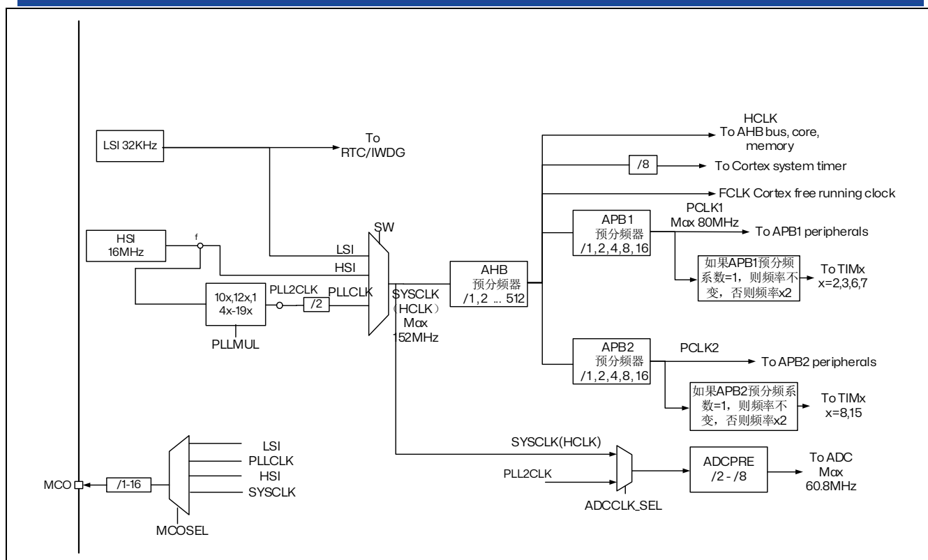
图 7.2 时钟树
