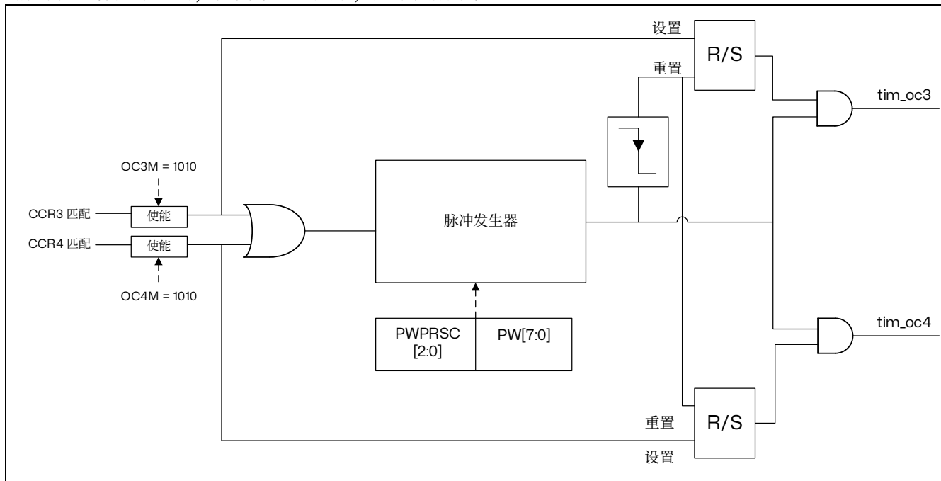
图 14.57 脉冲发生器电路
