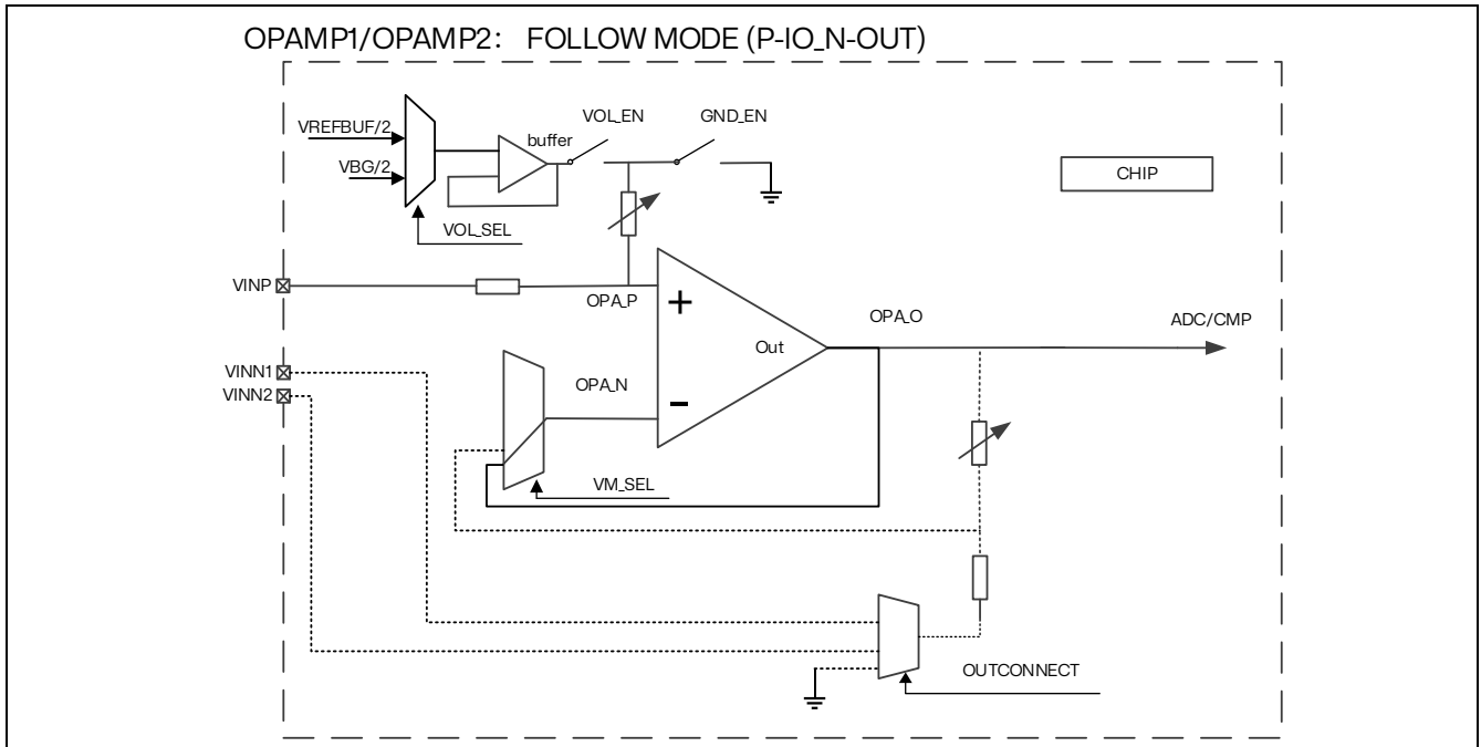
图 18.2 OPAMP1/OPAMP2 电压跟随器模式
