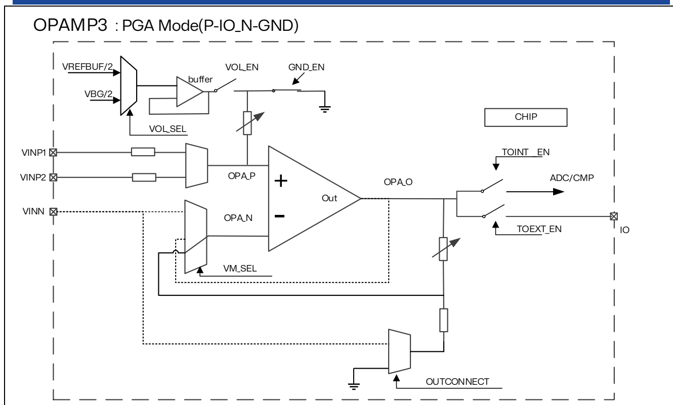
图 18.7 OPAMP3 PGA 模式 (P-IO, N-GND)
