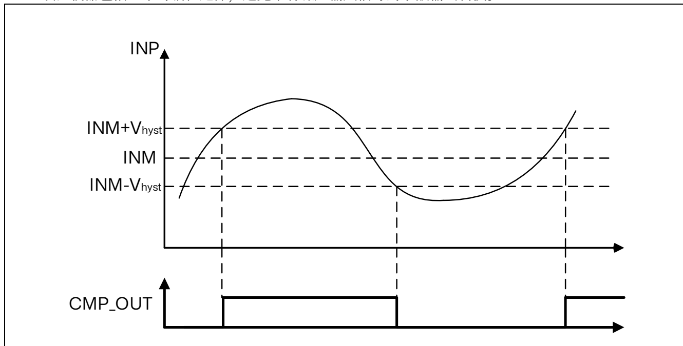
图 19.2 比较器迟滞
