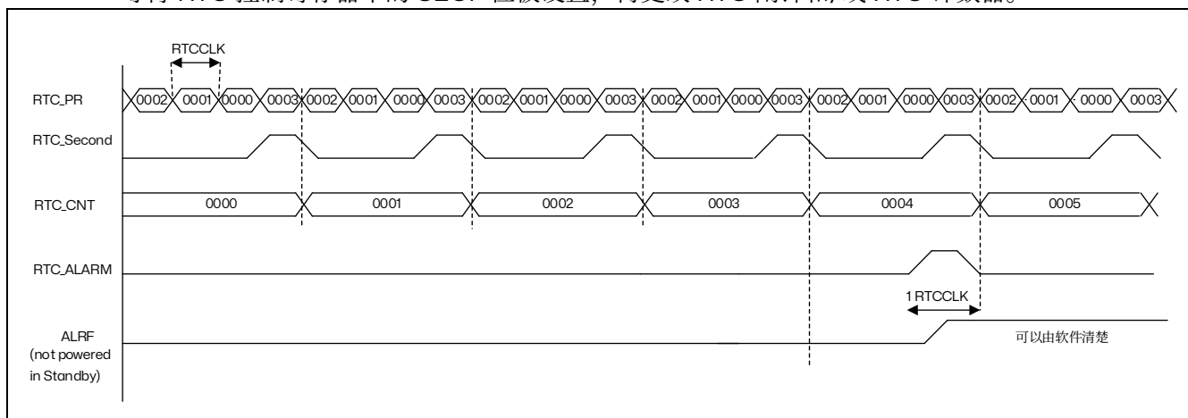
图 21.2 RTC 秒和闹钟波形图示例，PR=0003，ALARM=00004
