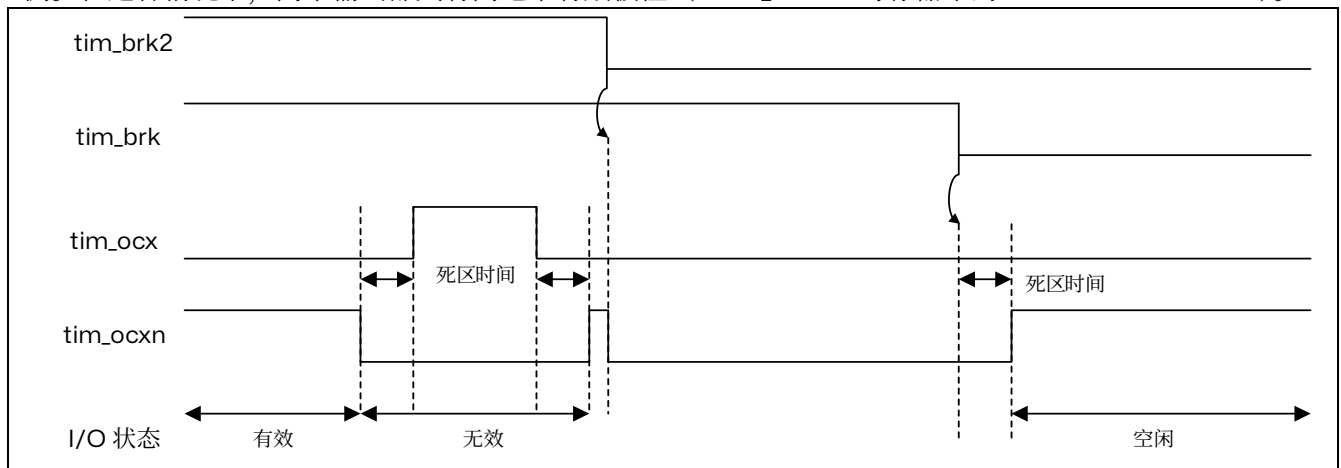
图 14.49 当 tim_brk 和 tim_brk2 有效 (OSS1=1) 时 PWM 输出状态
