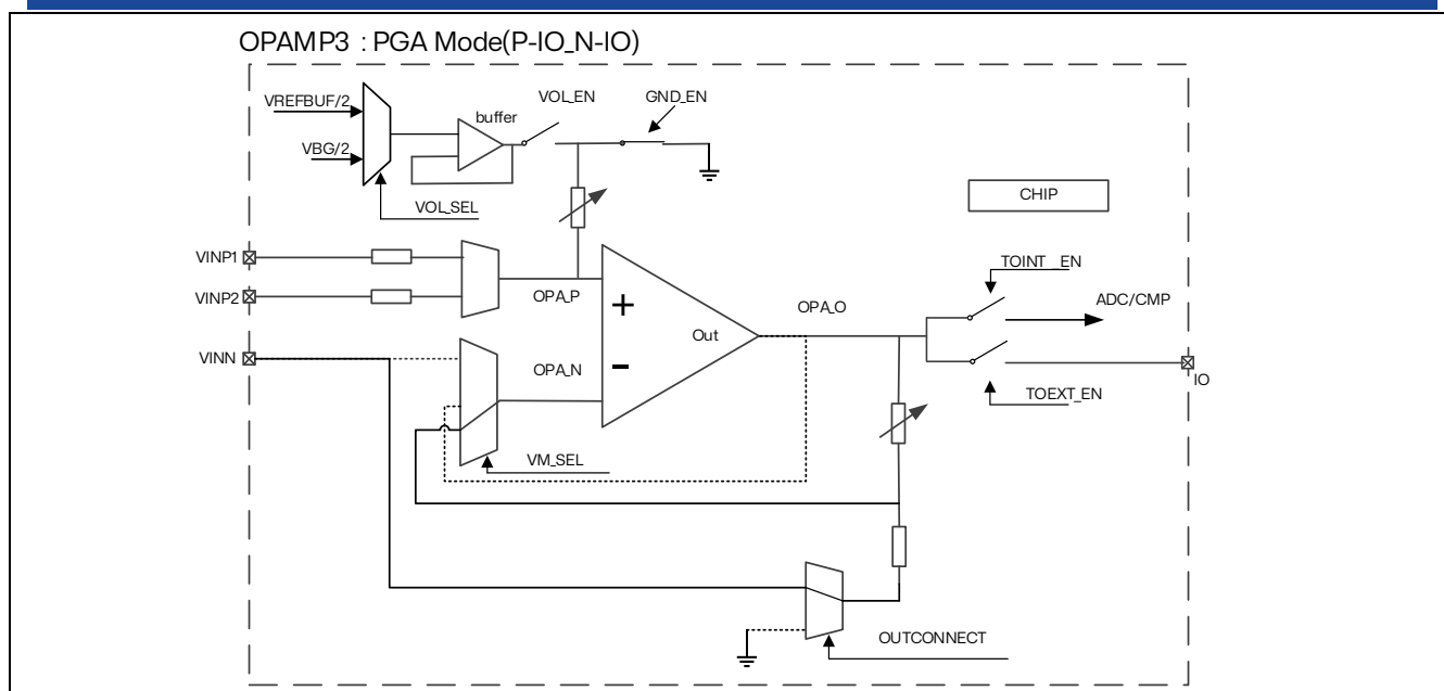
图 18.5 OPAMP3 PGA 模式 (P-IO, N-IO)
