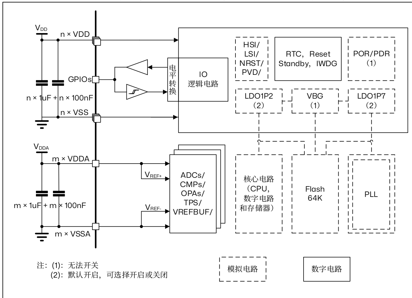
图 6.1 电源框图
