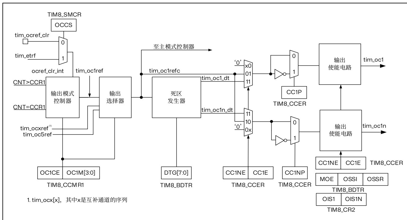
图 14.27 捕获/比较通道的输出阶段（通道 1，通道 2、3 和 4 同上）
