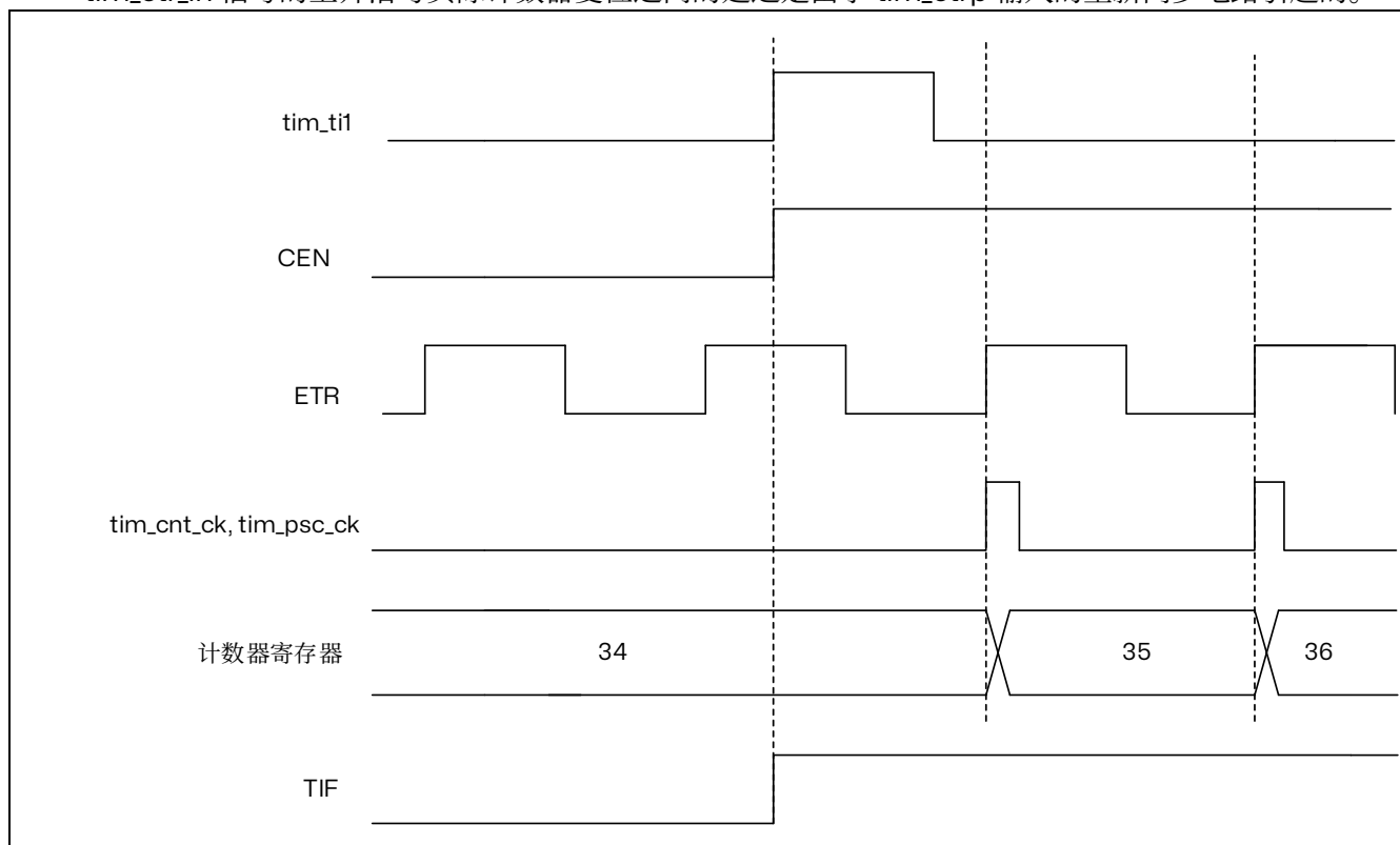
图 15.77 外部时钟模式 2+触发模式下的控制电路
