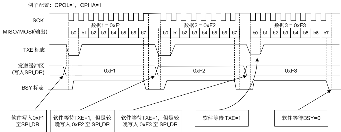
图 23.10 非连续传输发送 (BIDIMODE=0 并且 RXONLY=0) 时, TXE/BSY 变化示意图
