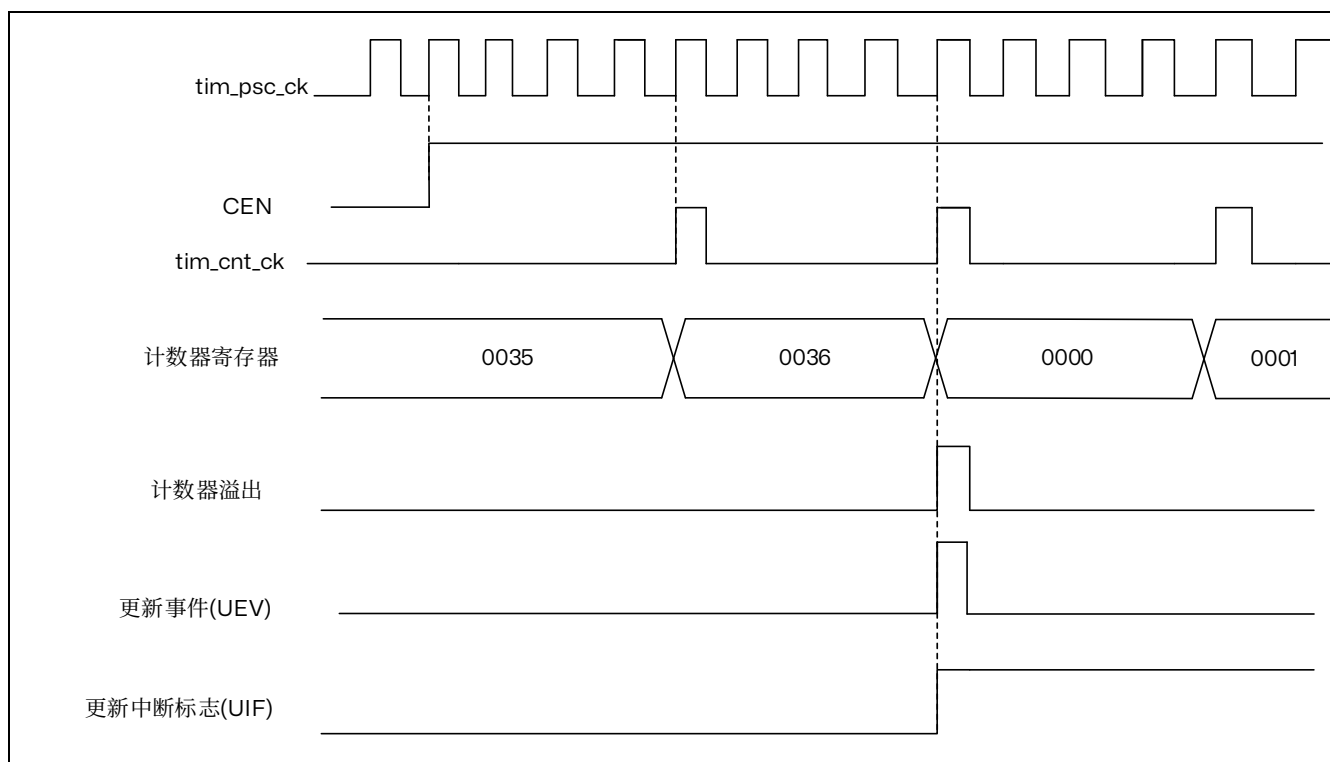
图 14.6 计数器时序图，内部时钟分频因子为 4
