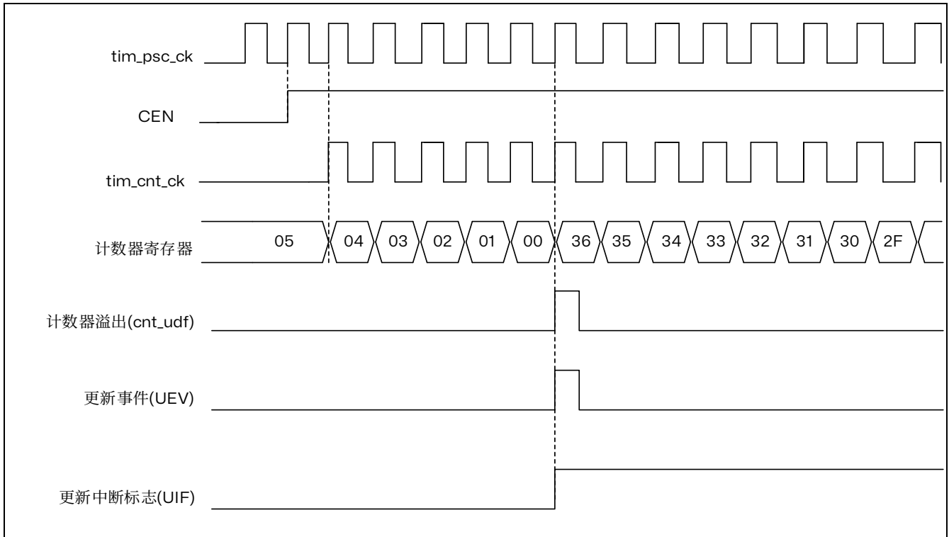
图 14.10 计数器时序图，内部时钟分频因子为 1
