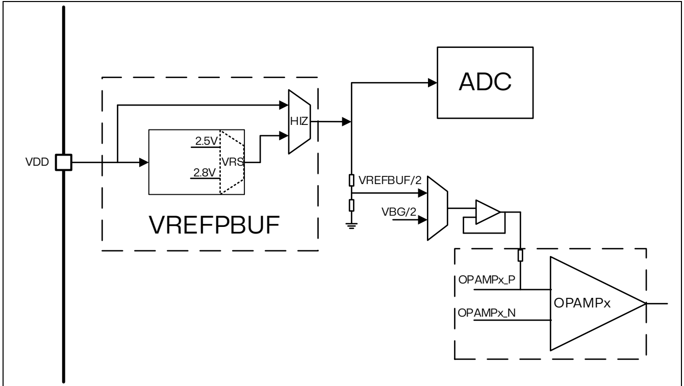
图 12.1 VREFBUF 框图
