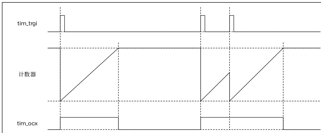
图 14.56 可重触发单脉冲模式
