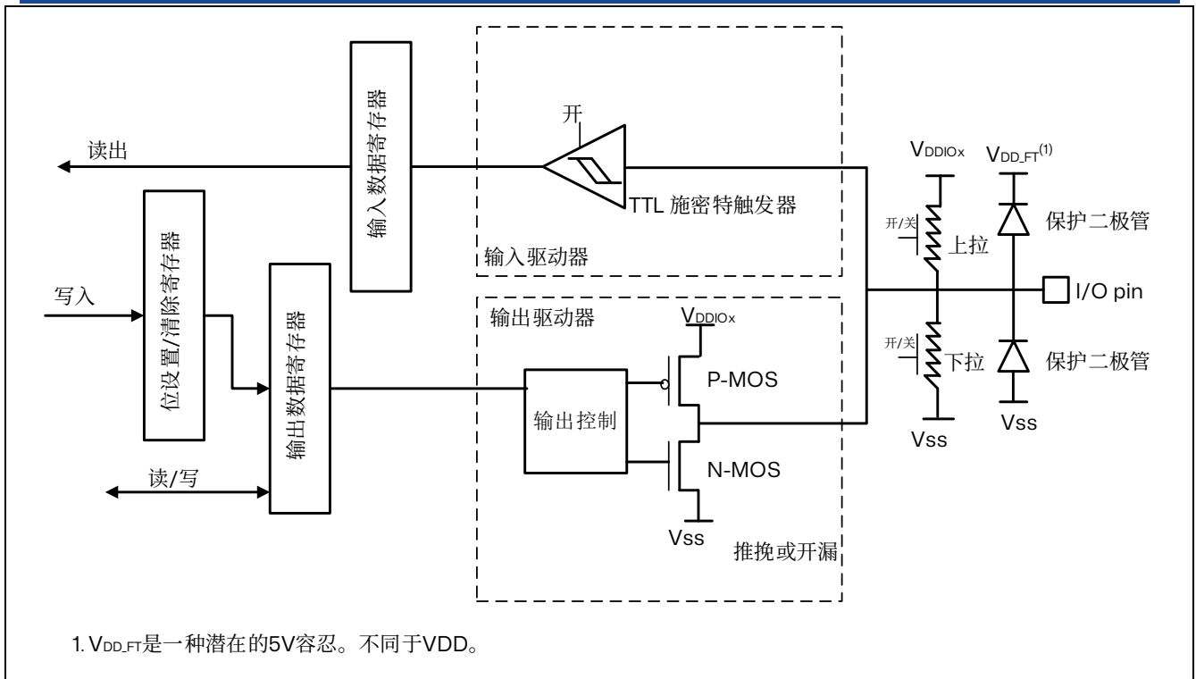
图 8.3 输出框图
