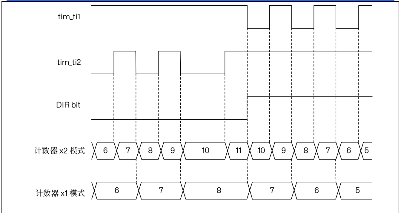
图 15.55 方向时钟编码器模式 (CC1P=CC2P=0)
