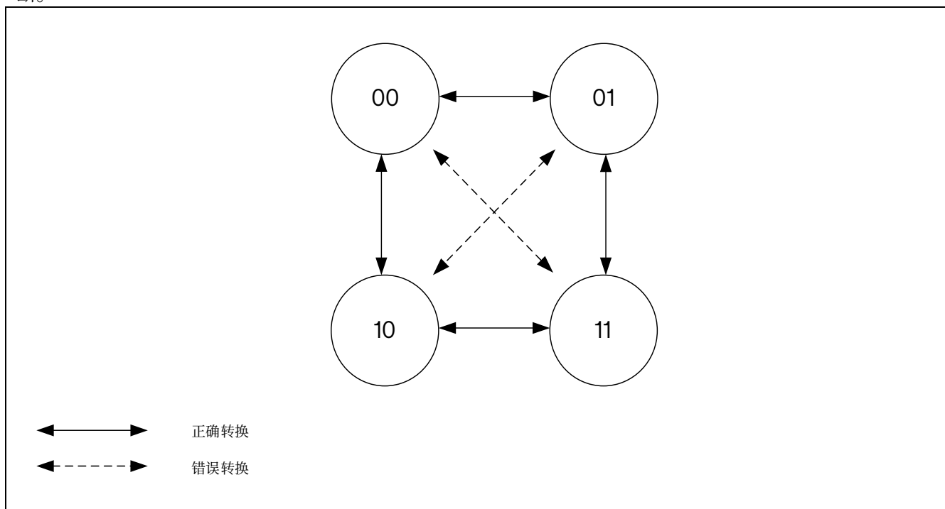
图 15.70 正交编码信号的状态图
