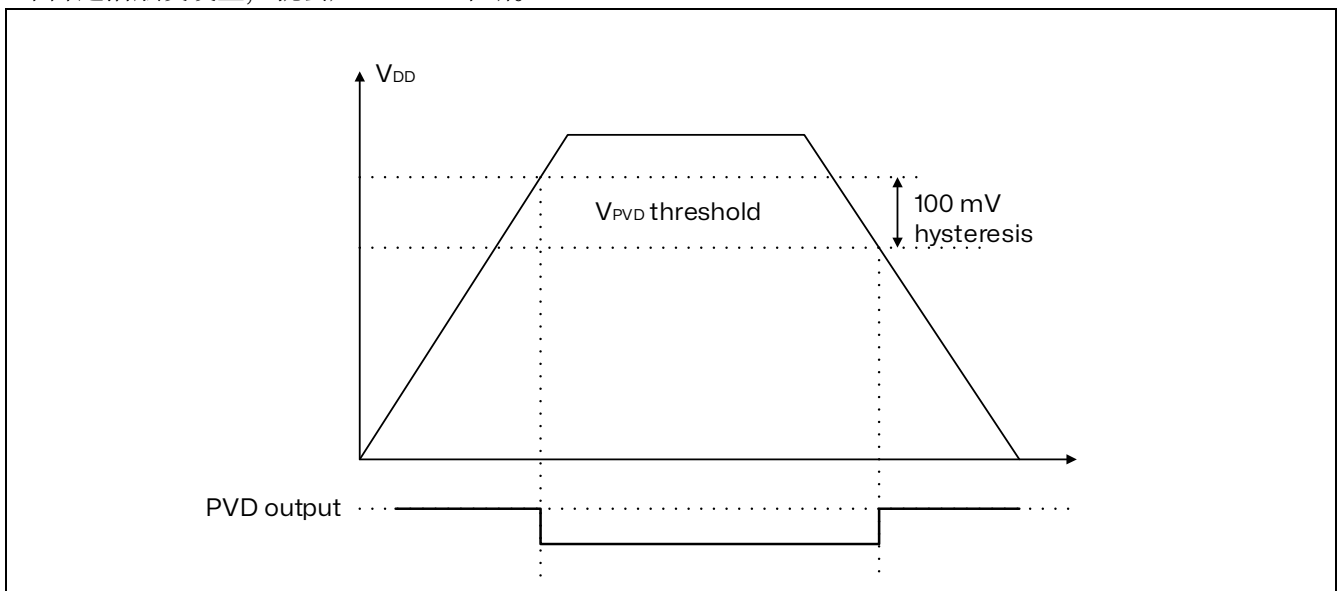
图 6.3 PVD 门限
