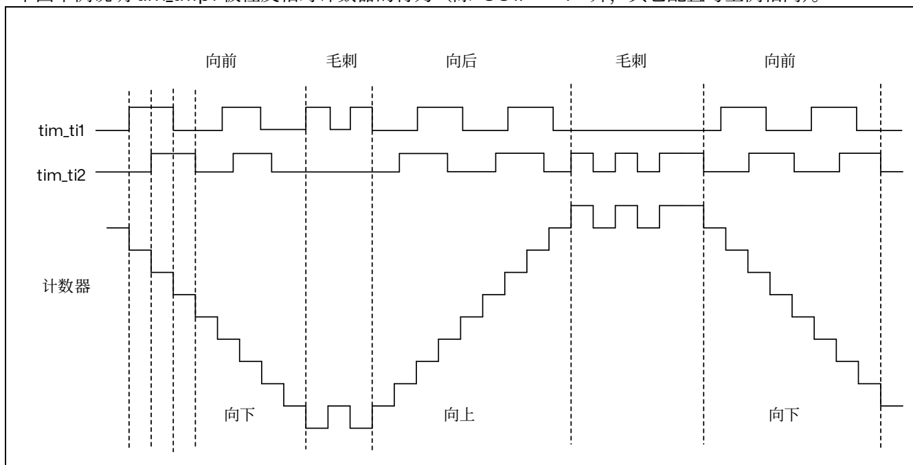
图 15.52 tim_ti1fp1 极性反相时的编码器接口模式示例
