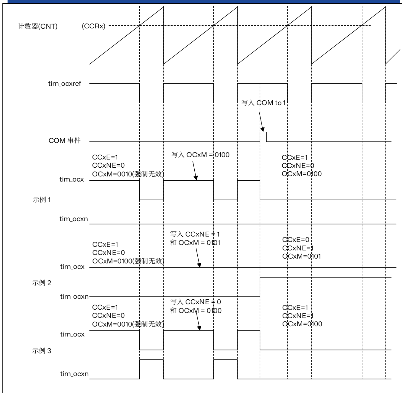
图 14.54 COM 事件生成 6 步 PWM 的示例 (OSSR=1)
