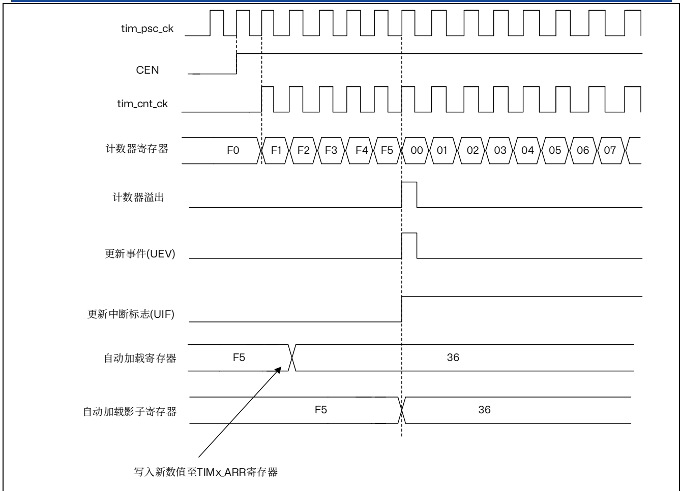
图 17.10 计数器时序图，当 ARPE=1 时的更新事件（预装入了 TIMx_ARR）
