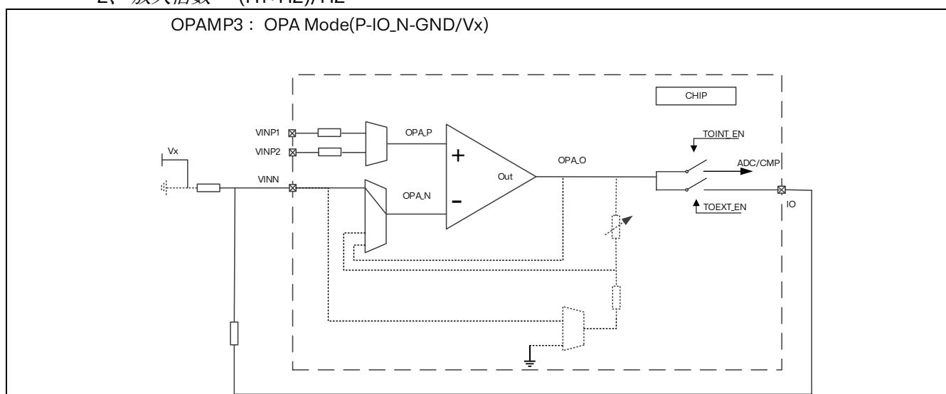
图 18.1 OPAMP3 独立模式
