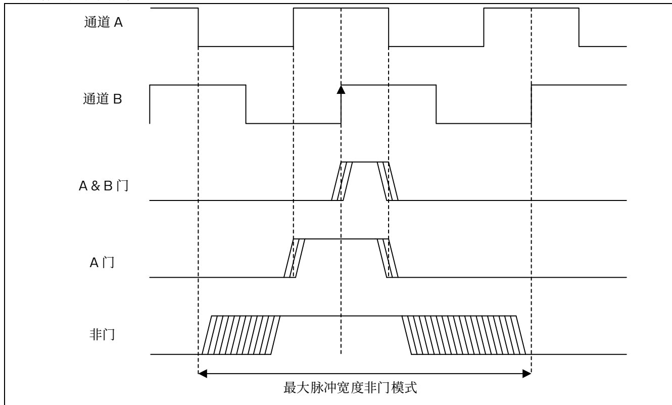
图 15.58 抖动的索引信号
