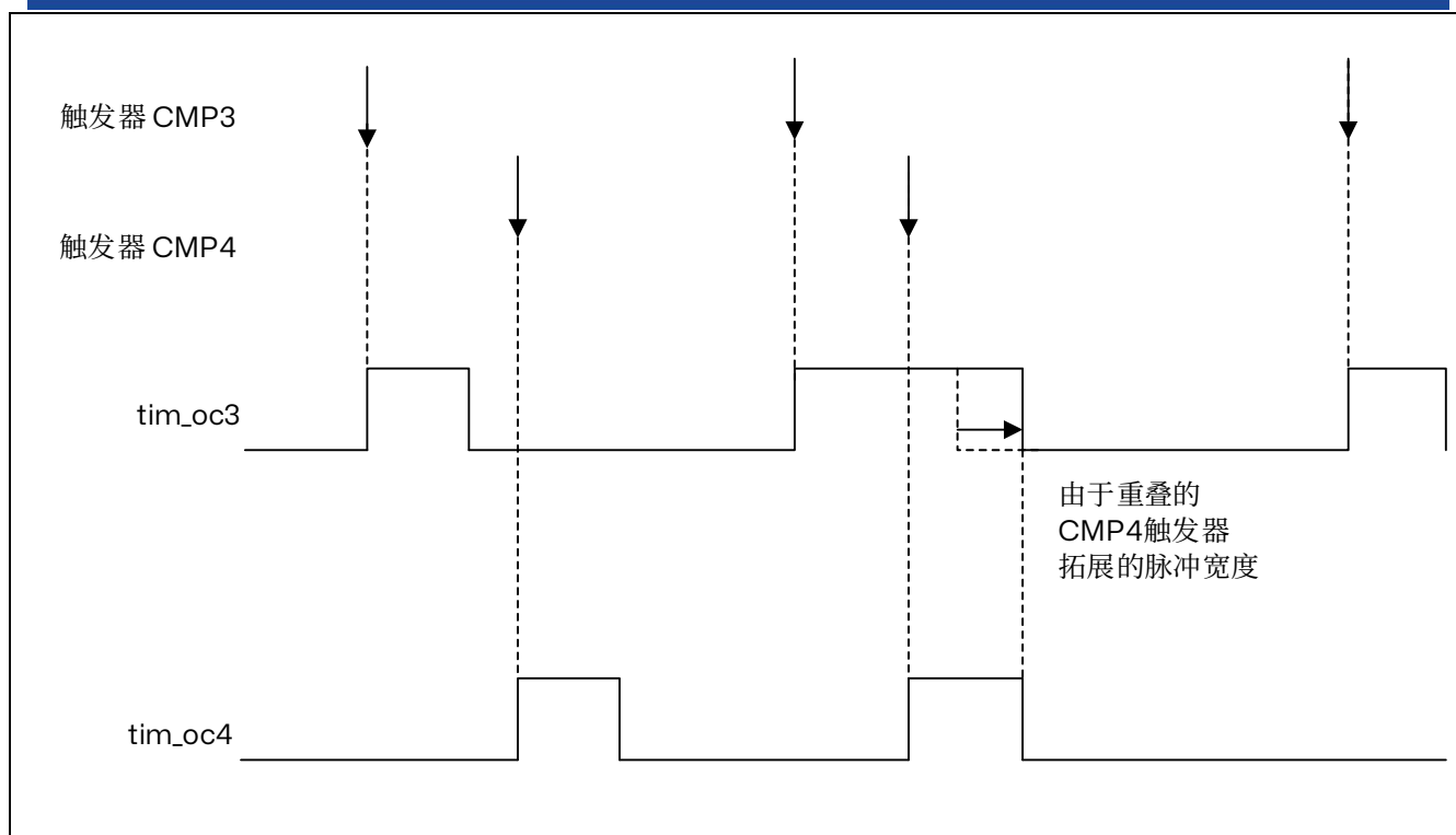
图 14.59 在同时触发的情况下延长脉冲宽度
