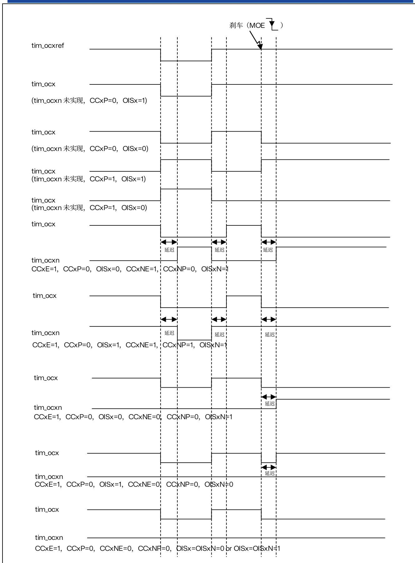
图 16.31 tim_brk 在发生刹车事件时的各种输出行为 (OSSI=1)
