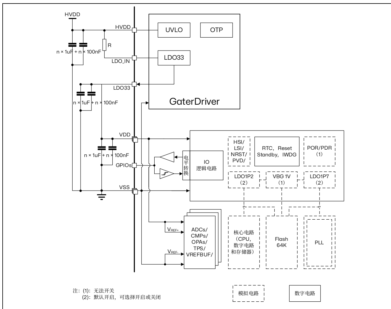
图 5.3 供电方案
