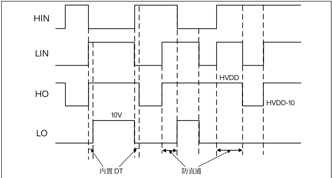
图 5.8 输入输出时序波形
