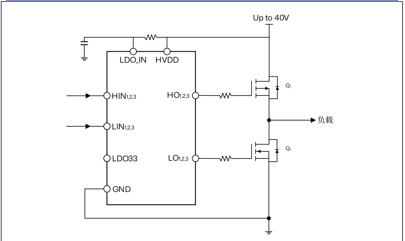
图 5.10 典型应用电路
