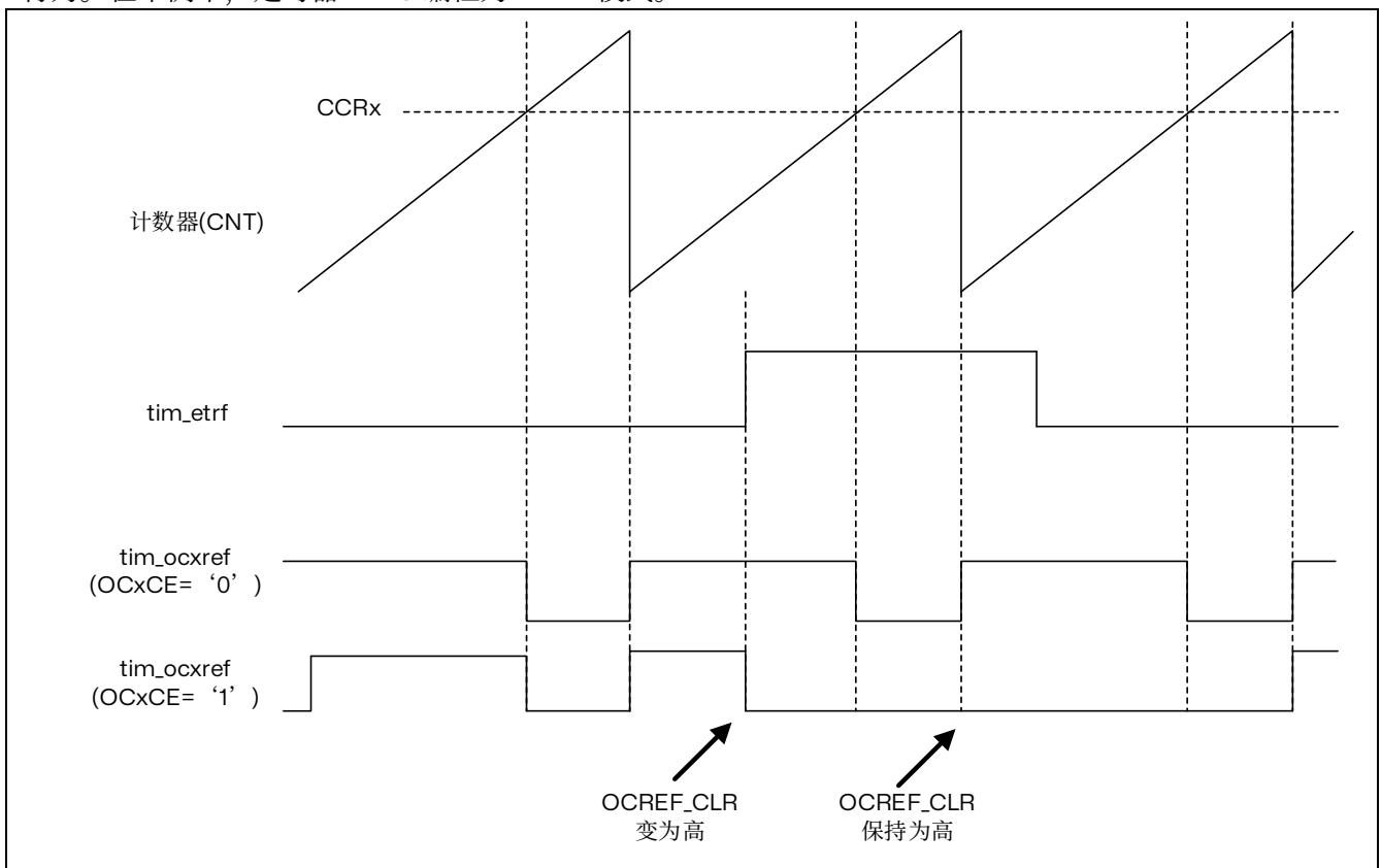
图 14.52 清除 TIM8 的 tim_ocref
