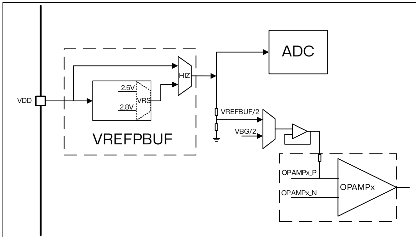
图 12.1 VREFBUF 框图
