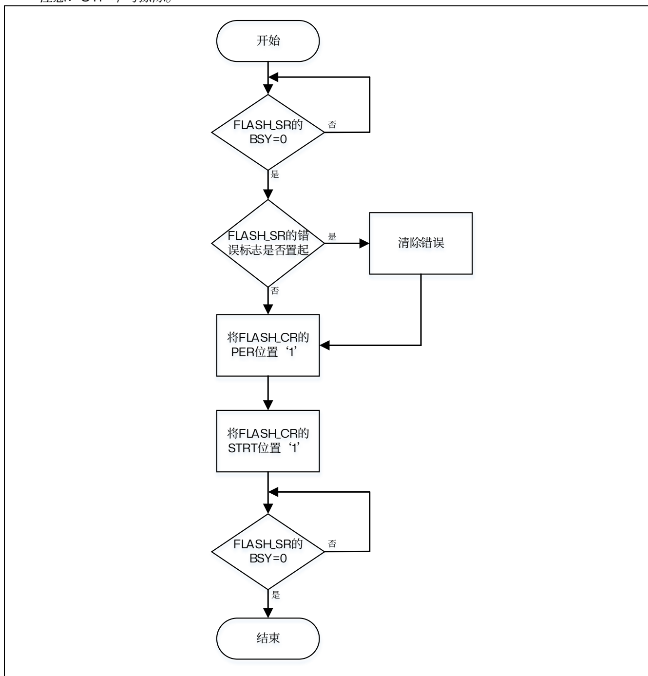
图 4.2 全擦流程
