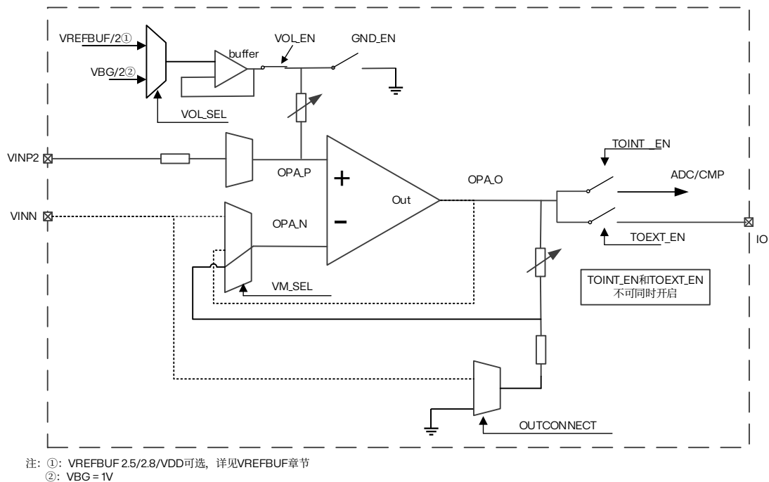
图 18.9 OPAMP3 PGA 模式 (P-偏置, N-GND)
