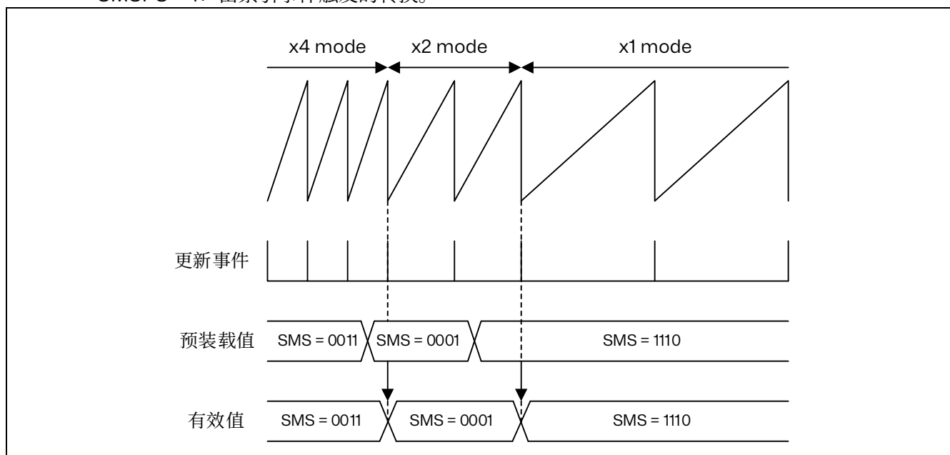
图 15.74 更新时带有预加载转移的编码器模式更改 (SMSPS = 0)
