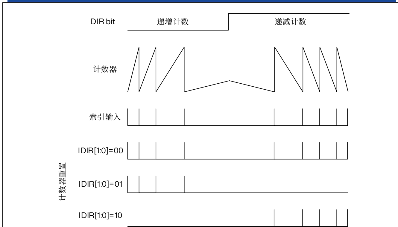
图 15.67 定向索引灵敏度
