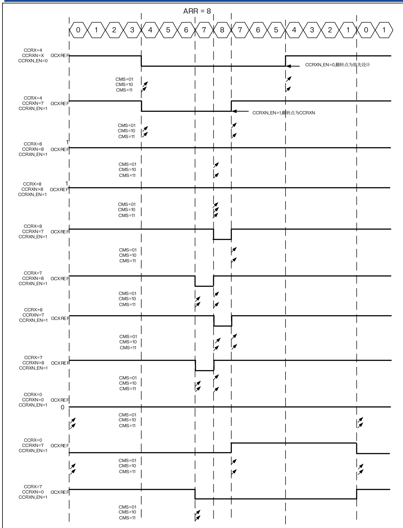
图 15.43 中央对齐的 PWM 波形 (ARR=8)
