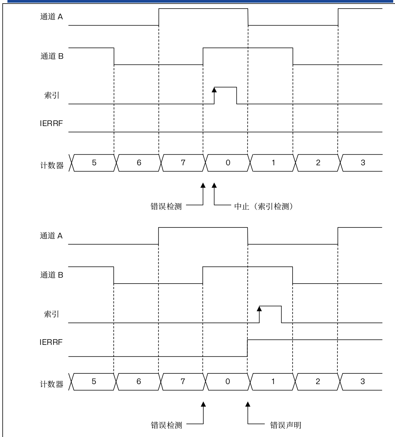
图 15.72 递增计数编码器错误检测
