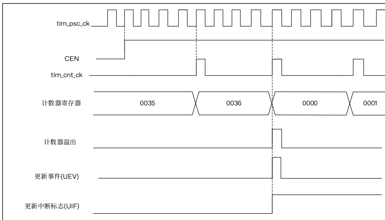
图 15.7 计数器时序图，内部时钟分频因子为 4
