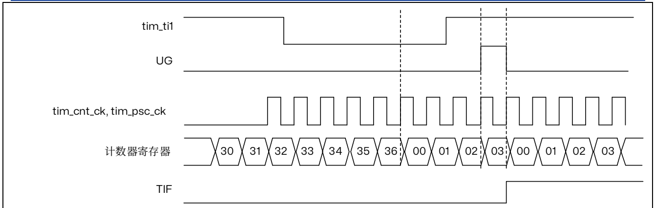
图 15.75 复位模式下的控制电路
