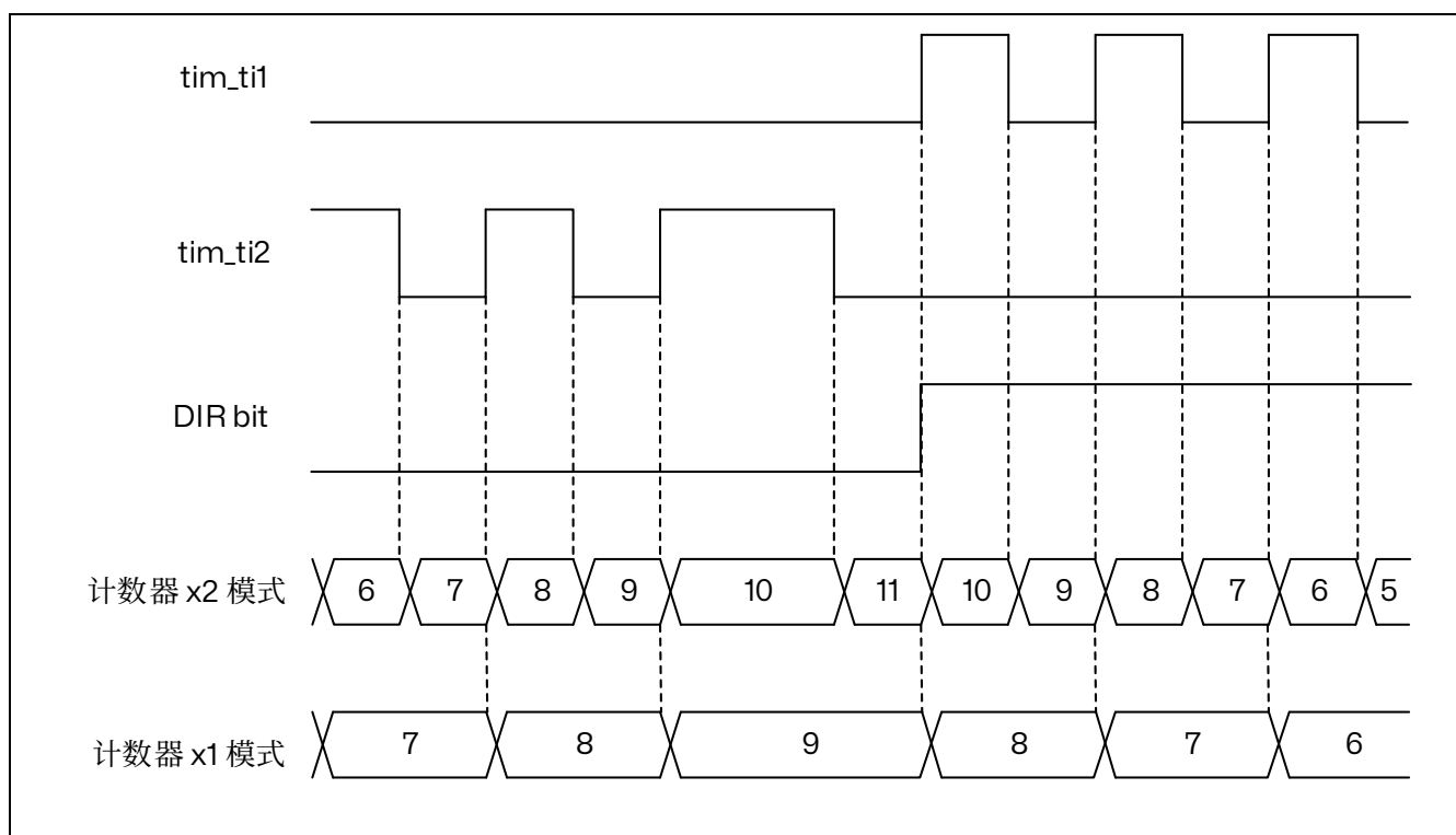
图 15.57 方向时钟编码器模式 ( CC1P=CC2P=1 )
