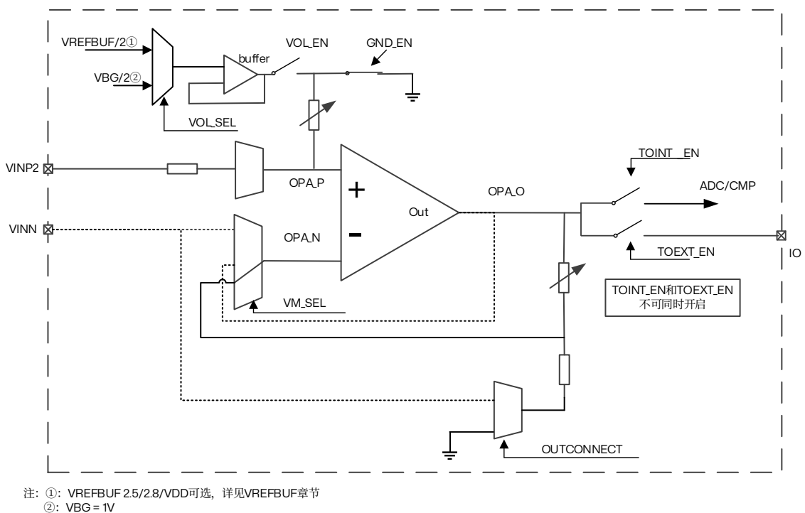
图 18.7 OPAMP3 PGA 模式 (P-IO, N-GND)
