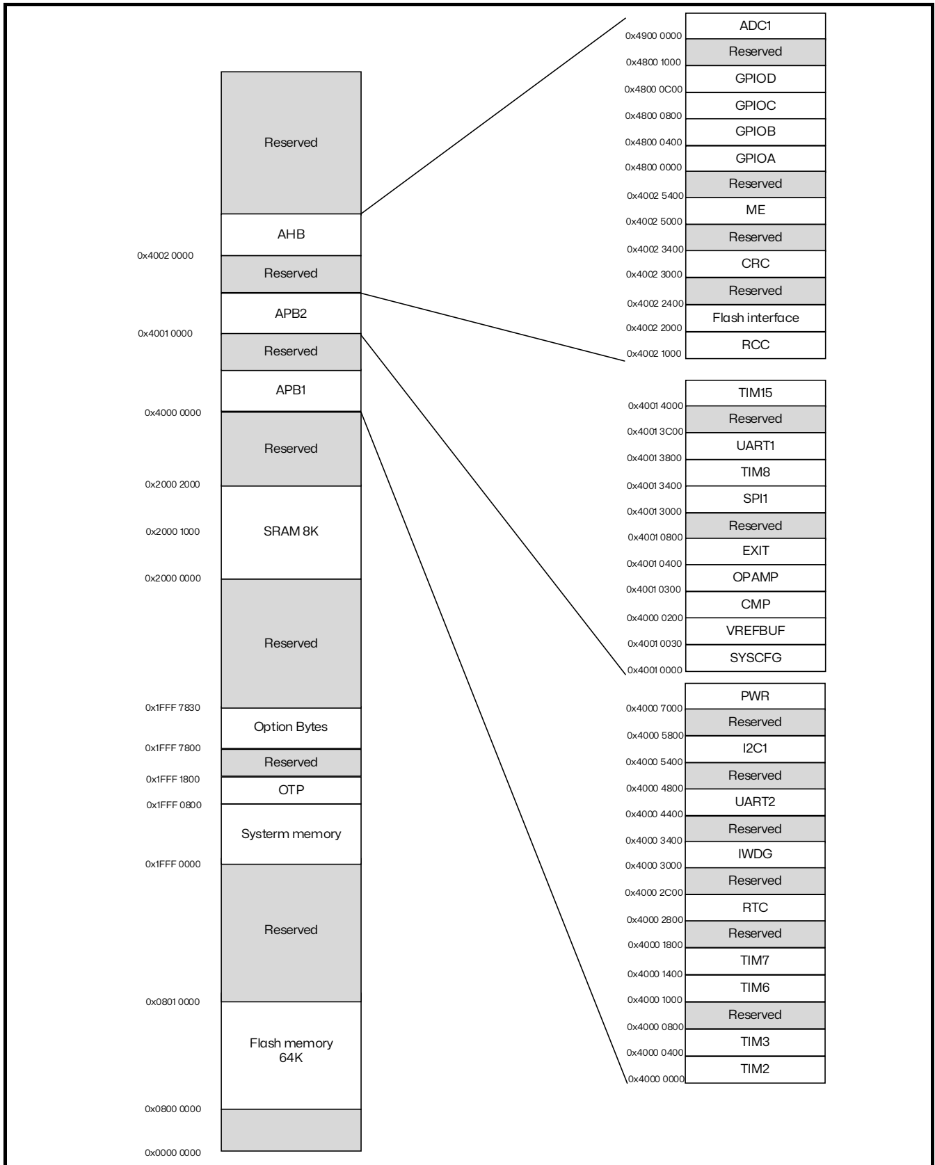
图 3.1 存储器映像
