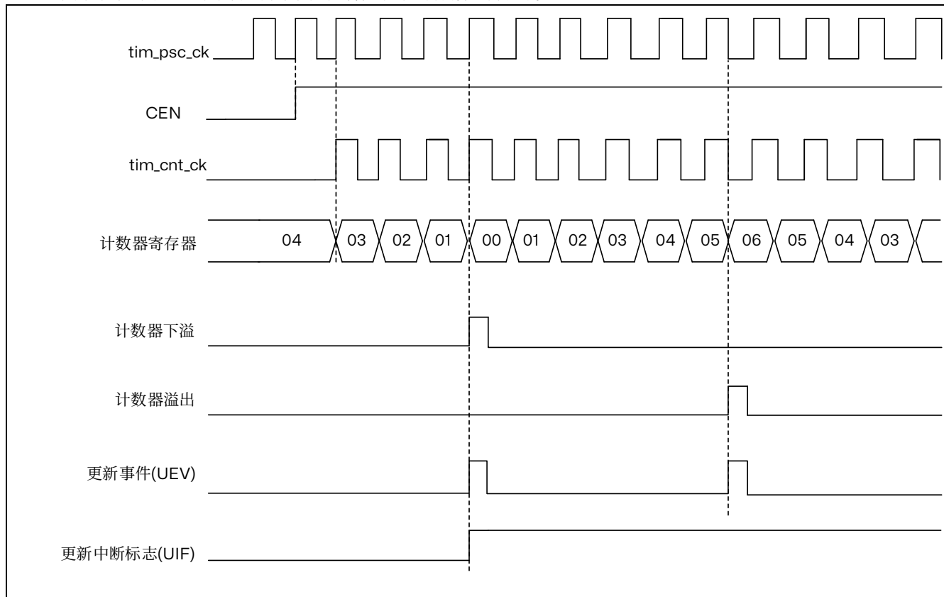
图 15.16 计数器时序图，内部时钟分频因子为 1，TIMx_ARR=0x6
