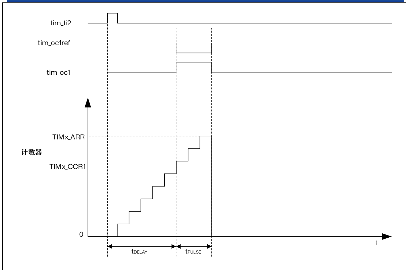
图 15.47 单脉冲模式的例子
