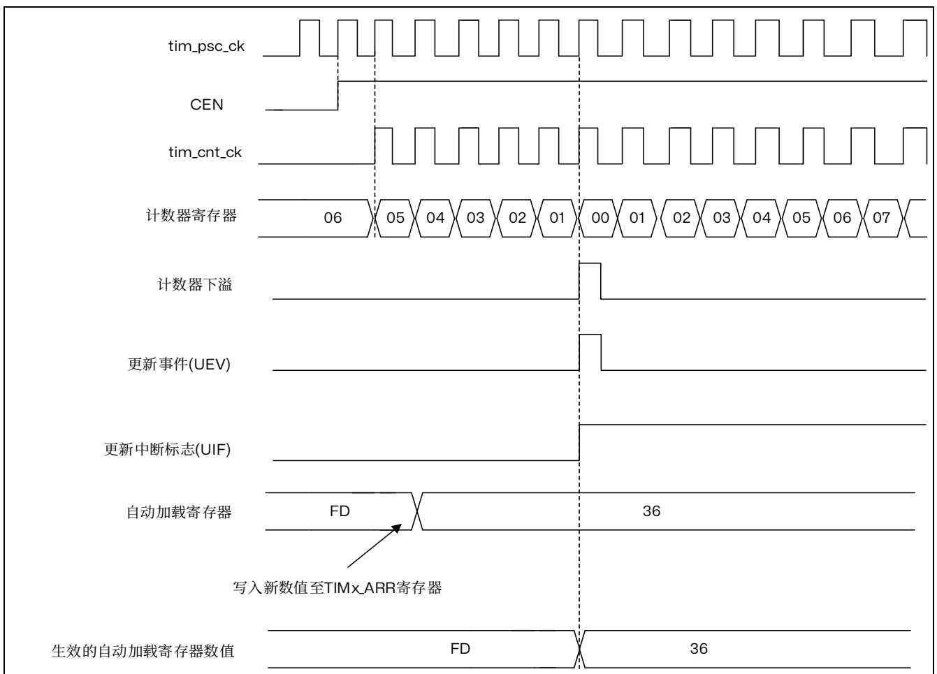
图 15.19 计数器时序图，内部时钟分频因子为 N
