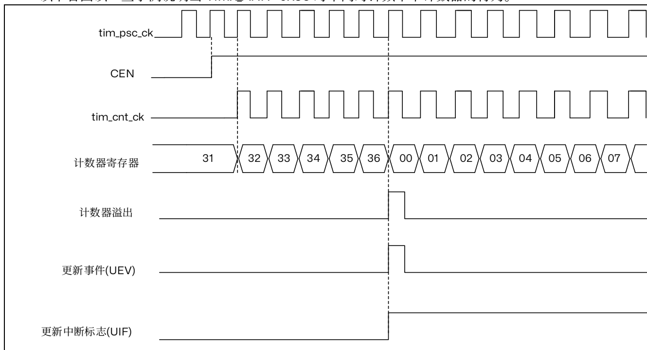
图 15.5 计数器时序图，内部时钟分频因子为 1
