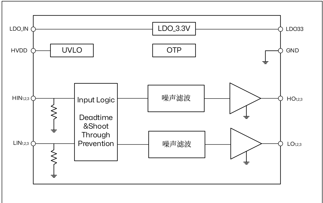
图 26.1 GateDriver 内部结构
