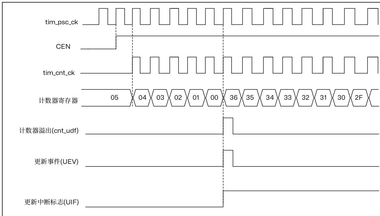
图 15.11 计数器时序图，内部时钟分频因子为 1
