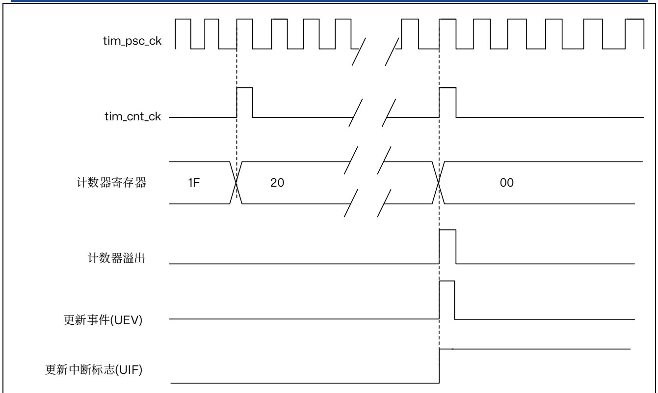
图 15.8 计数器时序图，内部时钟分频因子为 N
