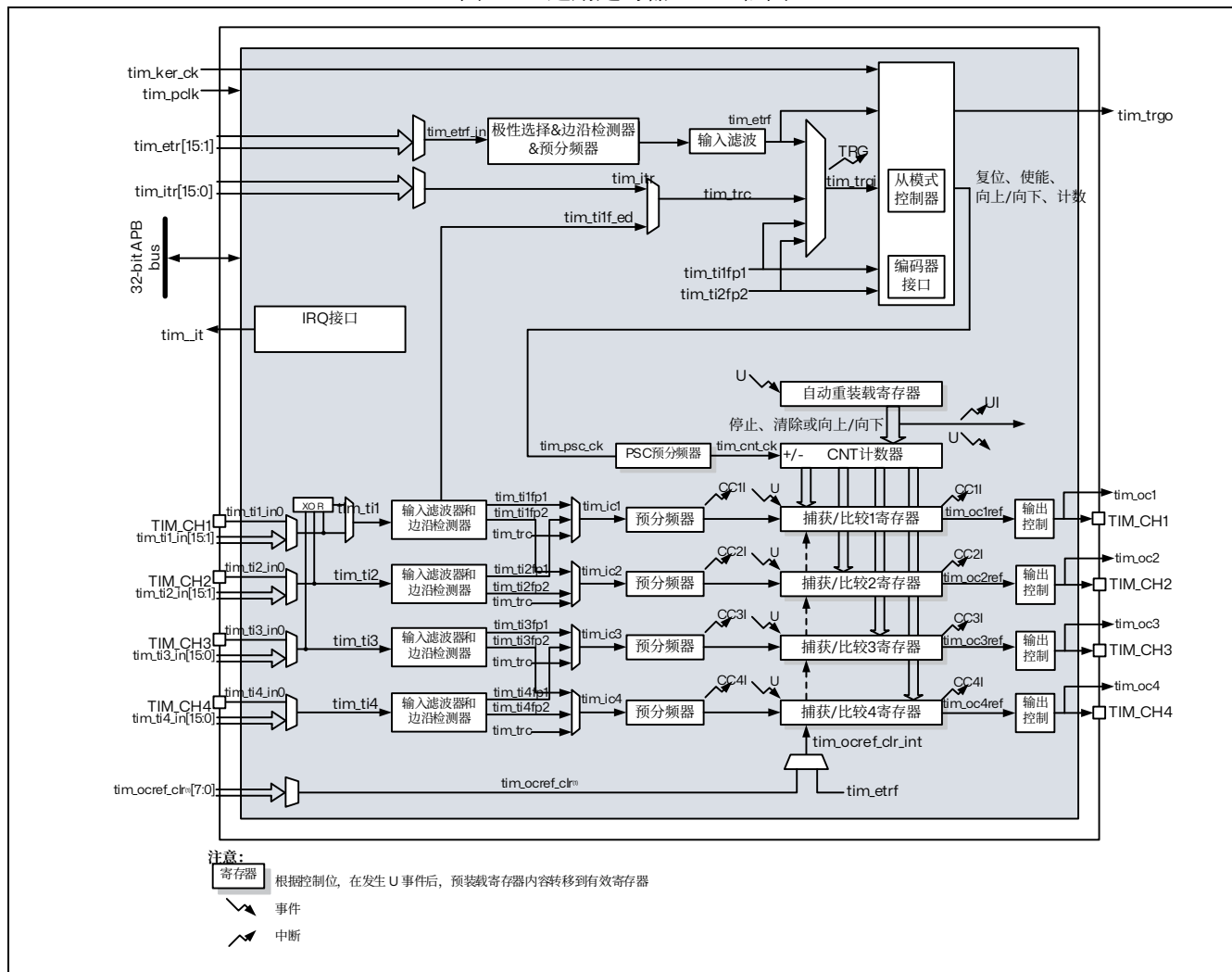
图 15.1 通用定时器 TIM2 框图
