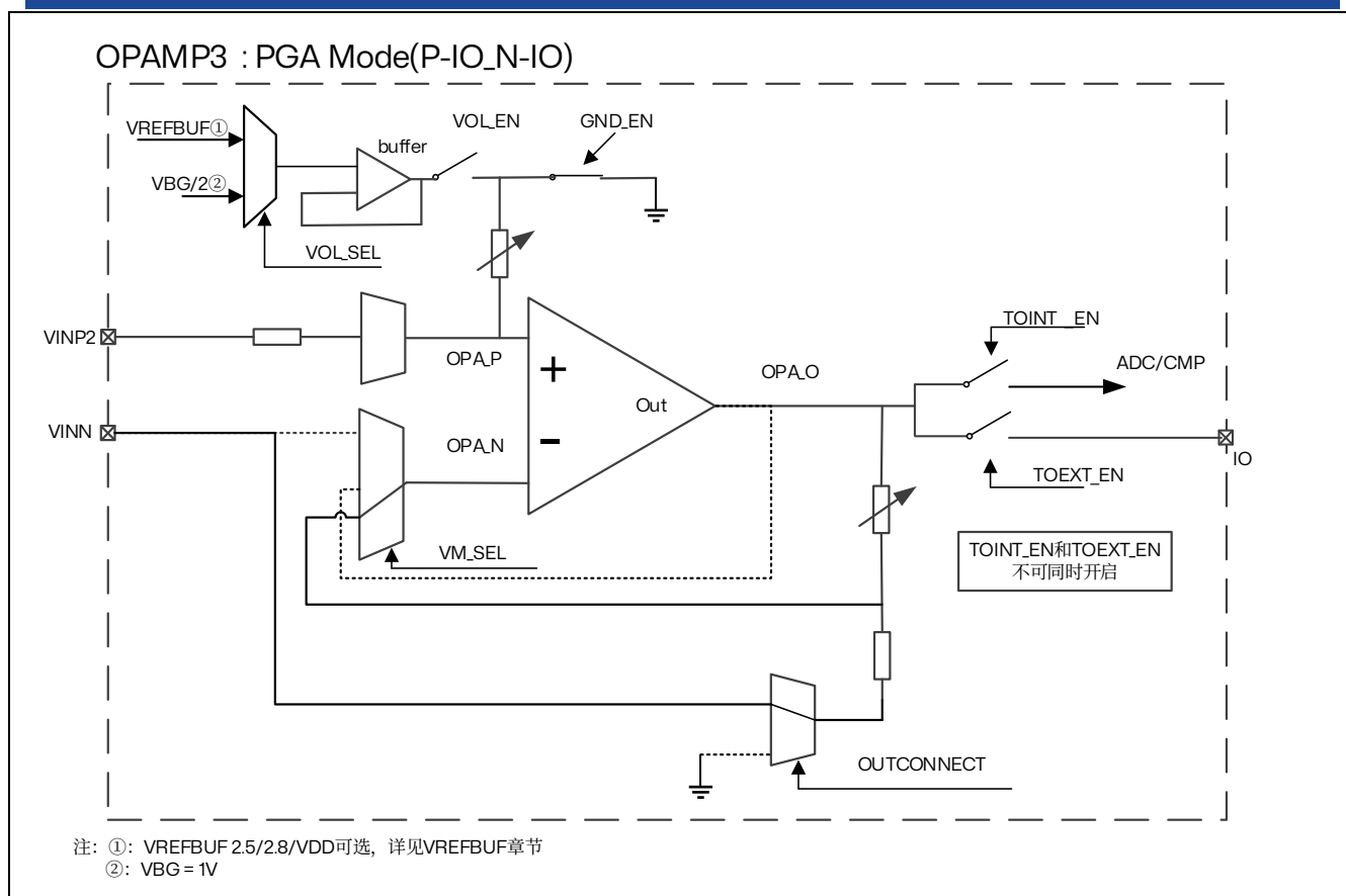
图 18.5 OPAMP3 PGA 模式 (P-IO, N-IO)
