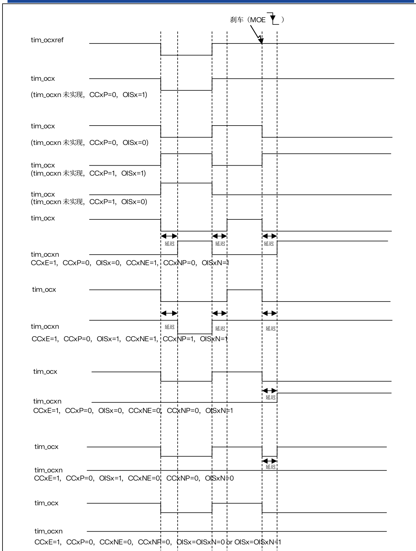
图 14.48 tim_brk 在发生刹车事件时的各种输出行为 (OSSl=1)
