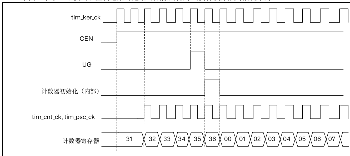
图 17.2 一般模式下的控制电路，内部时钟分频因子为 1
