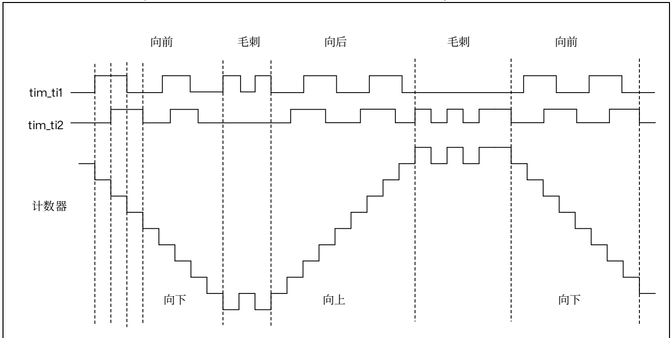
图 15.53 tim_tifp1 极性反相时的编码器接口模式示例
