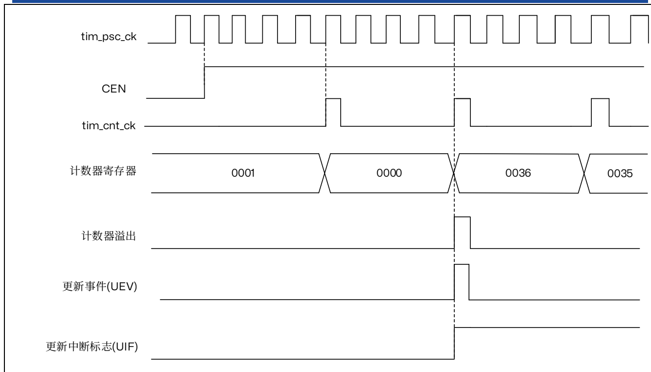
图 15.13 计数器时序图，内部时钟分频因子为 4
