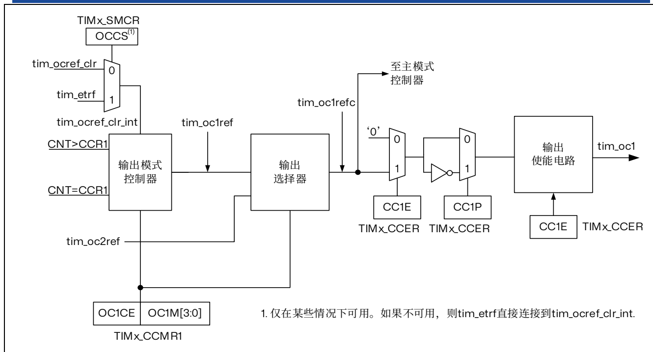
图 15.29 捕获/比较通道的输出阶段 (通道 1, 通道 2、3 和 4 同上)
