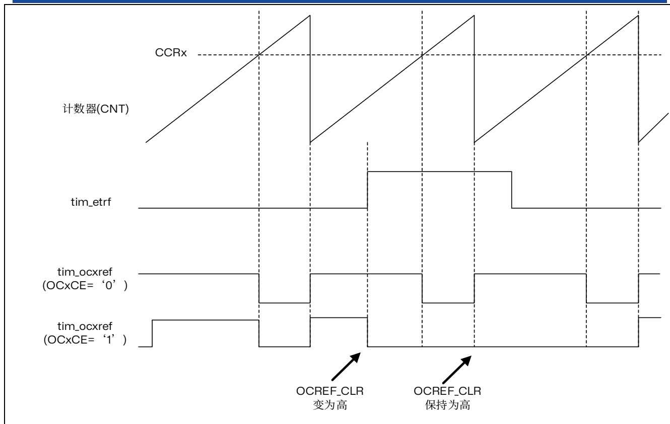
图 15.46 清除 TIMx 的 tim_ocxref
