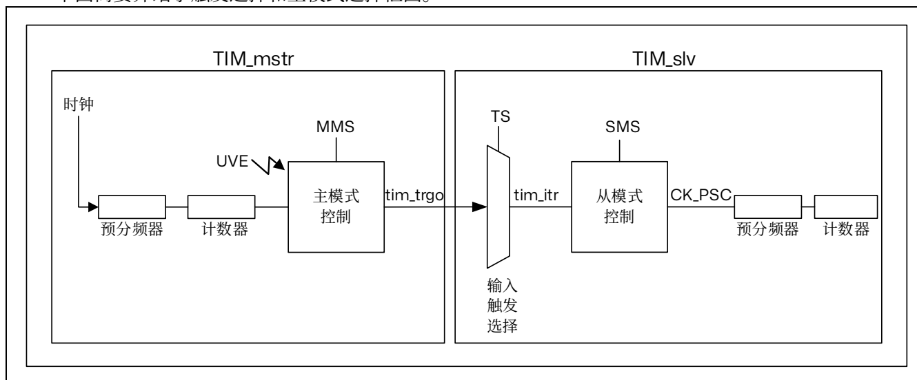
图 15.79 主/从定时器的例子
