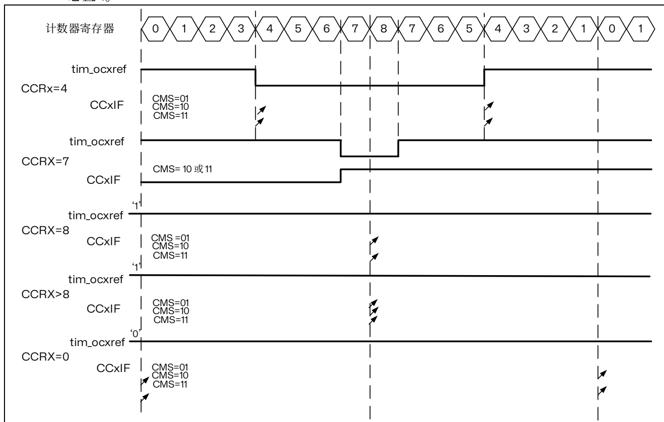
图 15.33 中央对齐的 PWM 波形 (APR=8)
