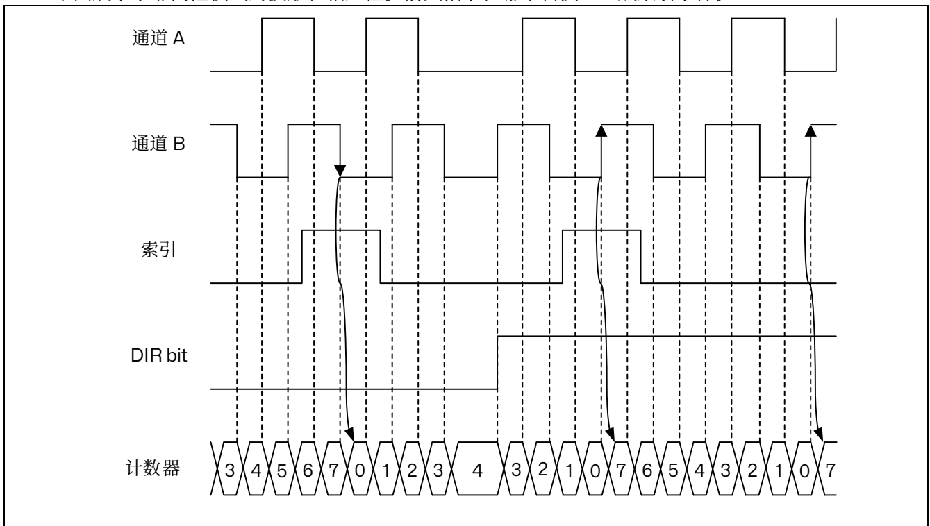
图 15.62 非门控模式下索引的计数器读取 (IPOS[1:0] = 00)
