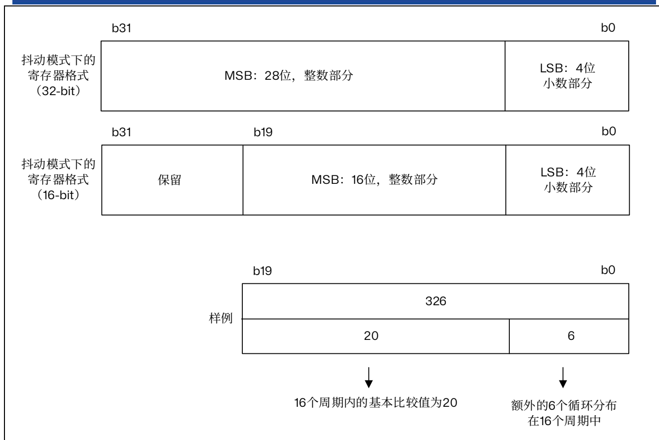
图 15.35 抖动模式下的数据格式和寄存器编码
