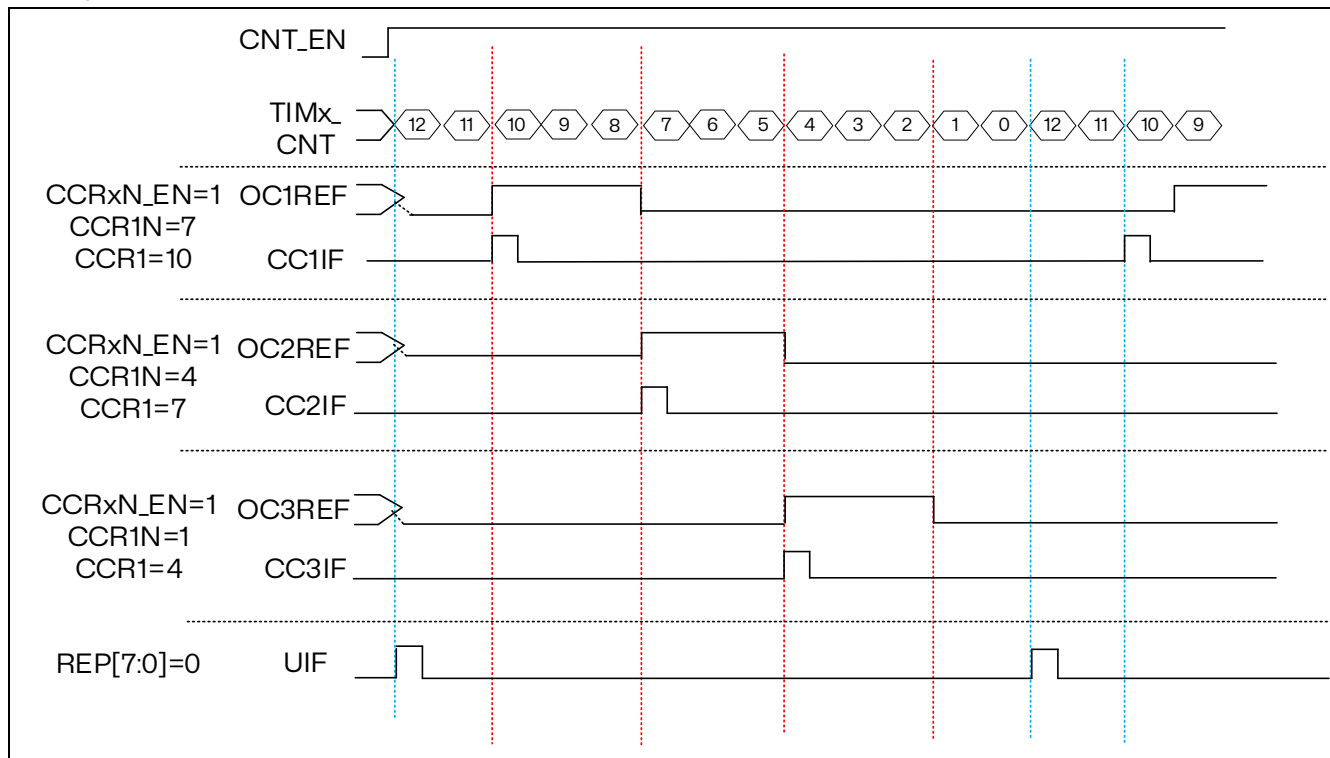
图 15.42 边沿对齐向下计数的 PWM 波形 (ARR=12)
