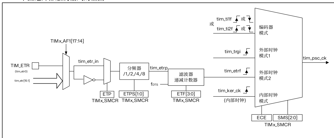
图 15.25 外部触发输入框图
