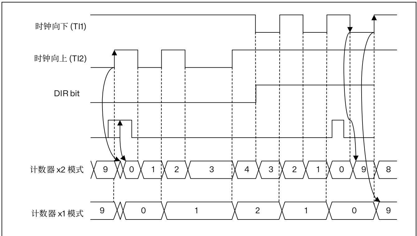
图 15.70 方向时钟模式下的索引行为，IPOS[0] = 1
