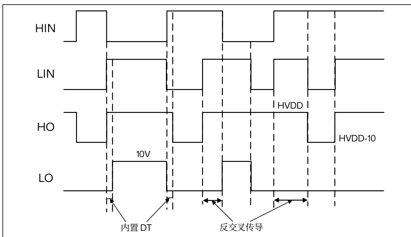
图 26.2 输入输出时序波形
