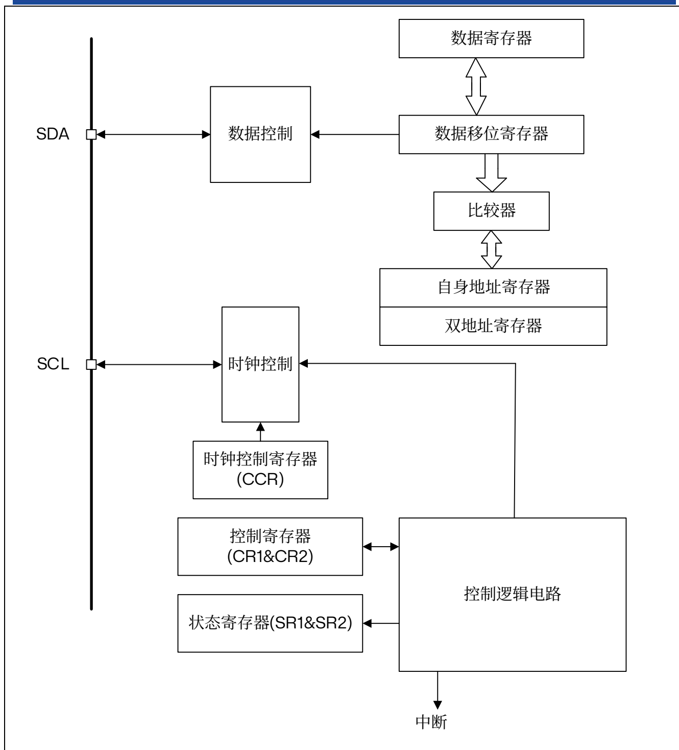
图 24.2 I²C 的功能框图
