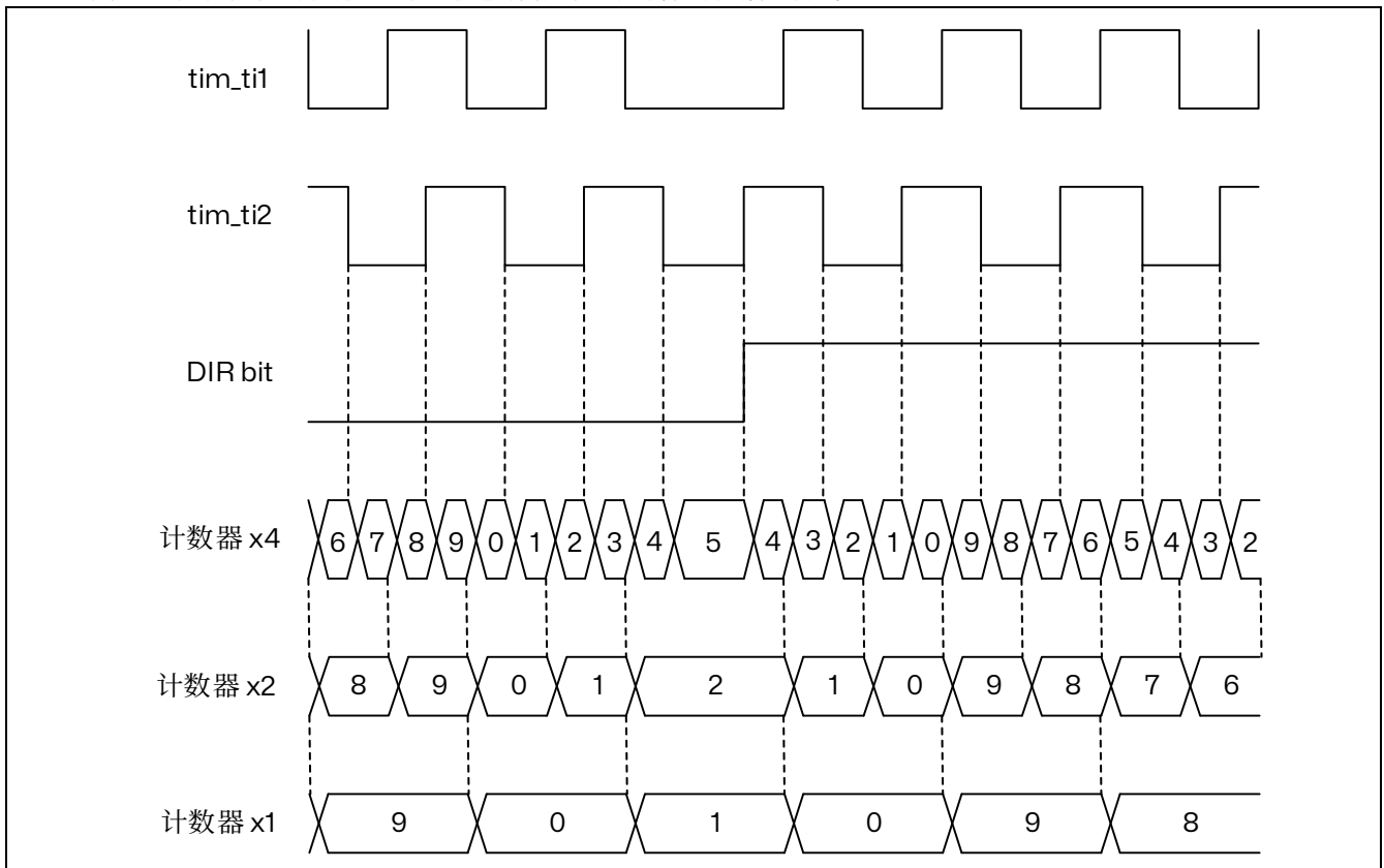
图 15.54 正交编码器的计数模式
