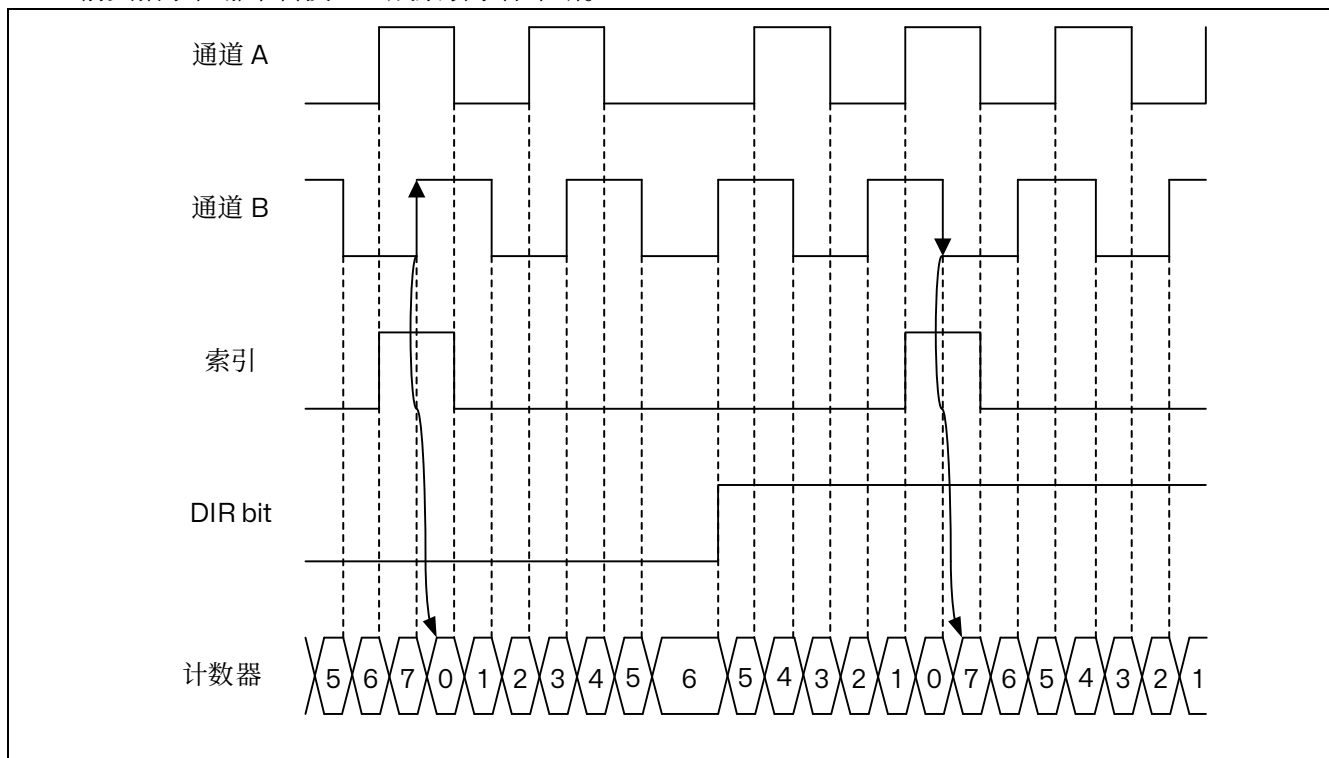
图 15.61 通道 A 上带索引门控的计数器读取 (IPOS[1:0] = 11)
