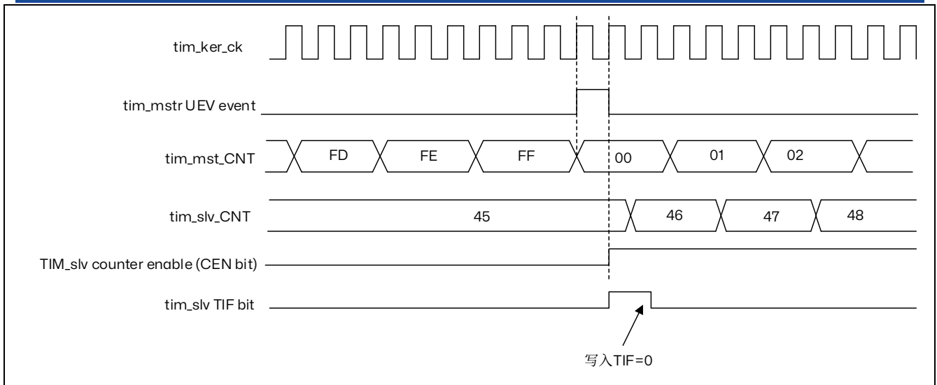
图 15.83 使用 TIM_mstr 的更新触发 TIM_slv
