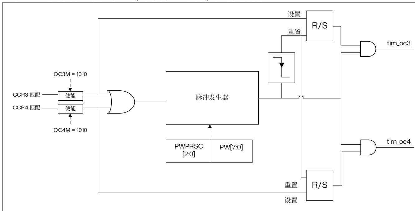
图 15.49 脉冲发生器电路
