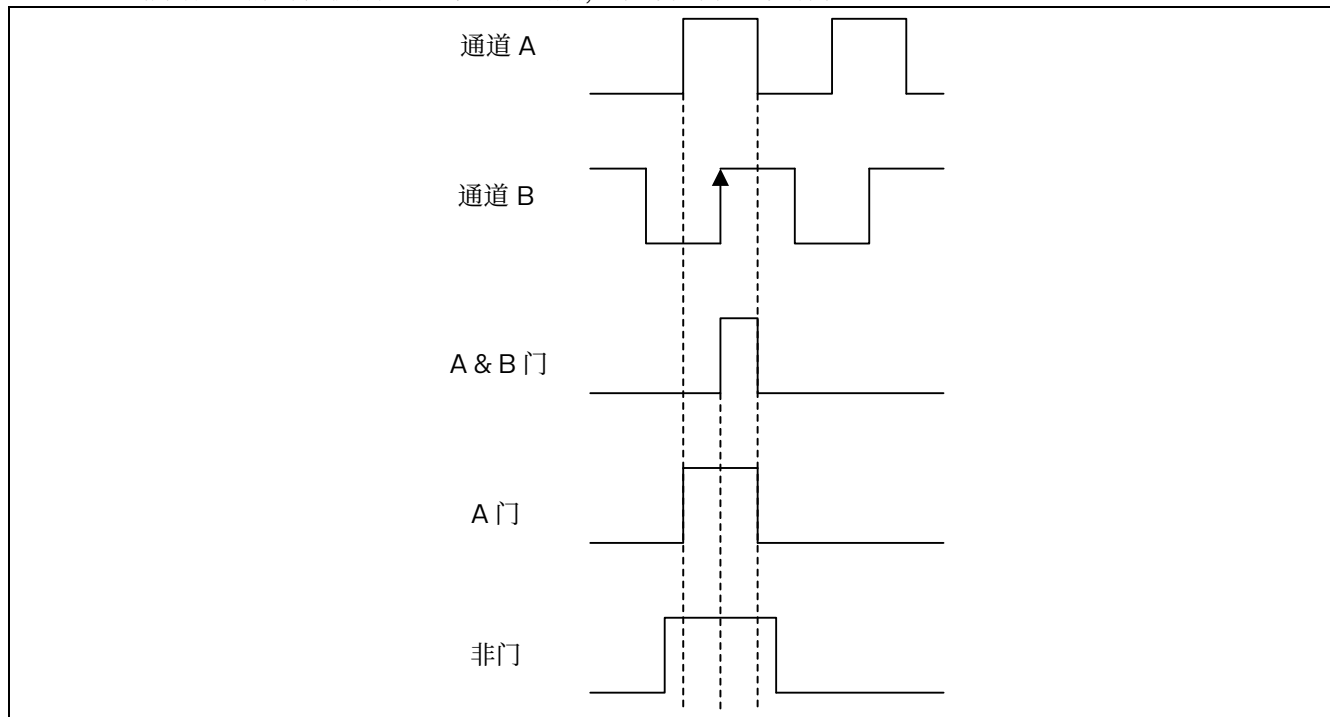
图 15.58 索引门控选项
