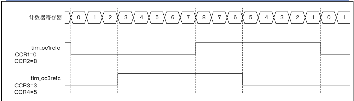
图 15.40 生成两个具有 50%占空比的相位偏移 PWM 信号
