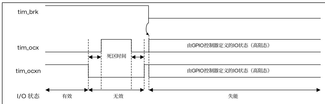
图 14.49 当 tim_brk/tim_brk2 有效 (OSS1=0) 时 PWM 输出状态
