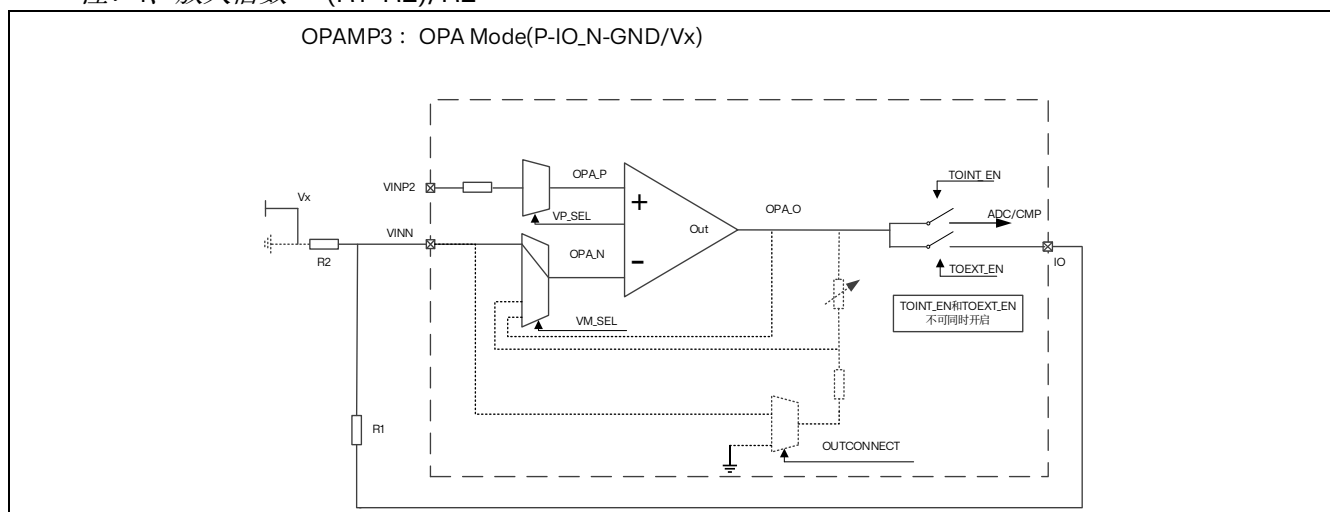
图 18.1 OPAMP3 独立模式
