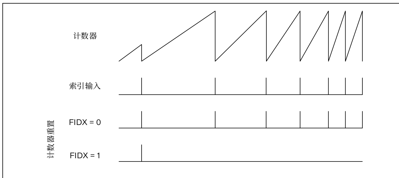
图 15.68 作为 FIDX 位设置的功能的计数器重置
