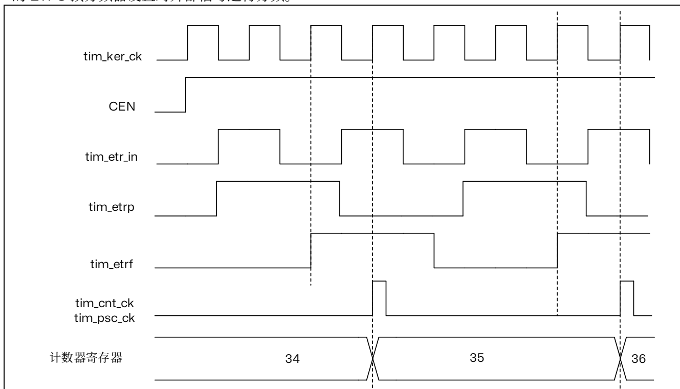
图 15.26 外部时钟模式 2 下的控制电路
