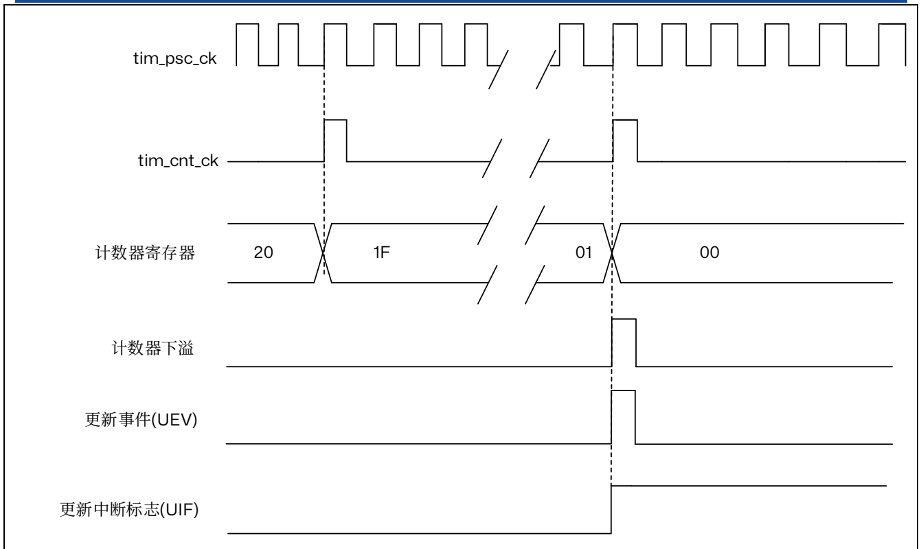
图 15.19 计数器时序图，内部时钟分频因子为 N
