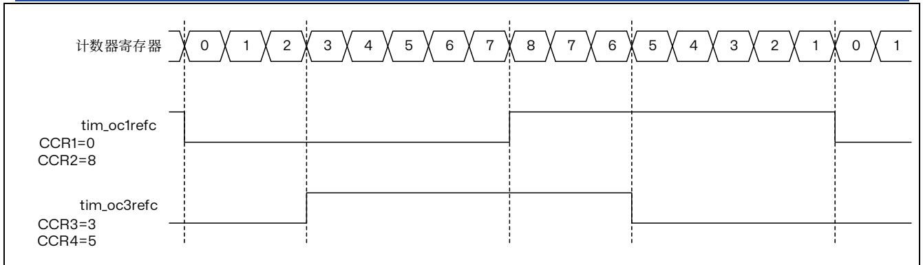
图 14.37 生成两个具有 50%占空比的相位偏移 PWM 信号
