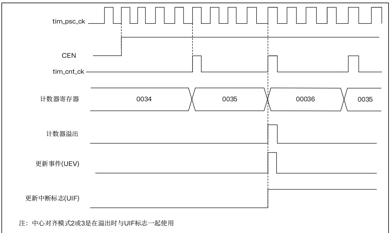
图 14.17 计数器时序图，内部时钟分频因子为 4，TIM8_ARR=0x36
