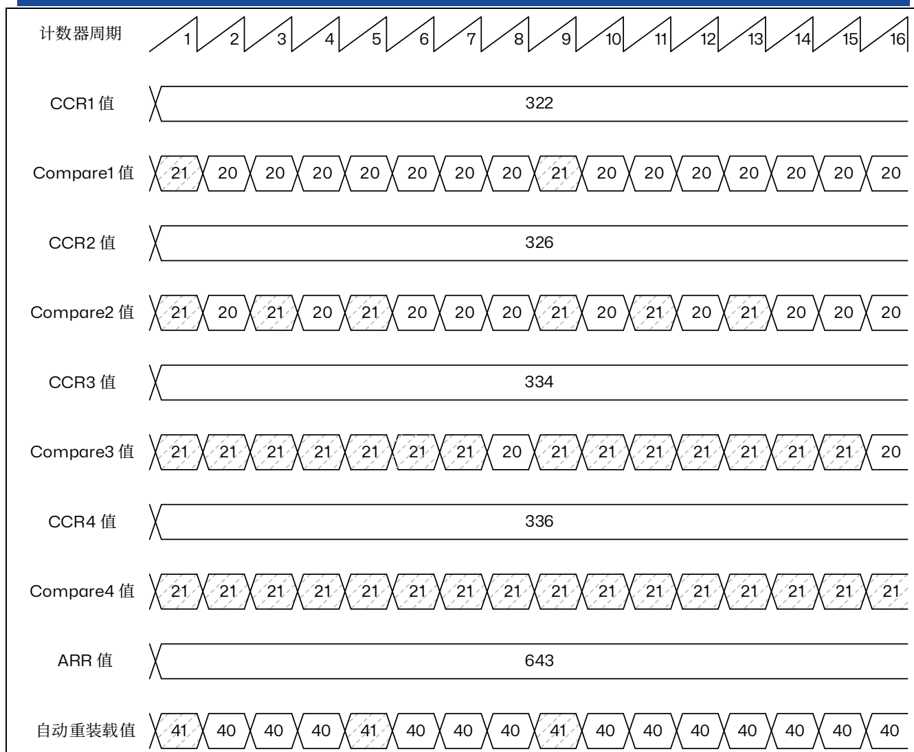
图 15.38 PWM 抖动模式
