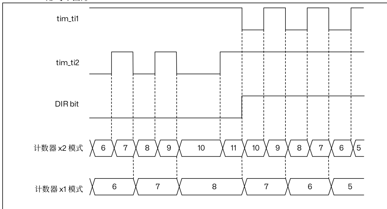
图 15.56 方向时钟编码器模式 ( CC1P=CC2P=0 )
