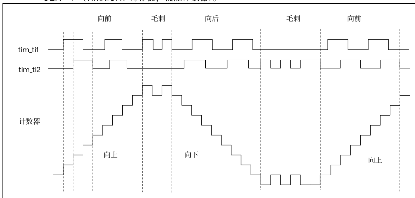
图 15.52 编码器接口模式下的计数器工作示例
