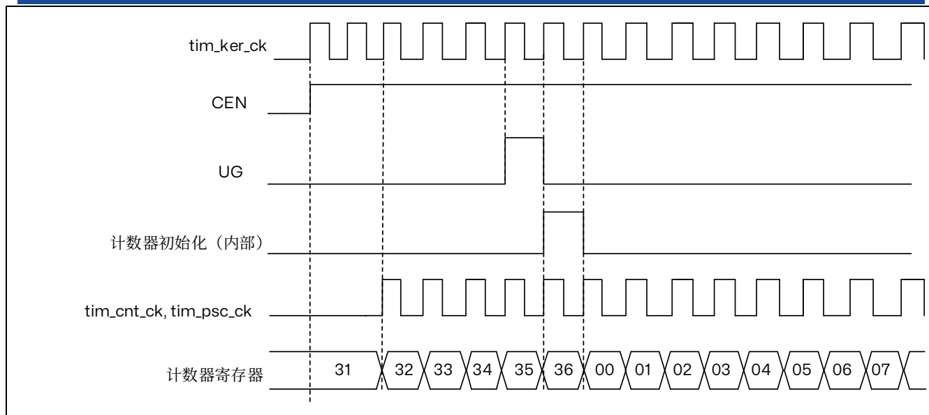
图 15.22 一般模式下的控制电路，内部时钟分频因子为 1
