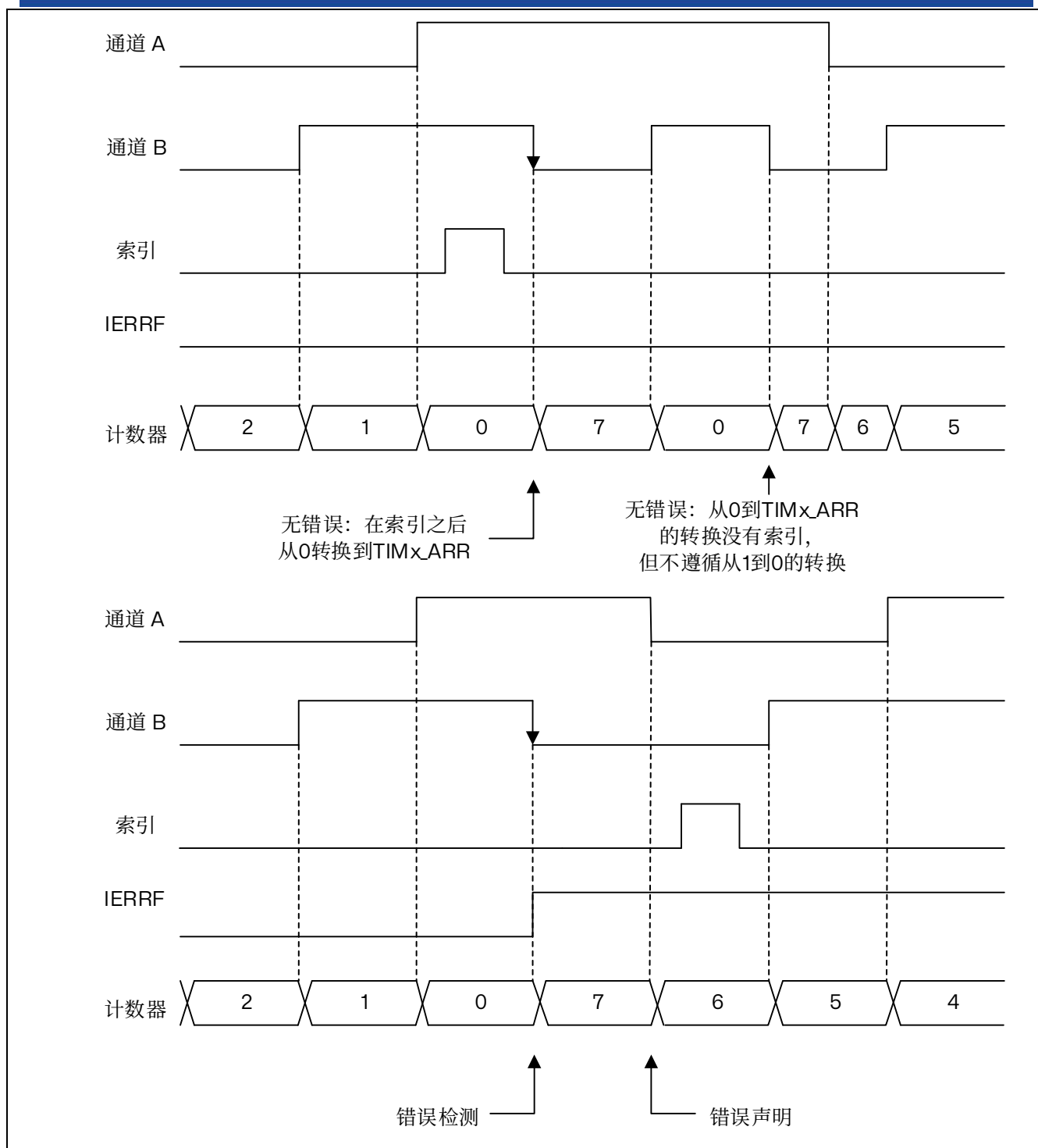
图 15.73 递减计数编码器错误检测
