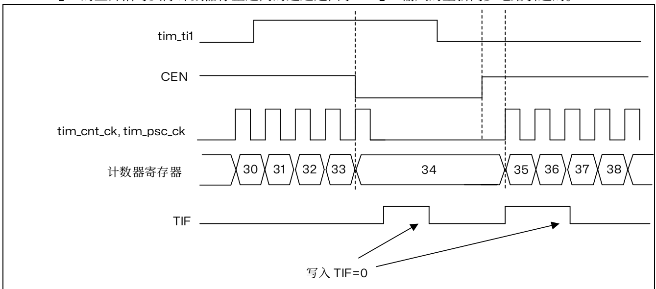
图 15.76 门控模式下的控制电路
