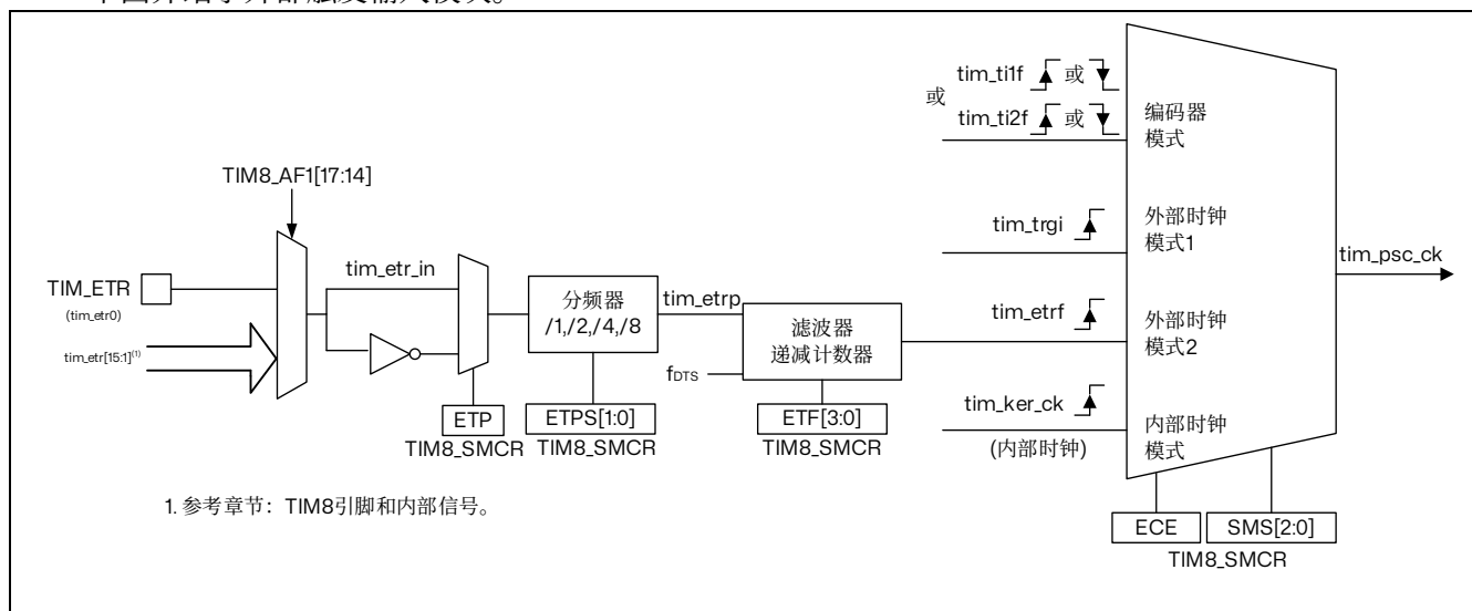
图 14.24 外部触发输入框图
