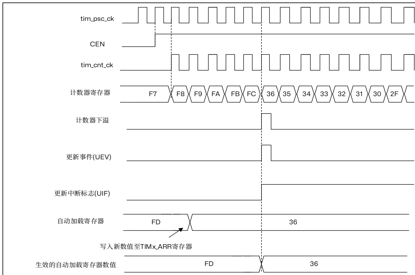
图 15.21 计数器时序图，ARPE=1 时的更新事件（计数器溢出）
