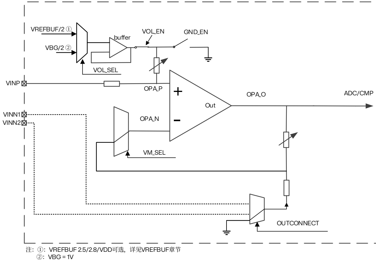
图 18.8 OPAMP1/OPAMP2 PGA 模式 (P-偏置, N-GND)
