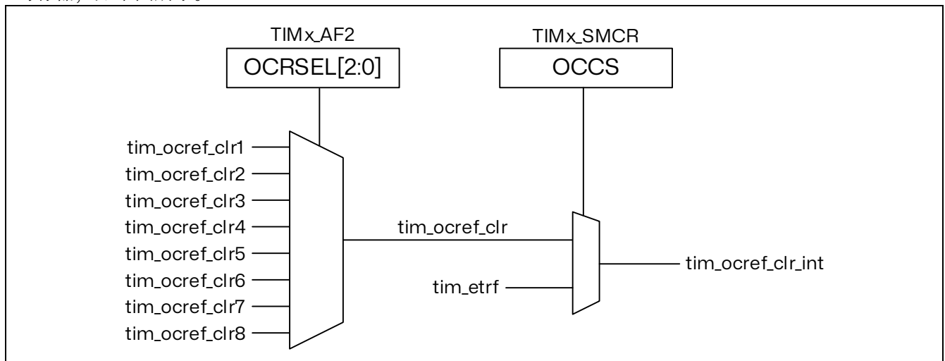
图 15.45 tim_ocref_clr 输入选择复用器
