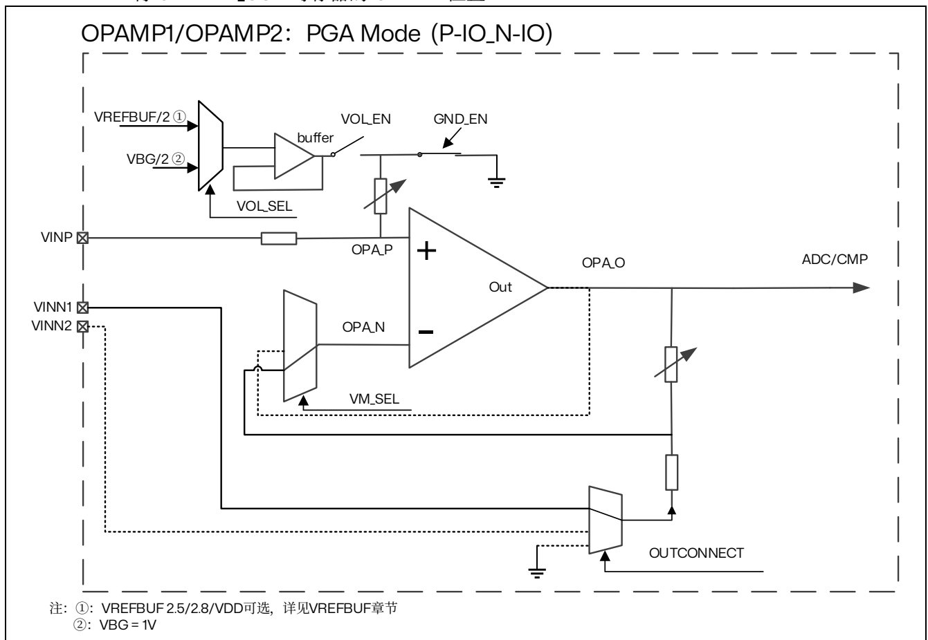
图 18.4 OPAMP1/OPAMP2 PGA 模式 (P-IO, N-IO)
