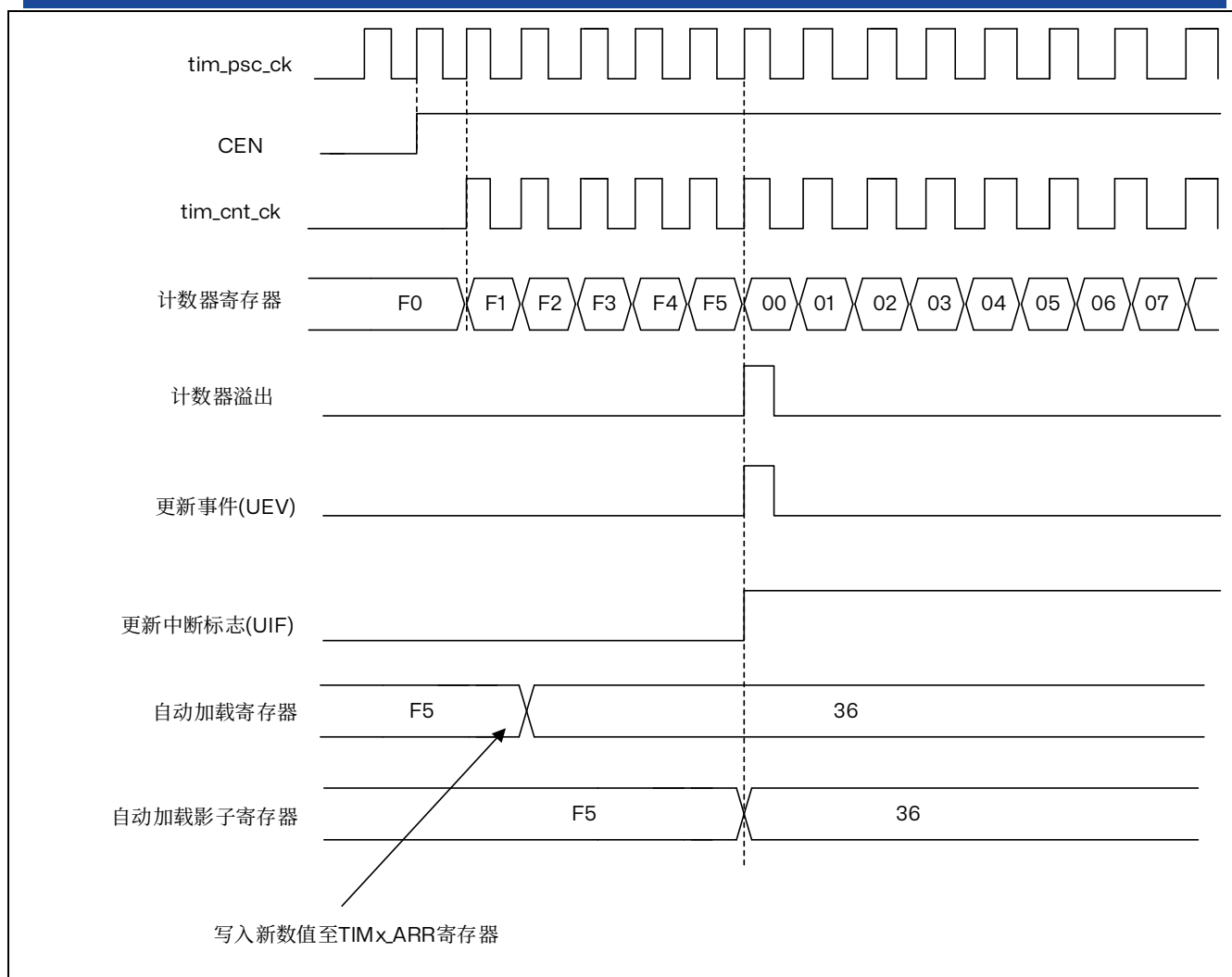
图 15.10 计数器时序图，当 ARPE=1 时的更新事件（预装入了 TIMx_ARR）
