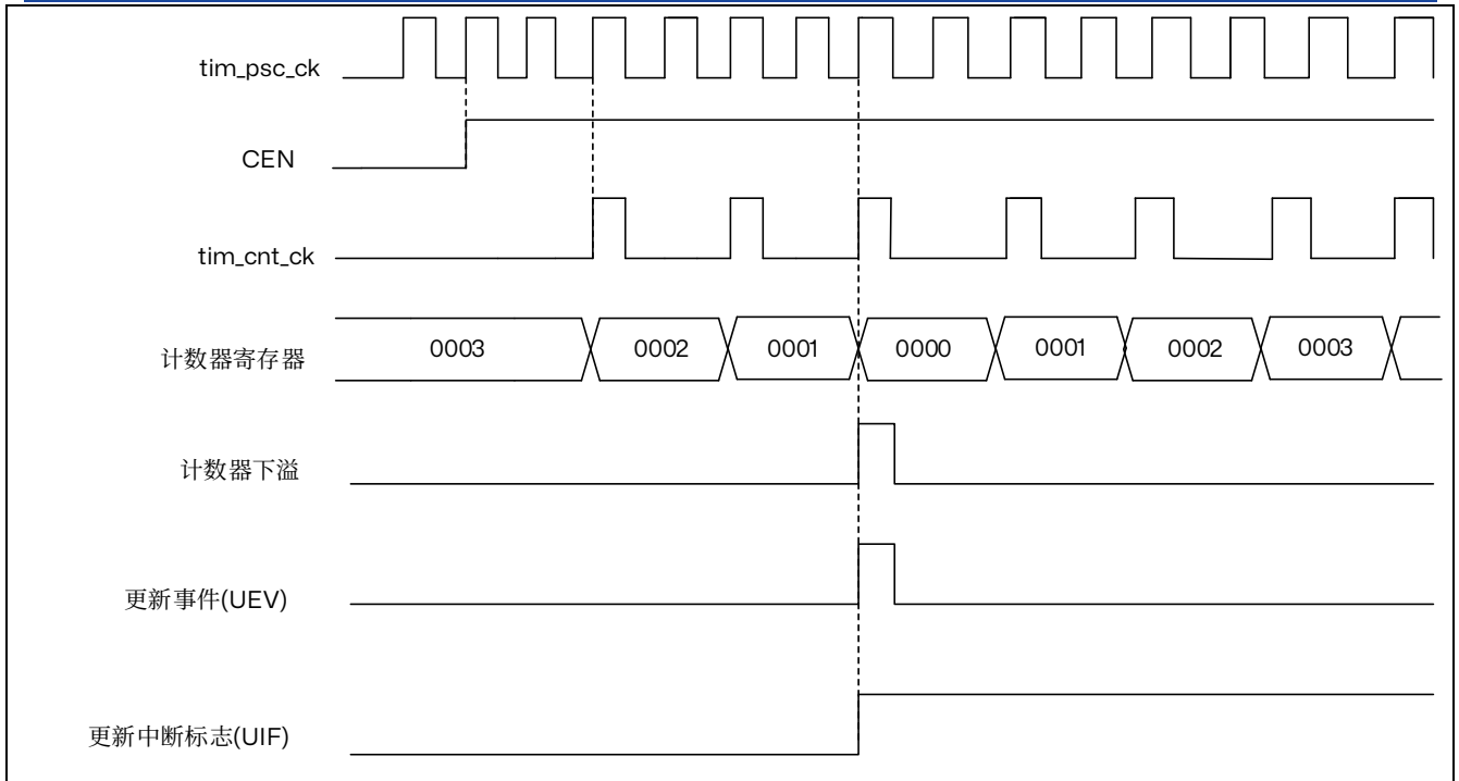
图 15.17 计数器时序图，内部时钟分频因子为 2
