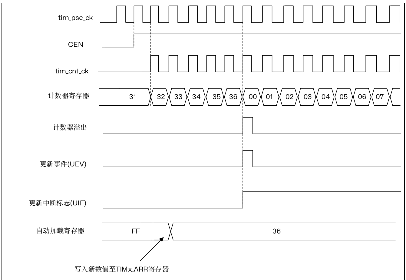
图 15.9 计数器时序图，当 ARPE=0 时的更新事件 (TIMx_ARR 没有预装入)
