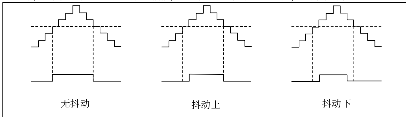
图 15.39 中央对齐 PWM 模式下抖动对占空比的影响
