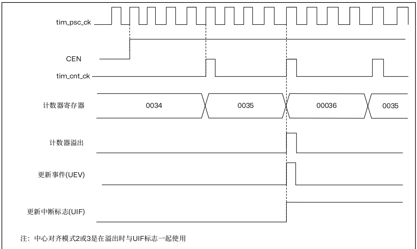
图 15.18 计数器时序图，内部时钟分频因子为 4，TIMx_ARR=0x36
