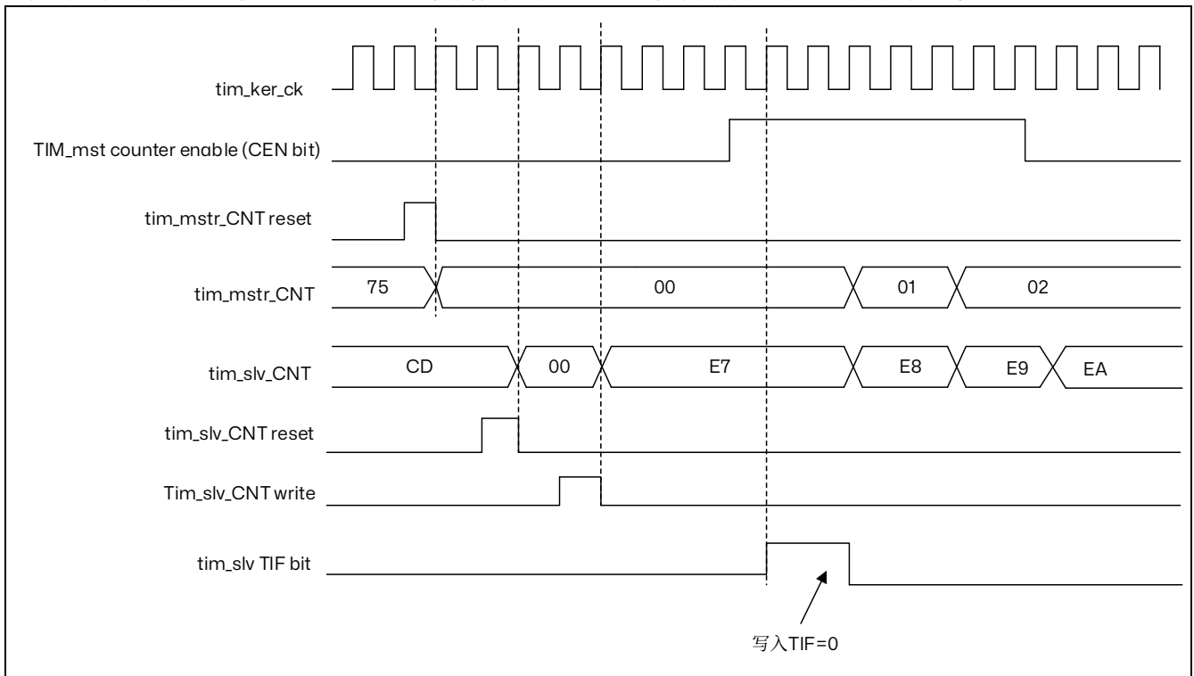
图 15.84 利用 TIM_mstr 的使能触发 TIM_slv
