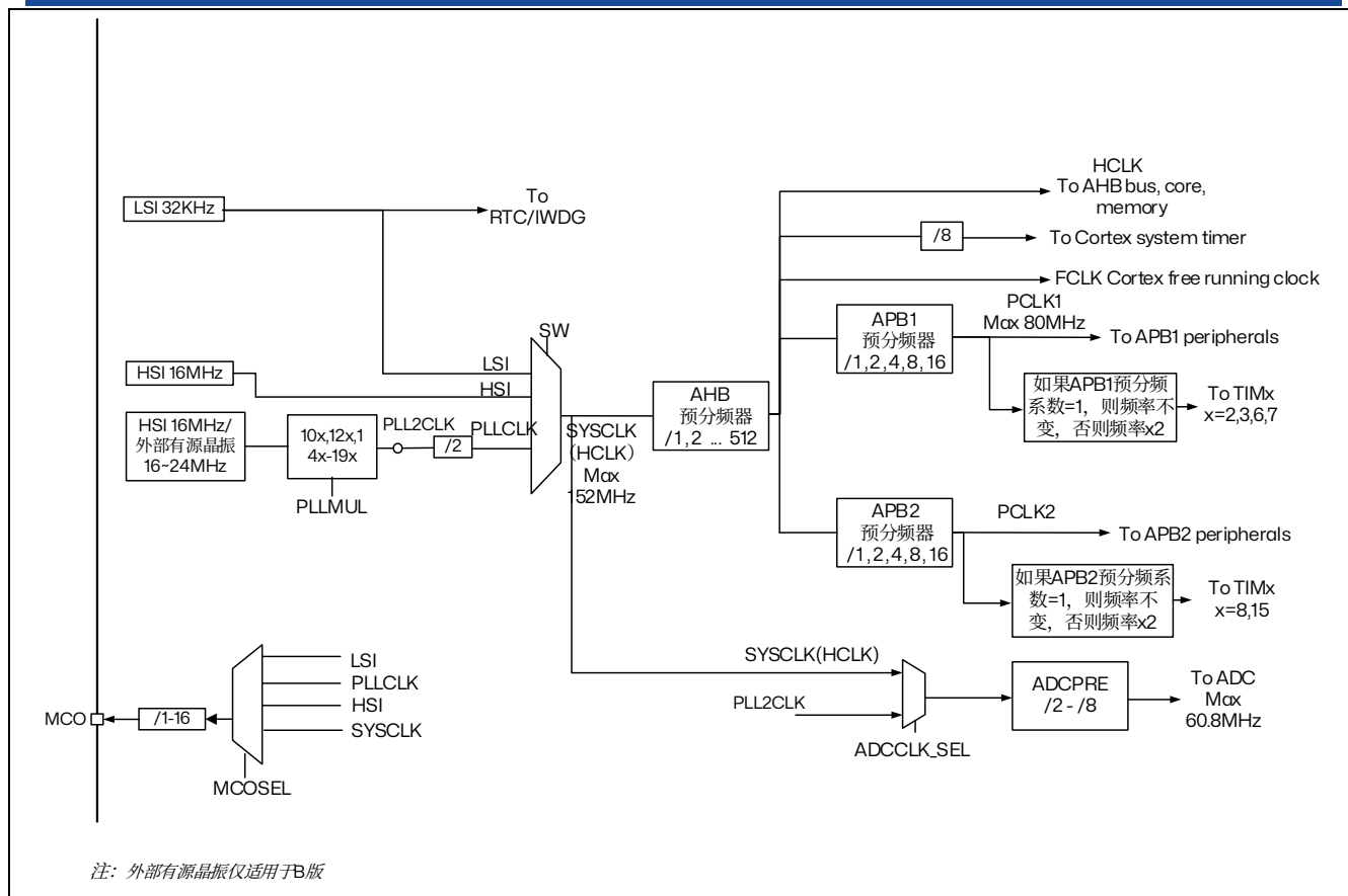
图 7.2 时钟树
