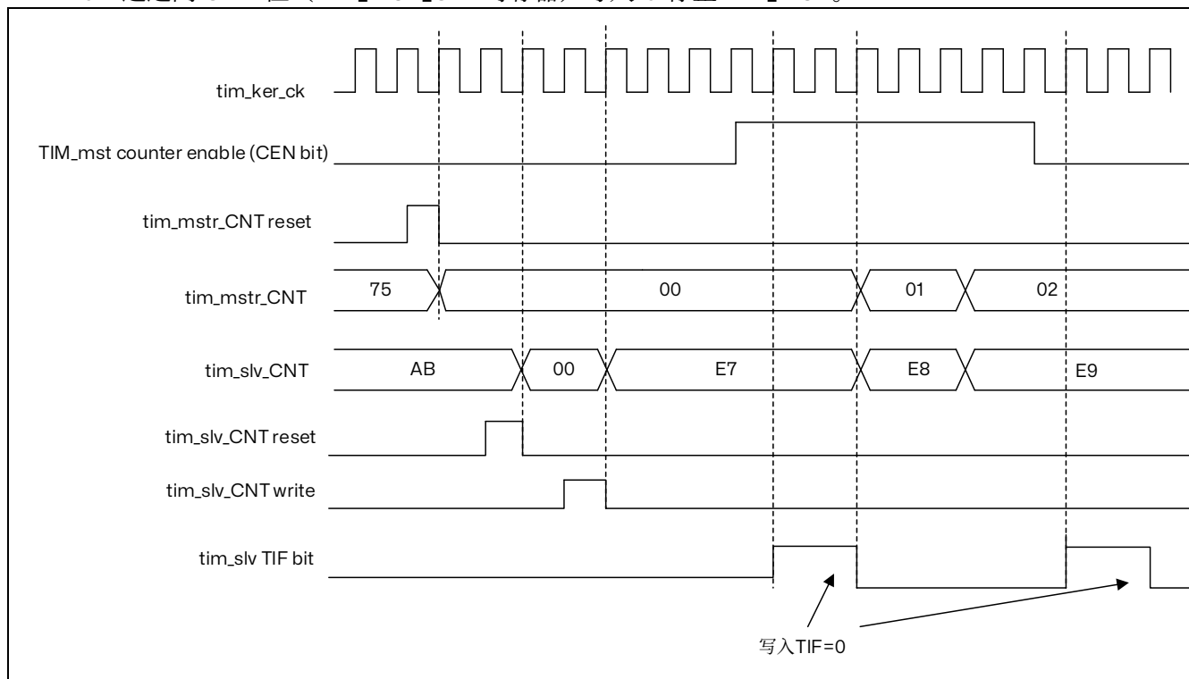
图 15.82 通过使能 TIM_mstr 可以控制 TIM_slv
