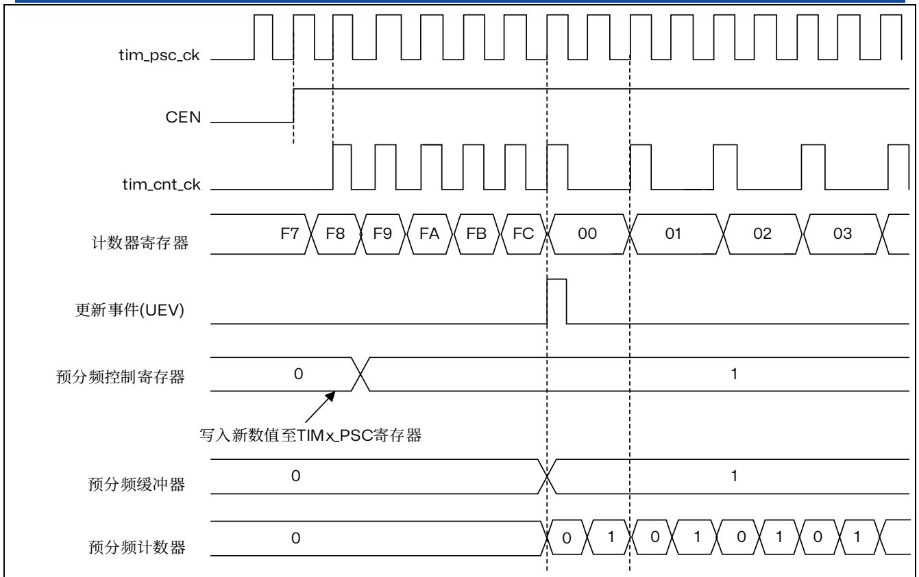
图 15.3 当预分频器的参数从1变到2时，计数器的时序图
