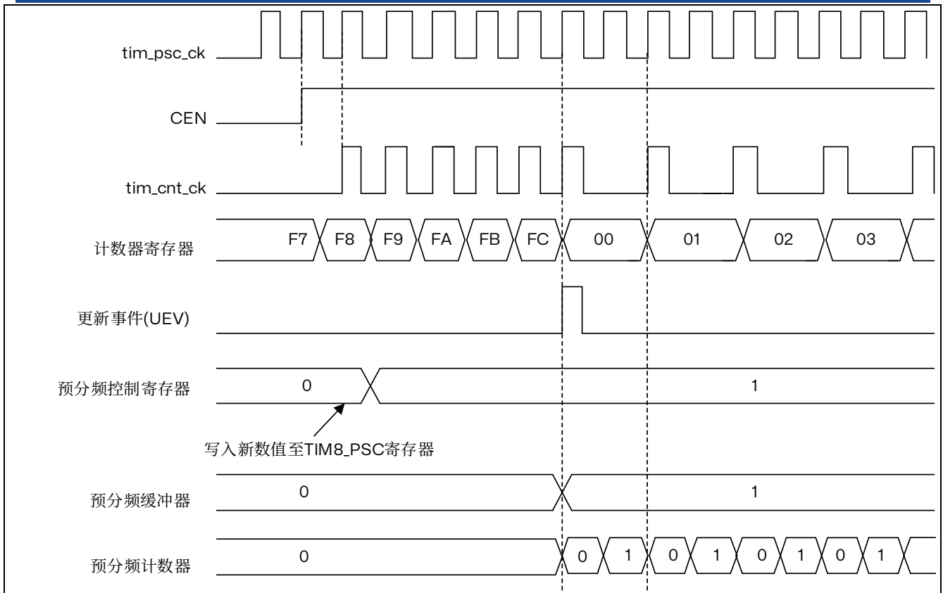
图 14.2 当预分频器的参数从1变成2时，计数器的时序图
