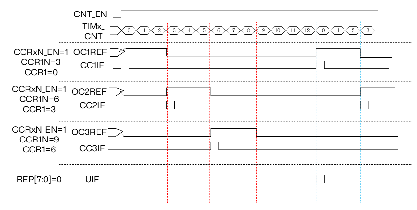
图 15.41 边沿对齐向上计数的 PWM 波形（ARR=12）
