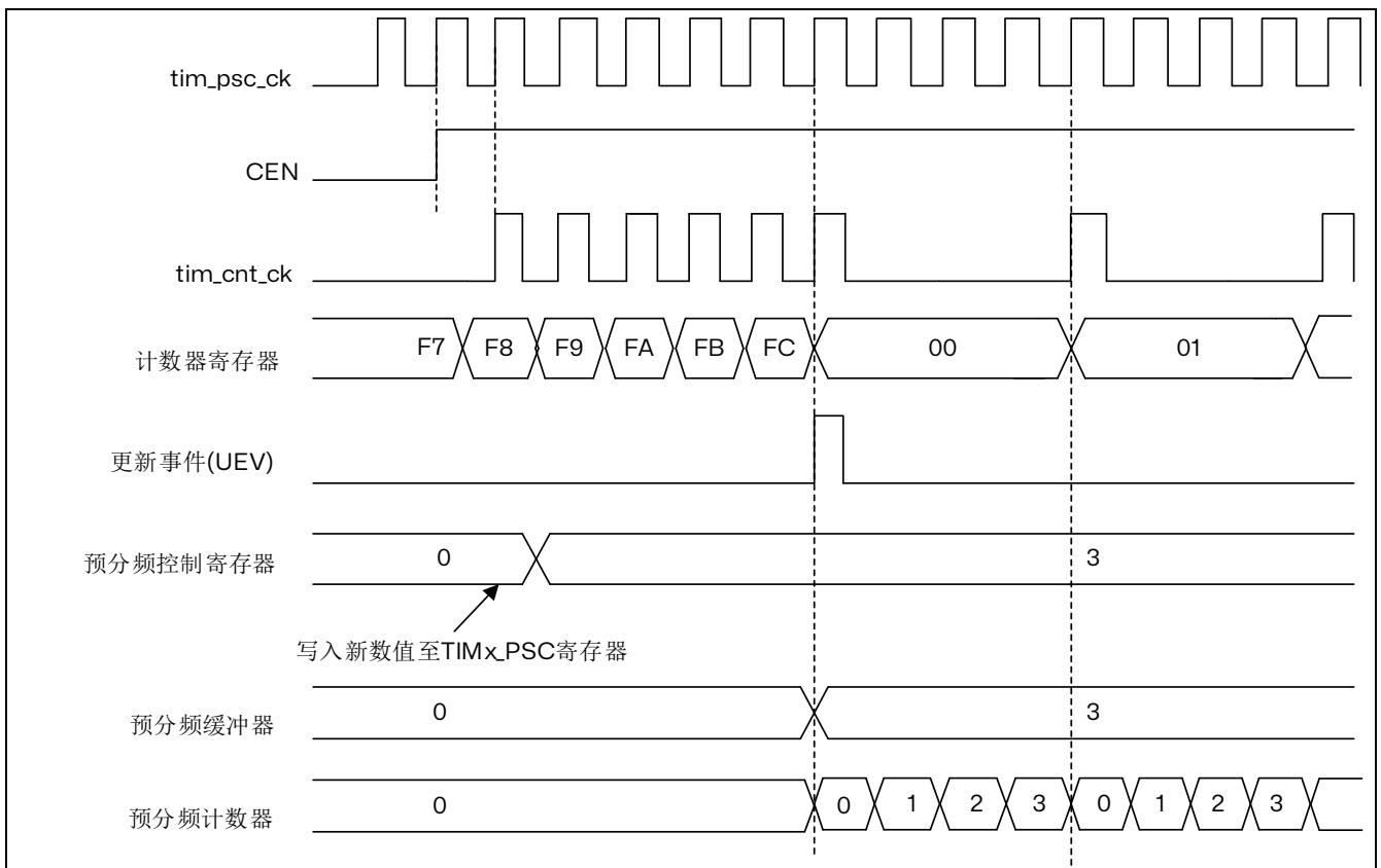
图 15.4 当预分频器的参数从1变到4时，计数器的时序图
