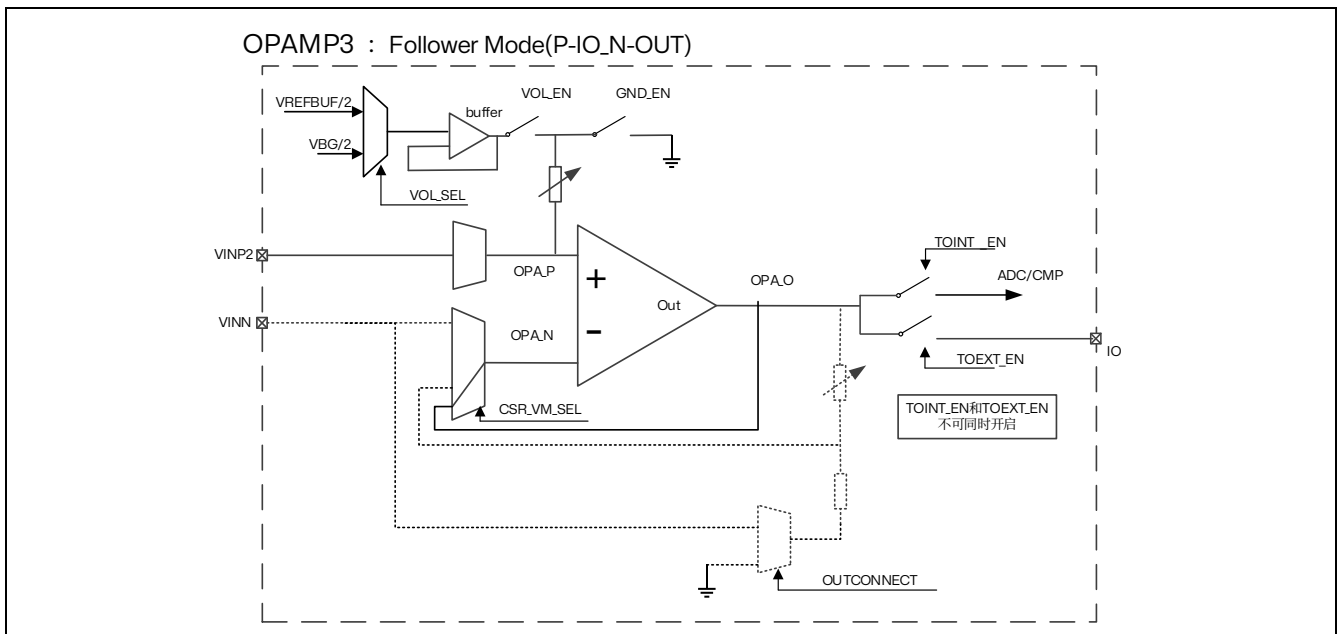
图 18.3 OPAMP3 电压跟随器模式
