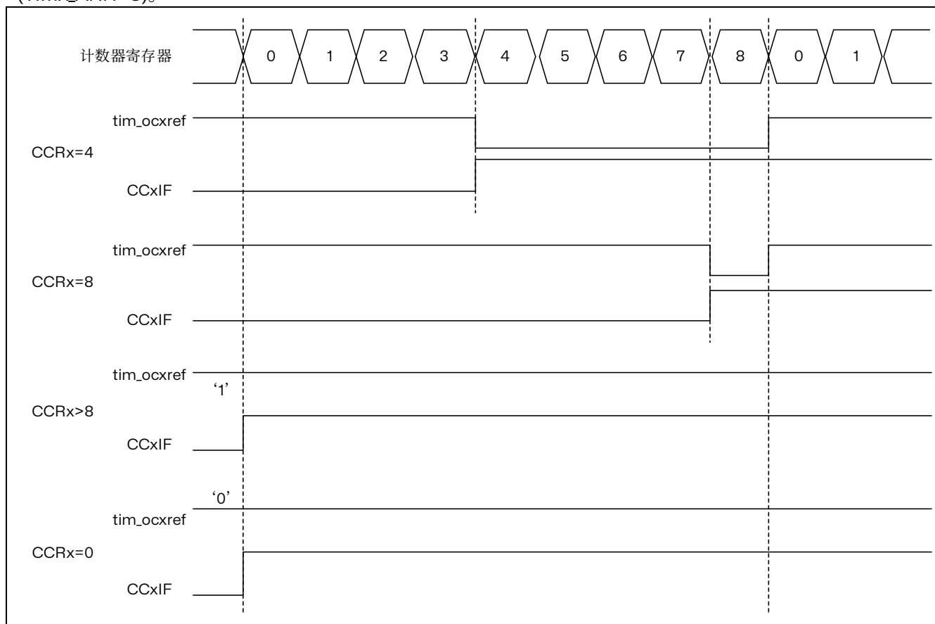
图 15.32 边沿对齐的 PWM 波形（ARR=8）
