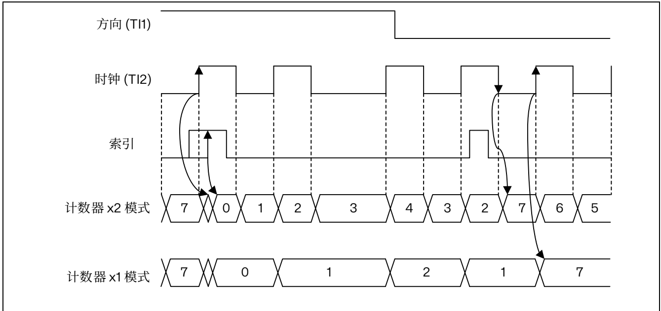
图 15.69 时钟+方向模式下的索引行为，IPOS[0] = 1
