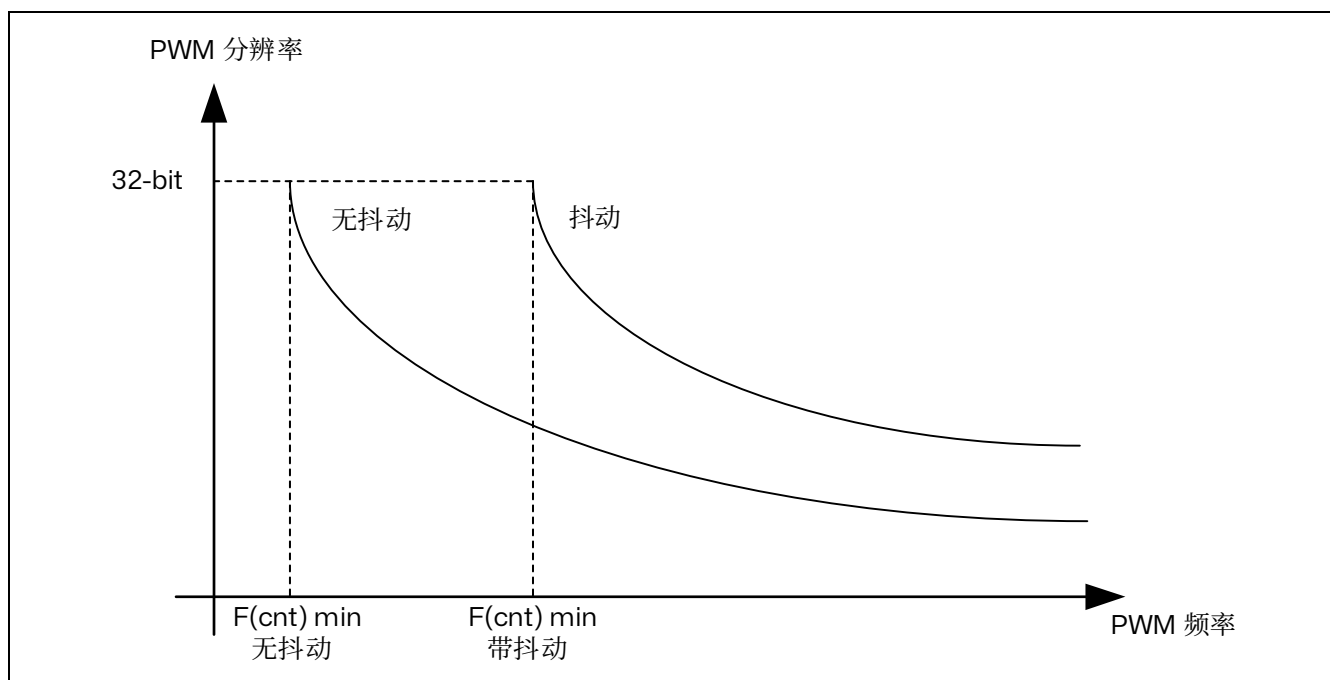
图 15.37 PWM 分辨率 vs 频率 (32 位模式)
