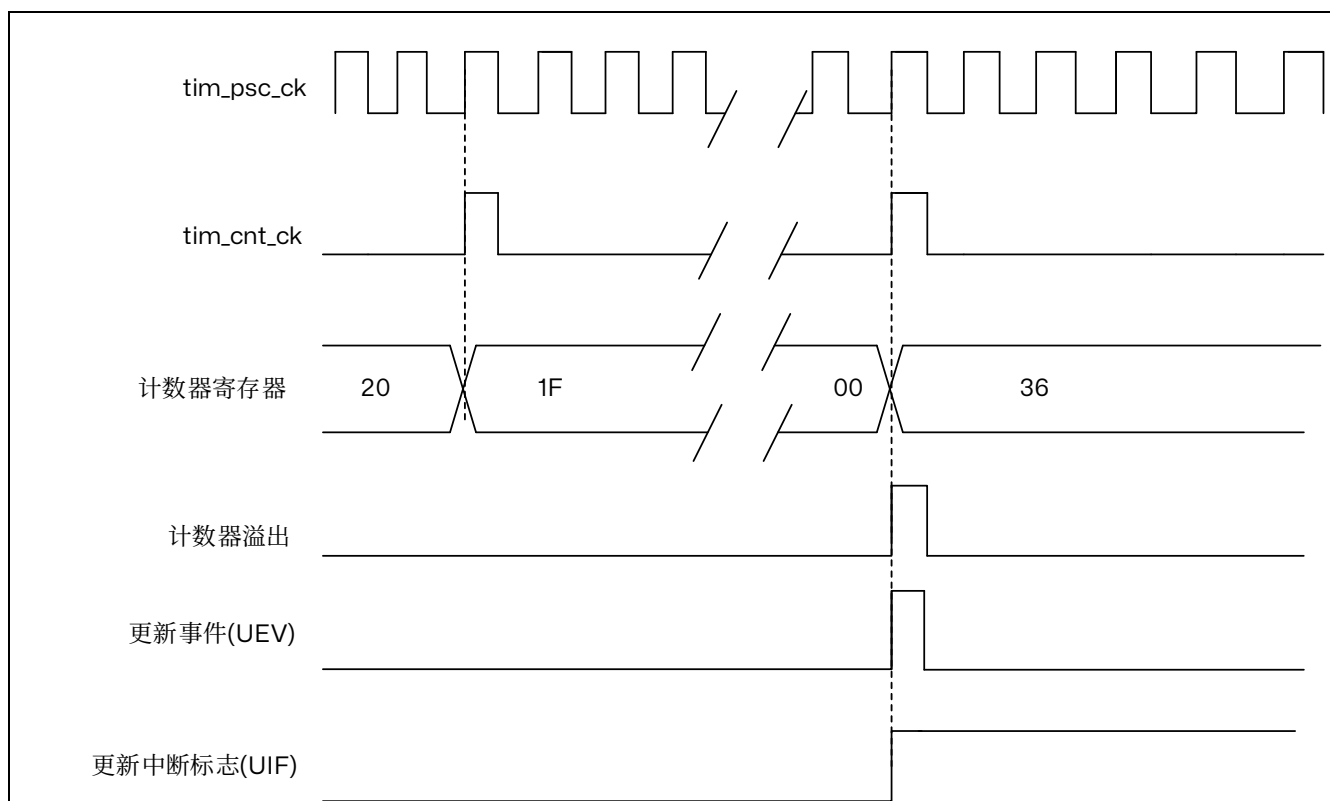
图 15.14 计数器时序图，内部时钟分频因子为 N
