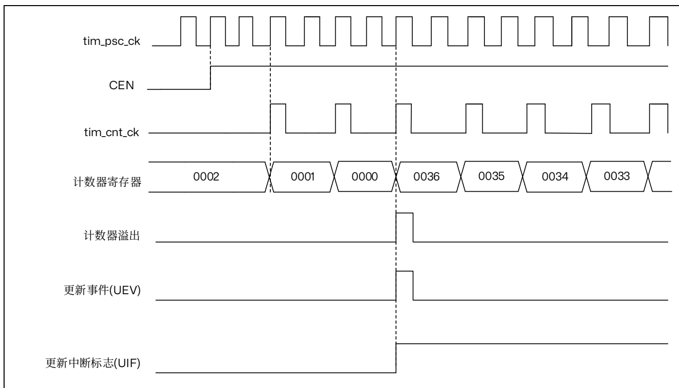
图 15.12 计数器时序图，内部时钟分频因子为 2
