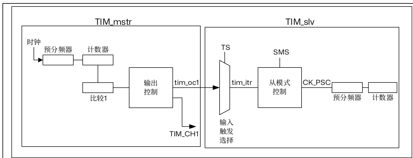
图 15.80 仅定时器通道 1 主/从连接示例
