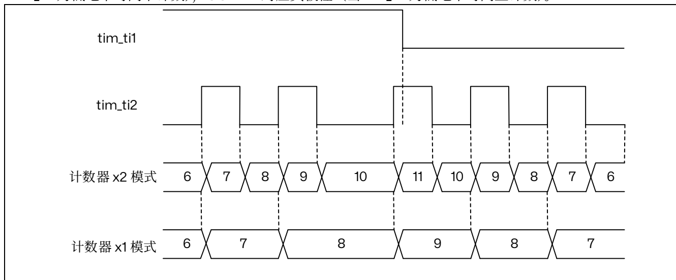
图 15.55 方向加时钟编码器模式
