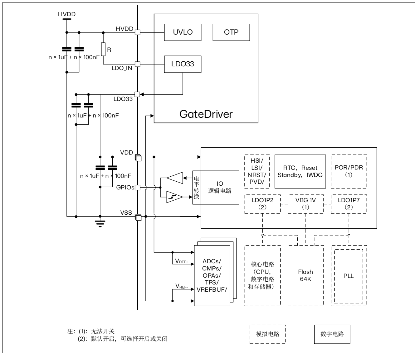
图 6.1 电源框图
