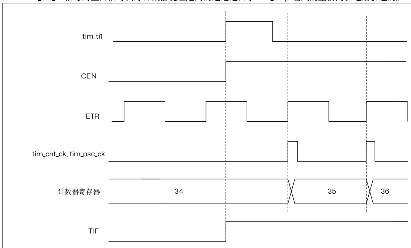
图 15.78 外部时钟模式 2+触发模式下的控制电路
