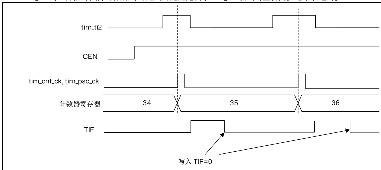
图 15.24 外部时钟模式 1 下的控制电路
