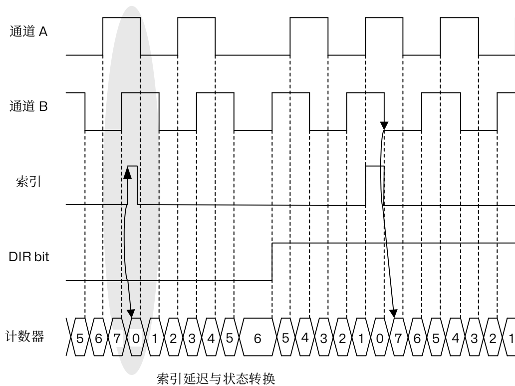
图 15.64 窄索引脉冲情况下的编码器模式行为 (IPOS[1:0] = 11)
