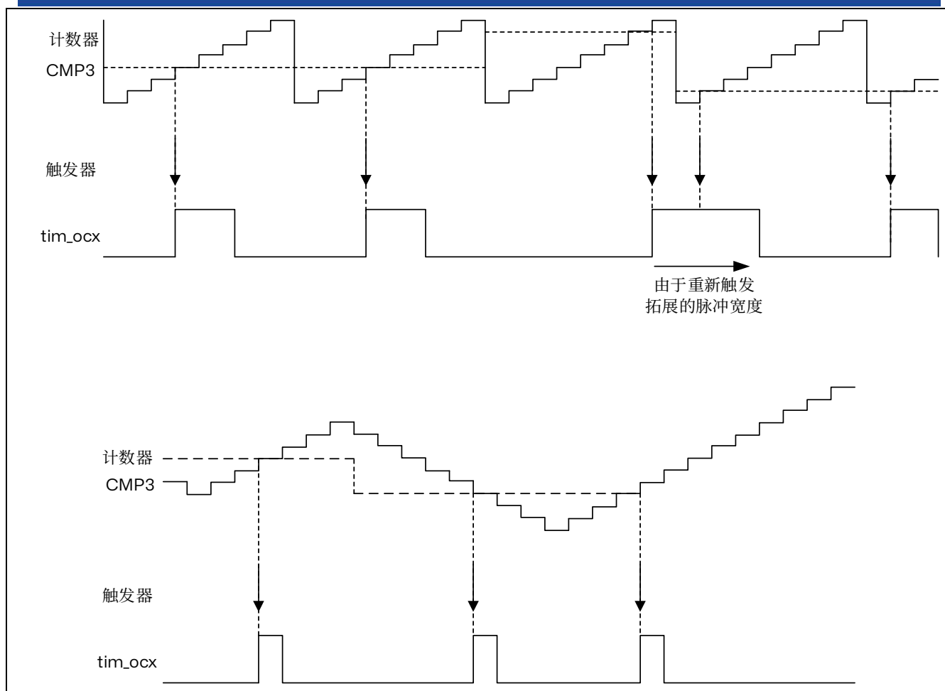
图 15.50 在比较事件上的脉冲生成，适用于边沿对齐模式和编码器模式
