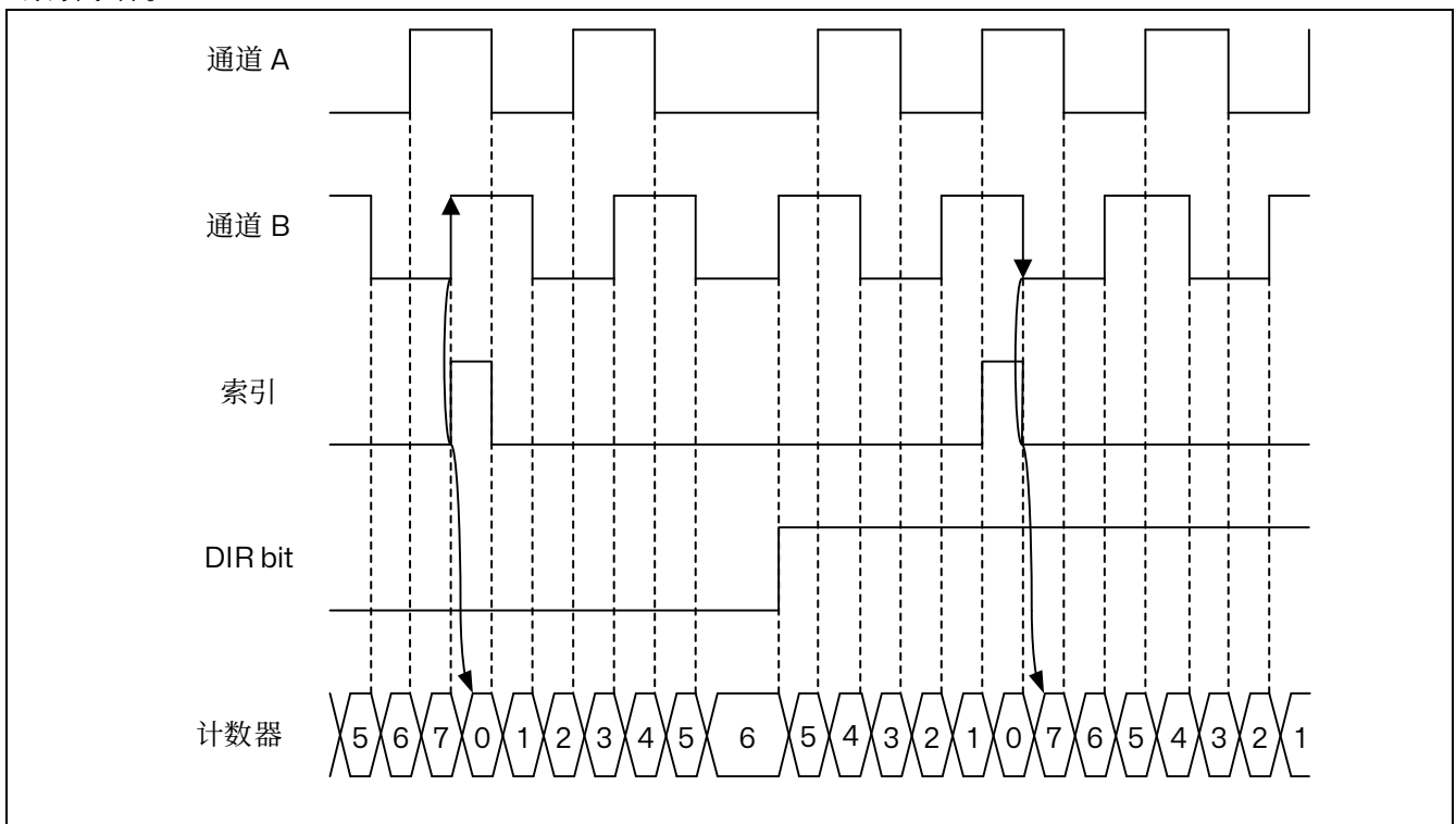
图 15.63 通道 A 和 B 上带索引门控的计数器读取
