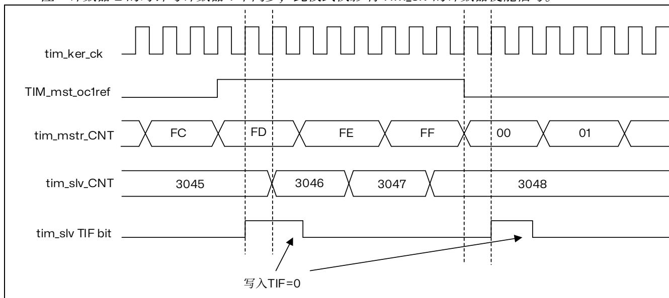
图 15.81 TIM_mstr 的 tim_oc1ref 控制 TIM_slv
