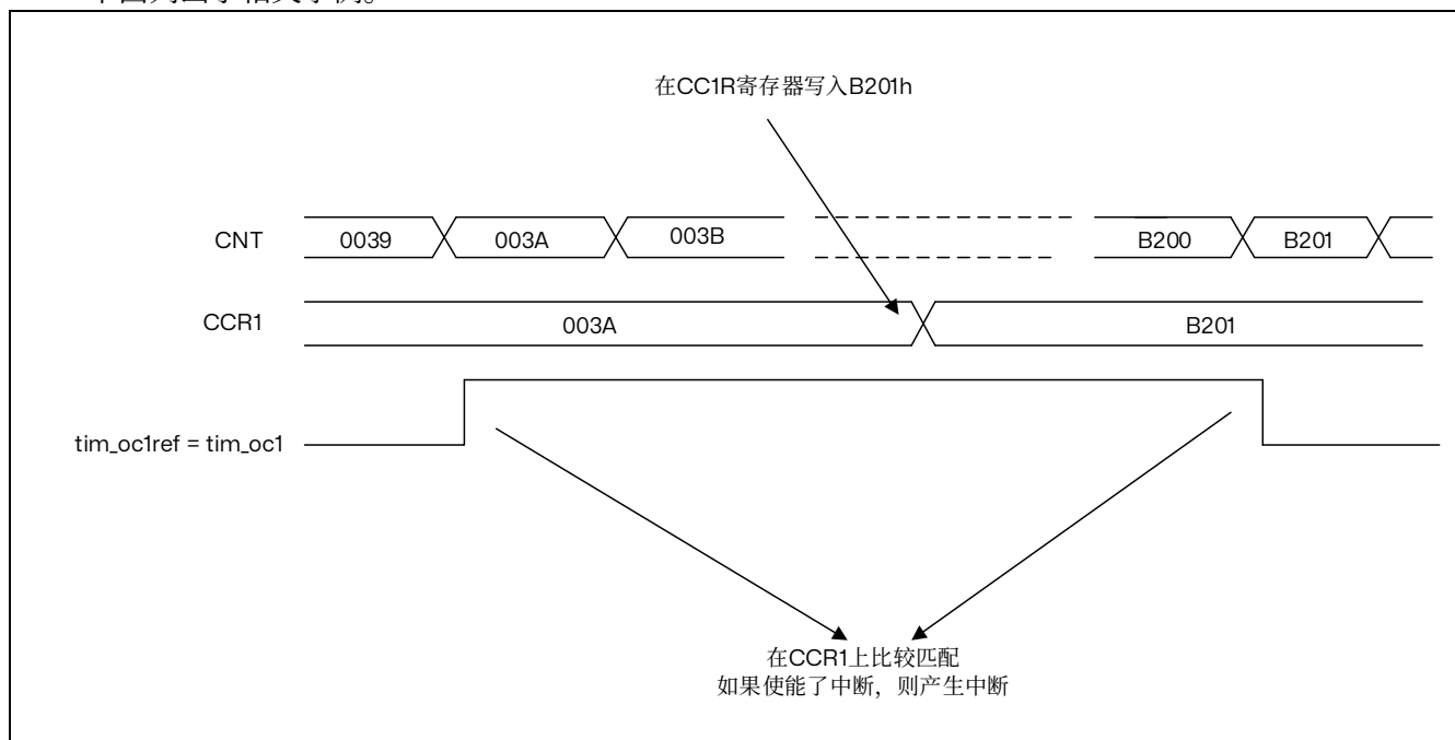
图 15.31 输出比较模式，翻转 tim_oc1
