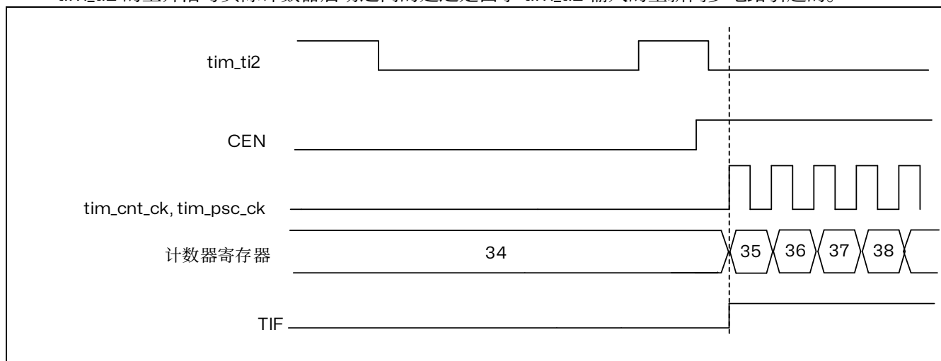
图 15.77 触发器模式下的控制电路
