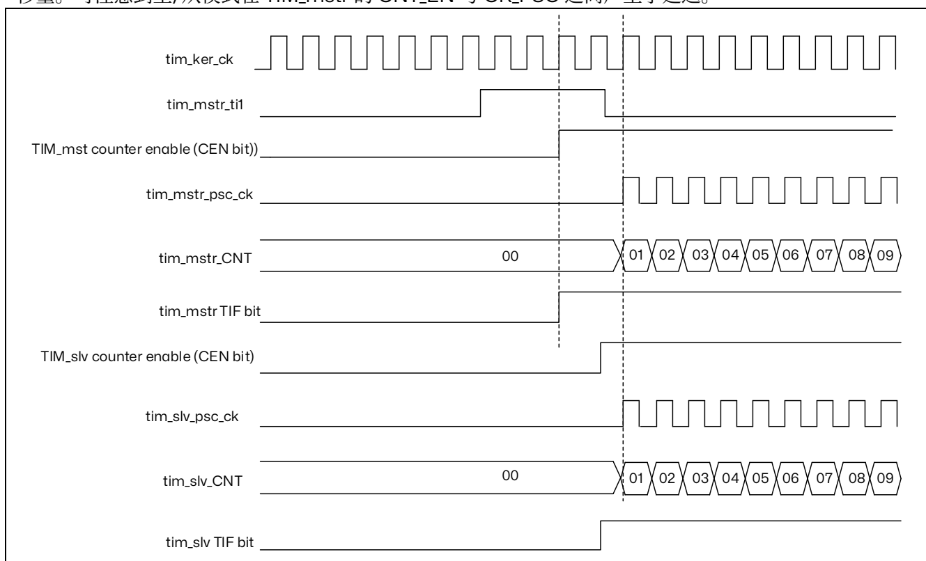
图 15.85 使用 TIM_mstr 的 tim_ti1 输入触发 TIM_mstr 和 TIM_slv
