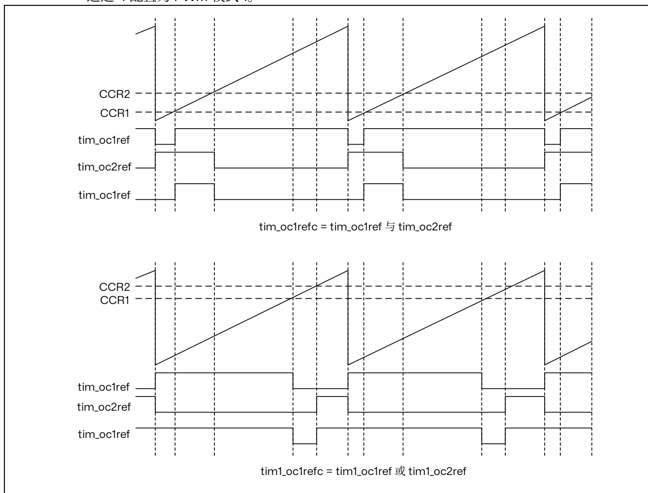
图 15.44 通道 1 和通道 3 的组合 PWM 模式
