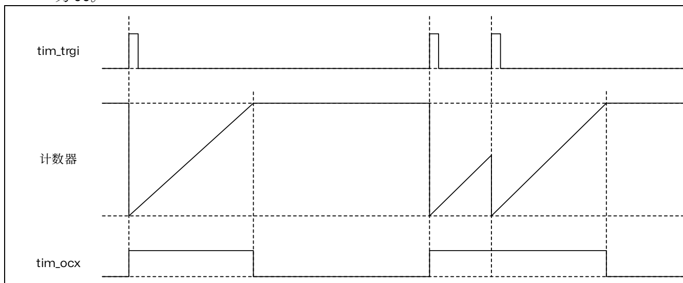
图 15.48 可重触发单脉冲模式
