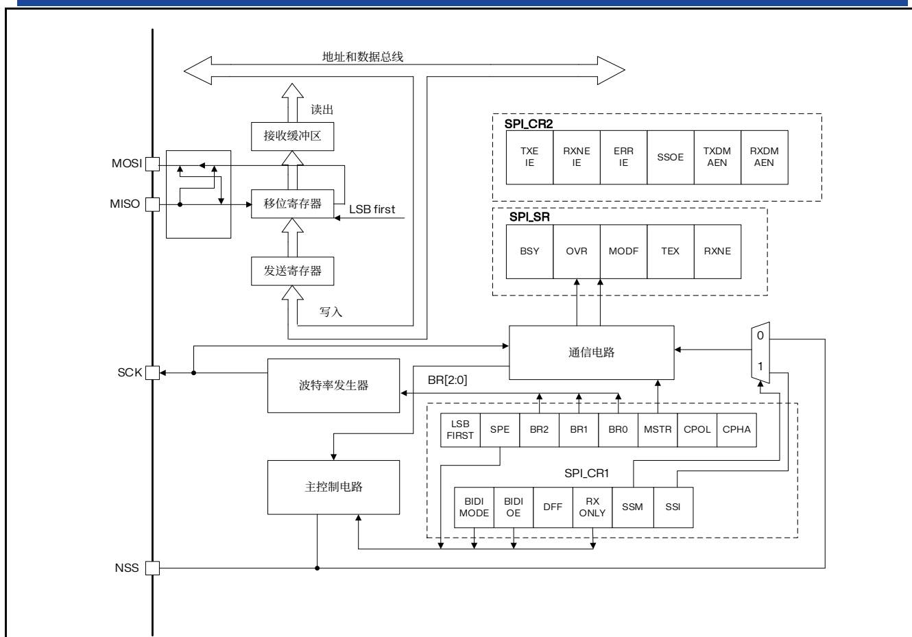
图 23.1 SPI 框图
