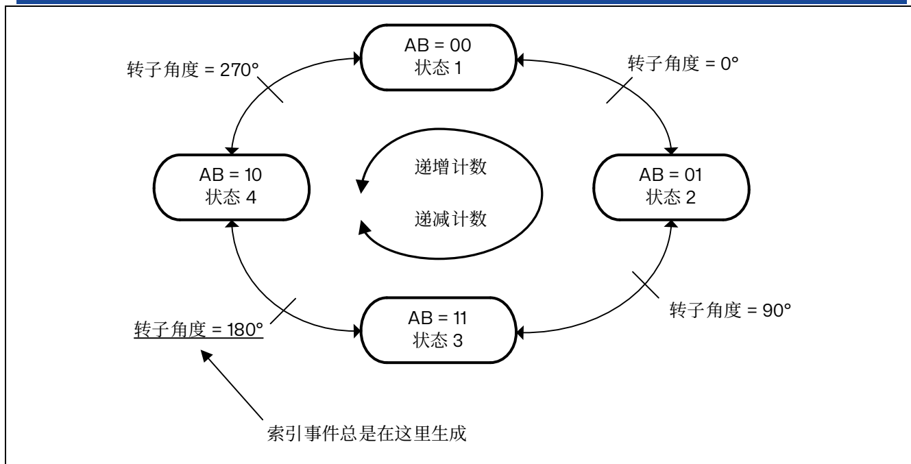
图 15.60 IPOS[1:0] = 11 时的索引生成
