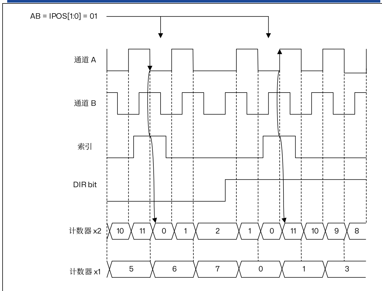
图 15.66 x1 和 x2 模式下的索引行为 (IPOS[1:0] = 01)
