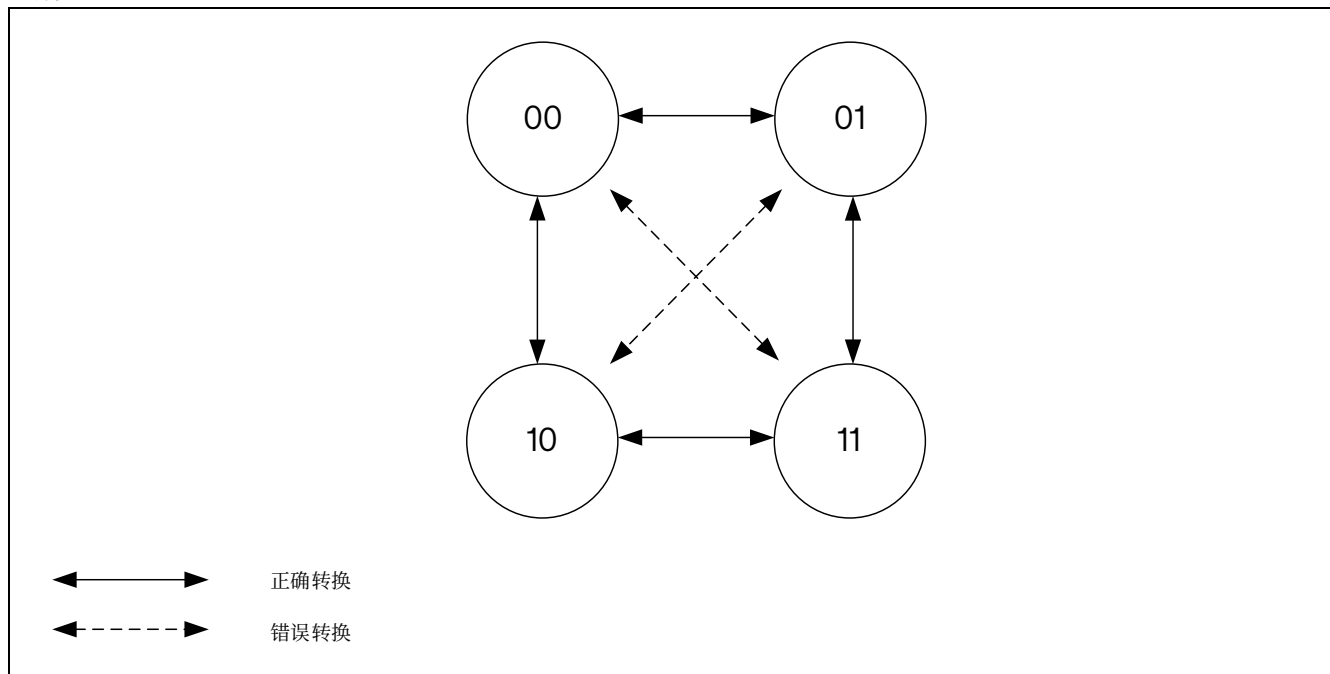
图 15.71 正交编码信号的状态图
