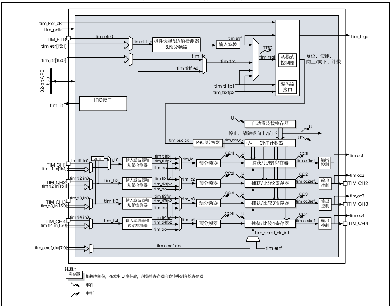
图 15.2 通用定时器 TIM3 框图
