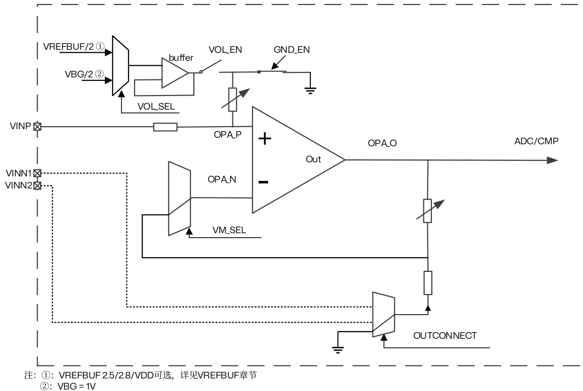
图 18.6 OPAMP1/OPAMP2 PGA 模式 (P-IO, N-GND)
