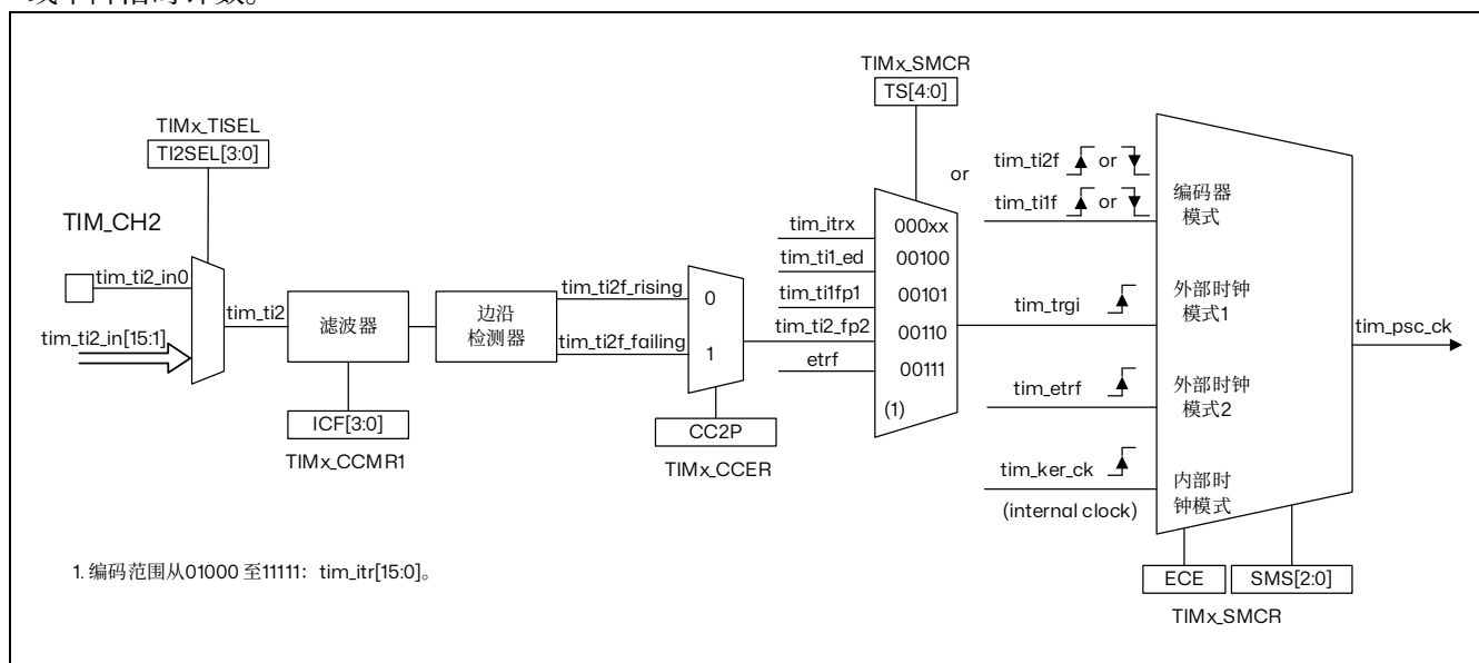
图 15.23 tim_ti2 外部时钟连接例子
