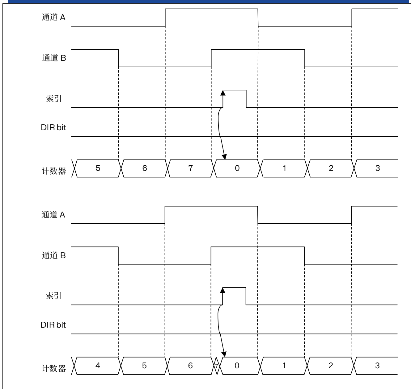
图 15.65 计数器重置窄索引脉冲（更近距离，ARR = 0x07）
