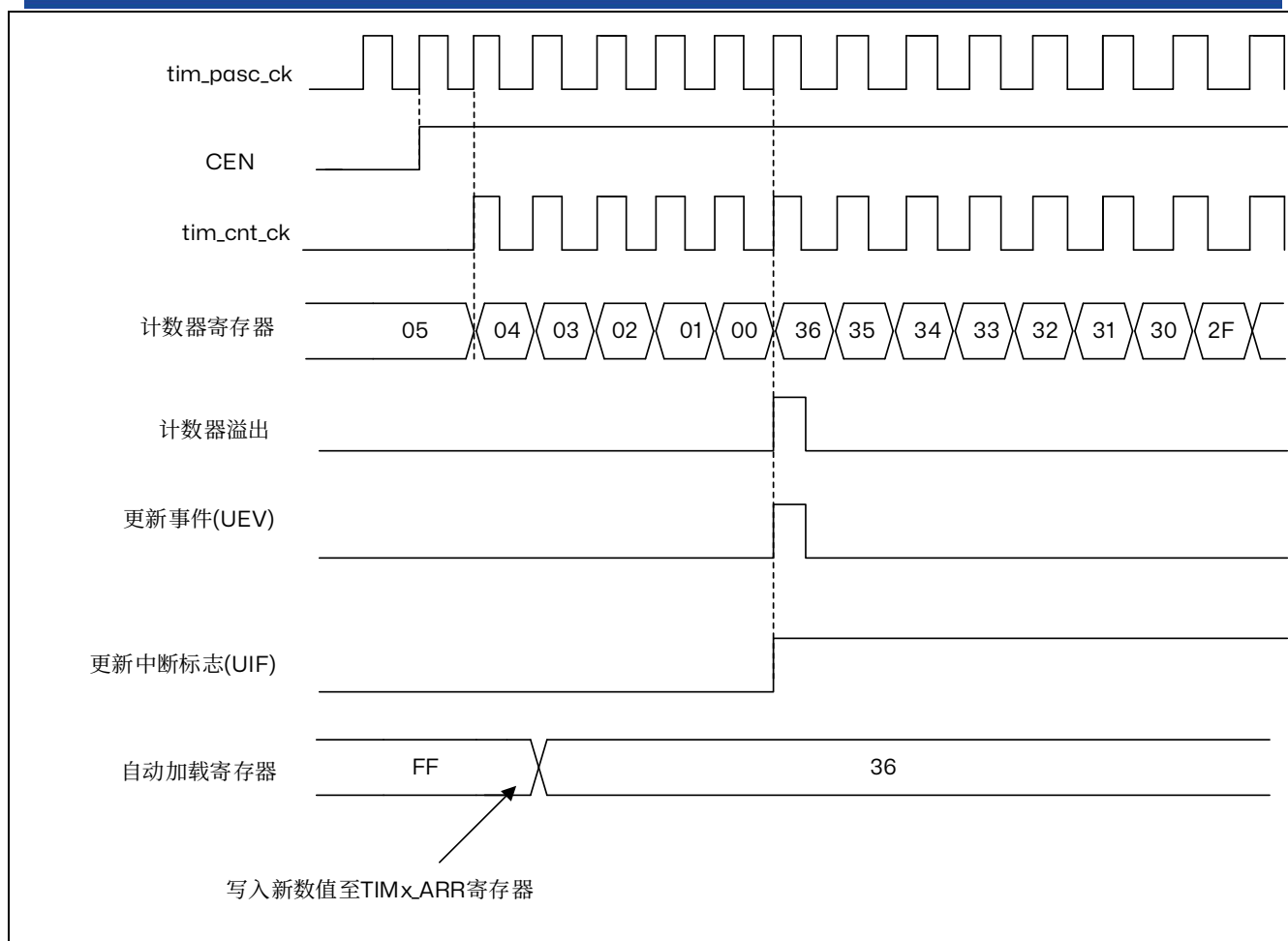
图 15.15 计数器时序图，更新事件
