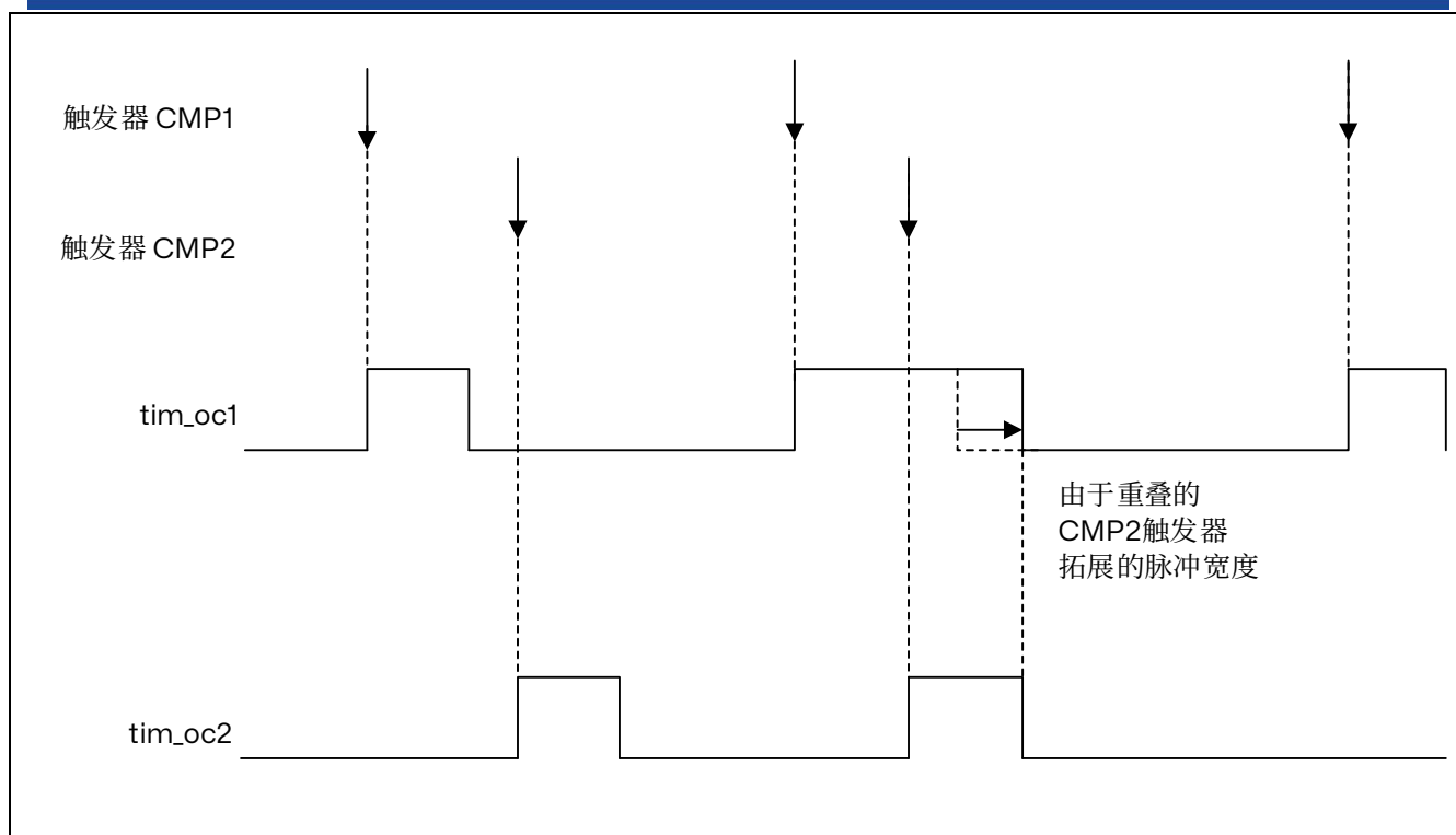
图 15.51 在同时触发的情况下延长脉冲宽度
