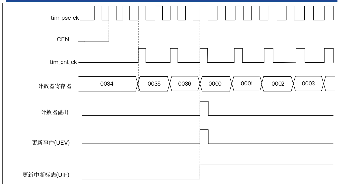
图 15.6 计数器时序图，内部时钟分频因子为 2
