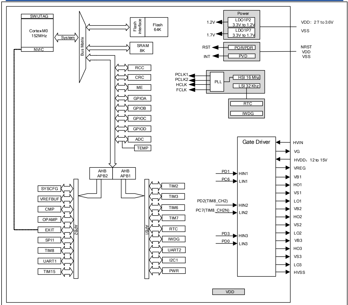
图 2.1 RX32S652 架构图
