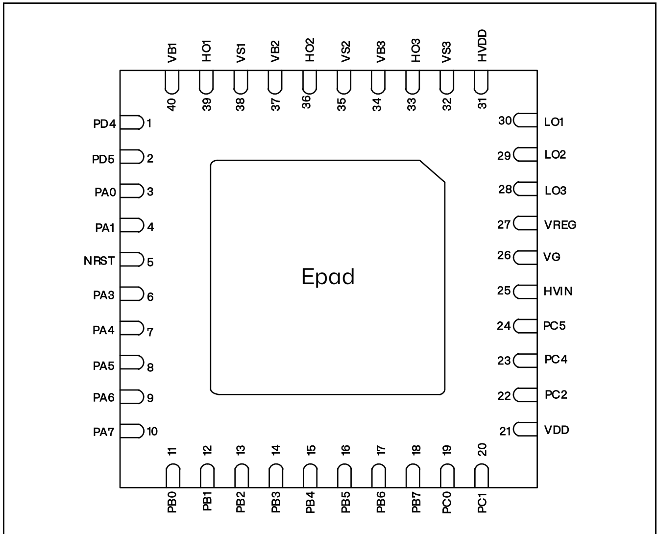
图 4.1 RX32S652 QFN40 引脚图
