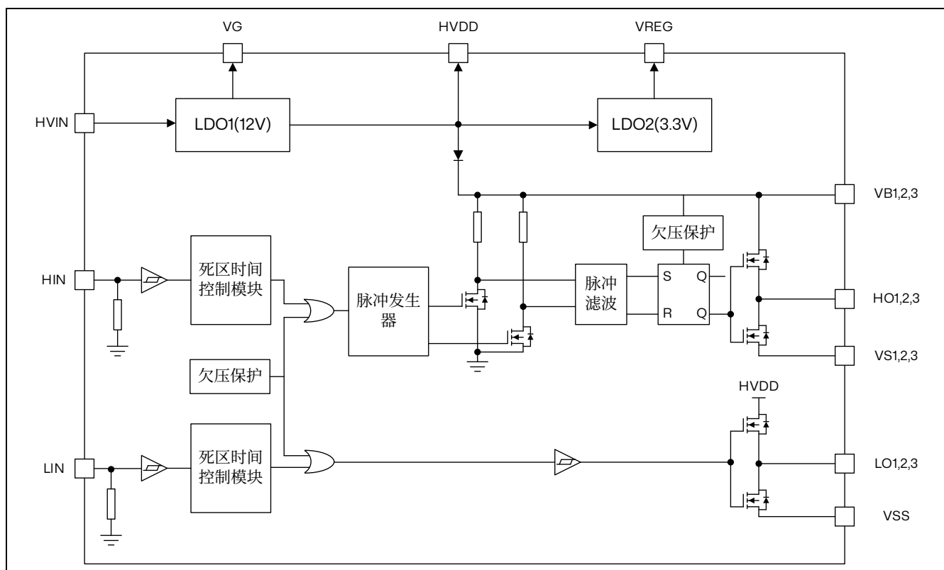
图 5.10 内部结构
