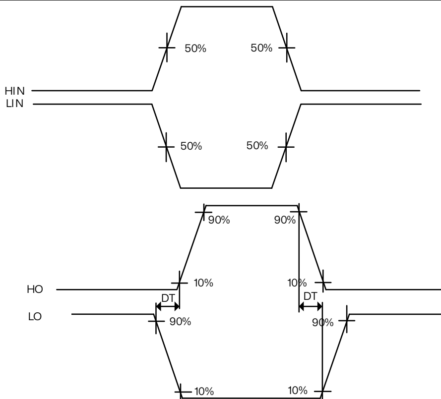
图 5.9 死区时间波形图
