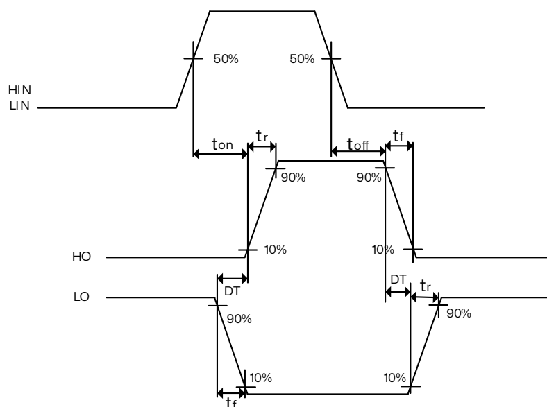
图 5.8 时间切换波形图
