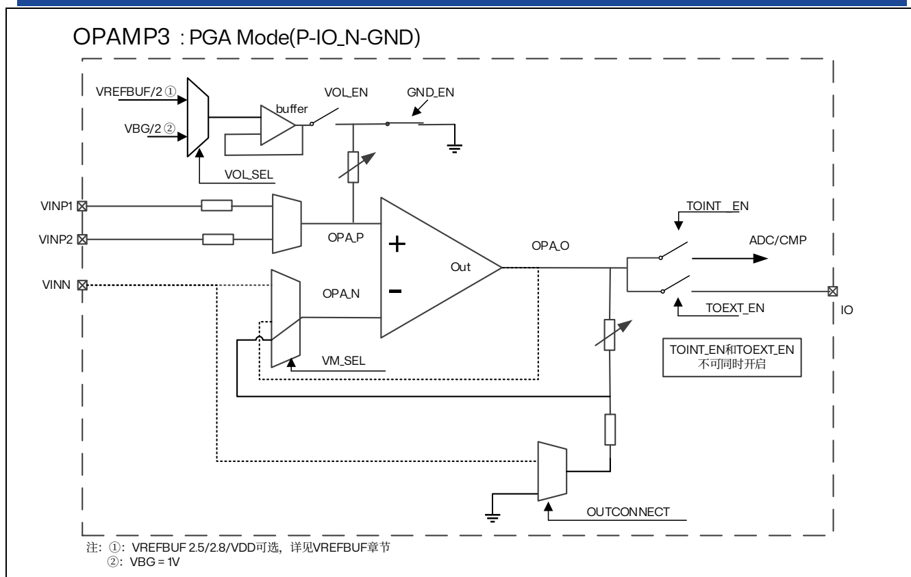
图 18.7 OPAMP3 PGA 模式 (P-IO, N-GND)
