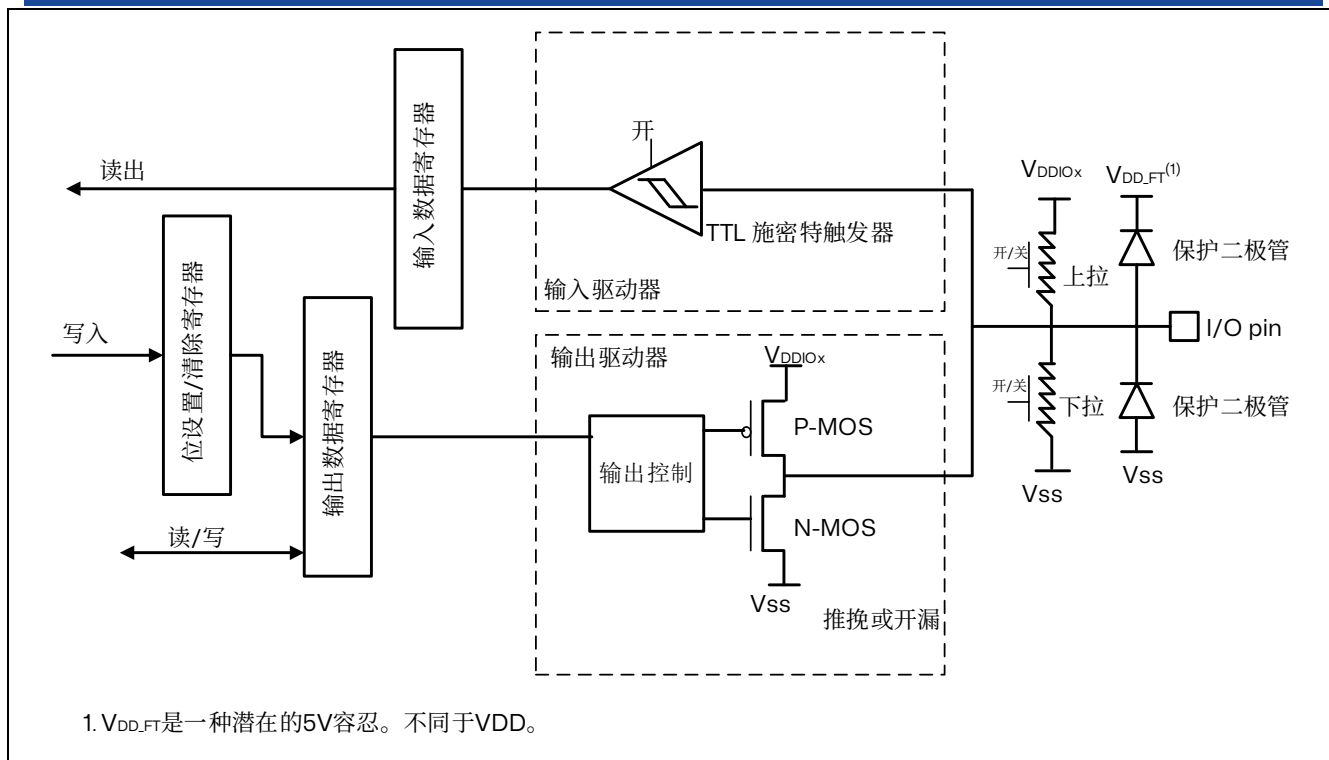
图 8.3 输出框图
