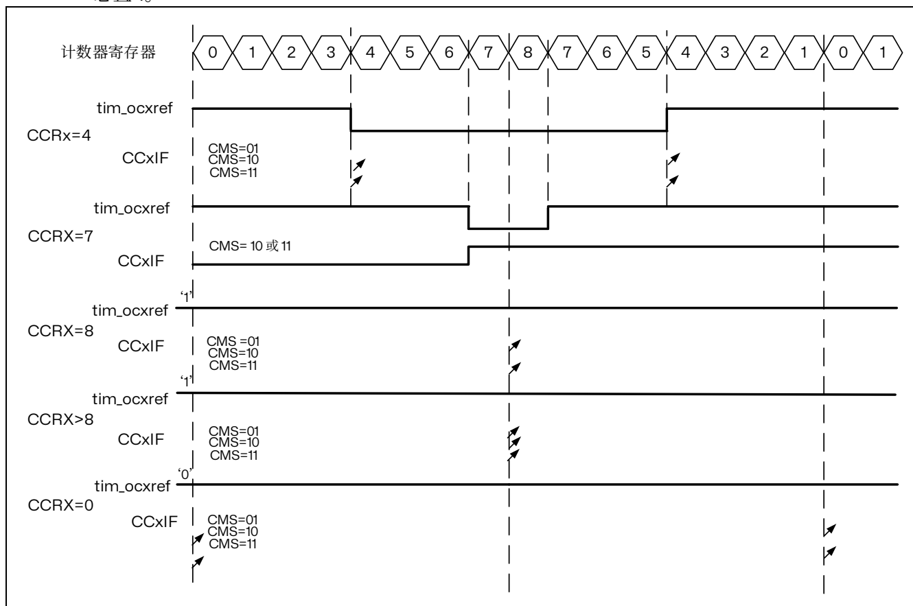
图 15.32 中央对齐的 PWM 波形 (APR=8)
