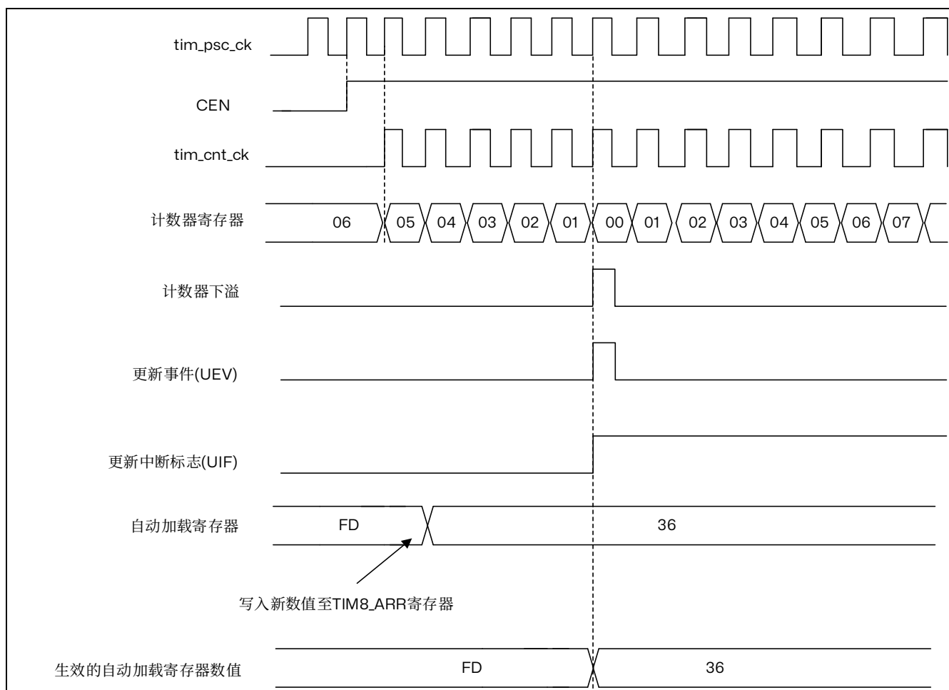
图 14.18 计数器时序图，内部时钟分频因子为 N
