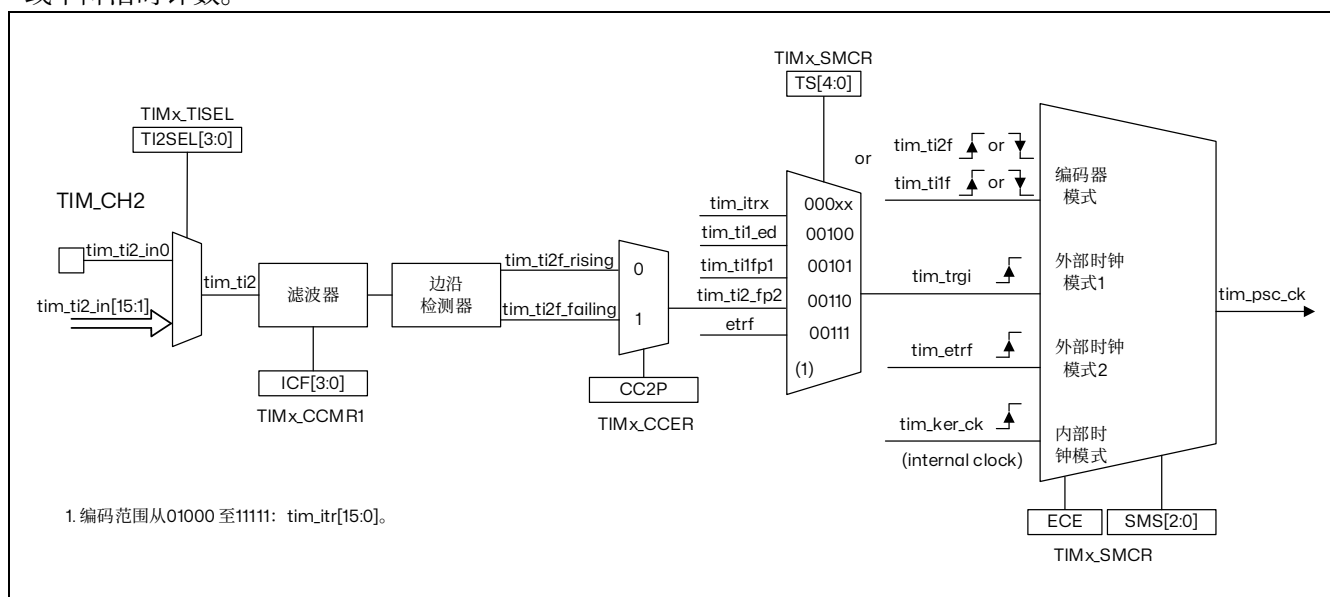
图 15.22 tim_t2 外部时钟连接例子
