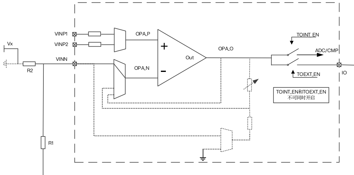
图 18.1 OPAMP3 独立模式
