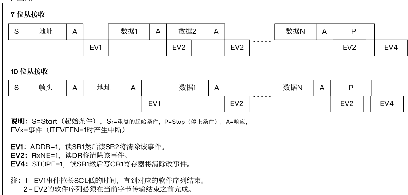
图 24.4 从接收器的传送序列图
