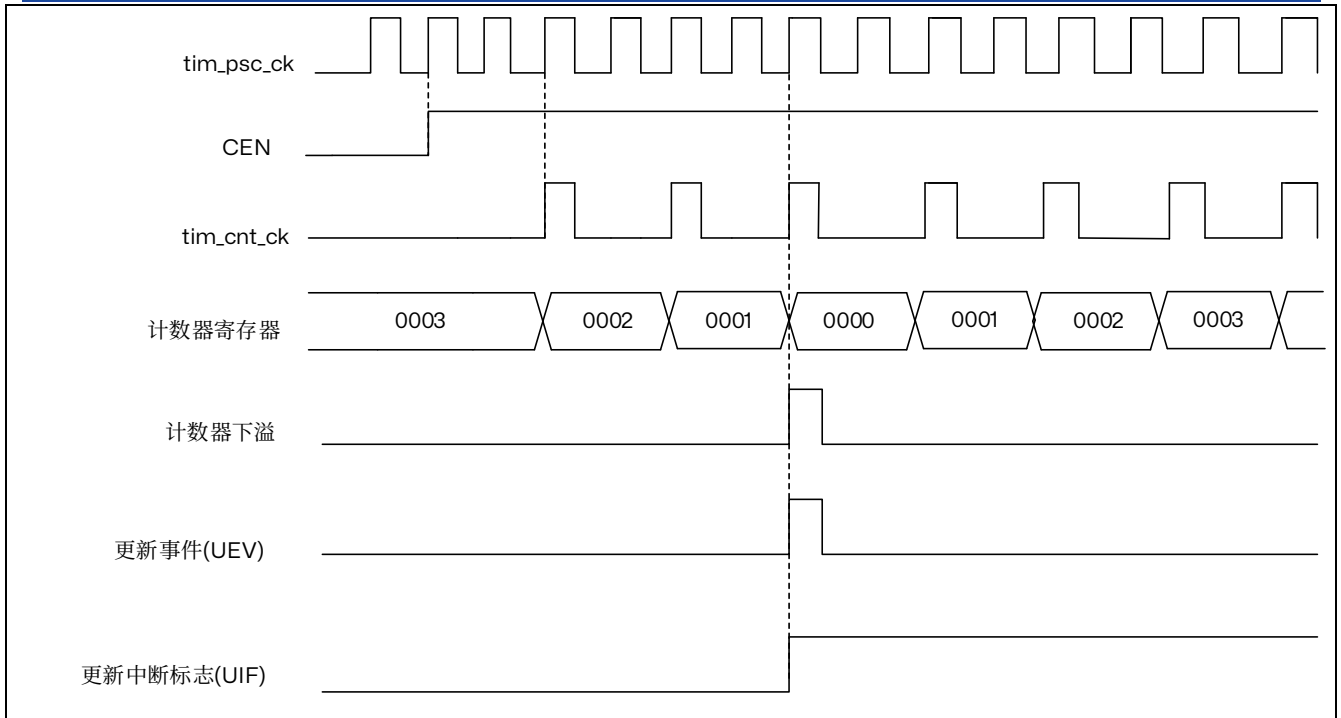
图 15.16 计数器时序图，内部时钟分频因子为 2
