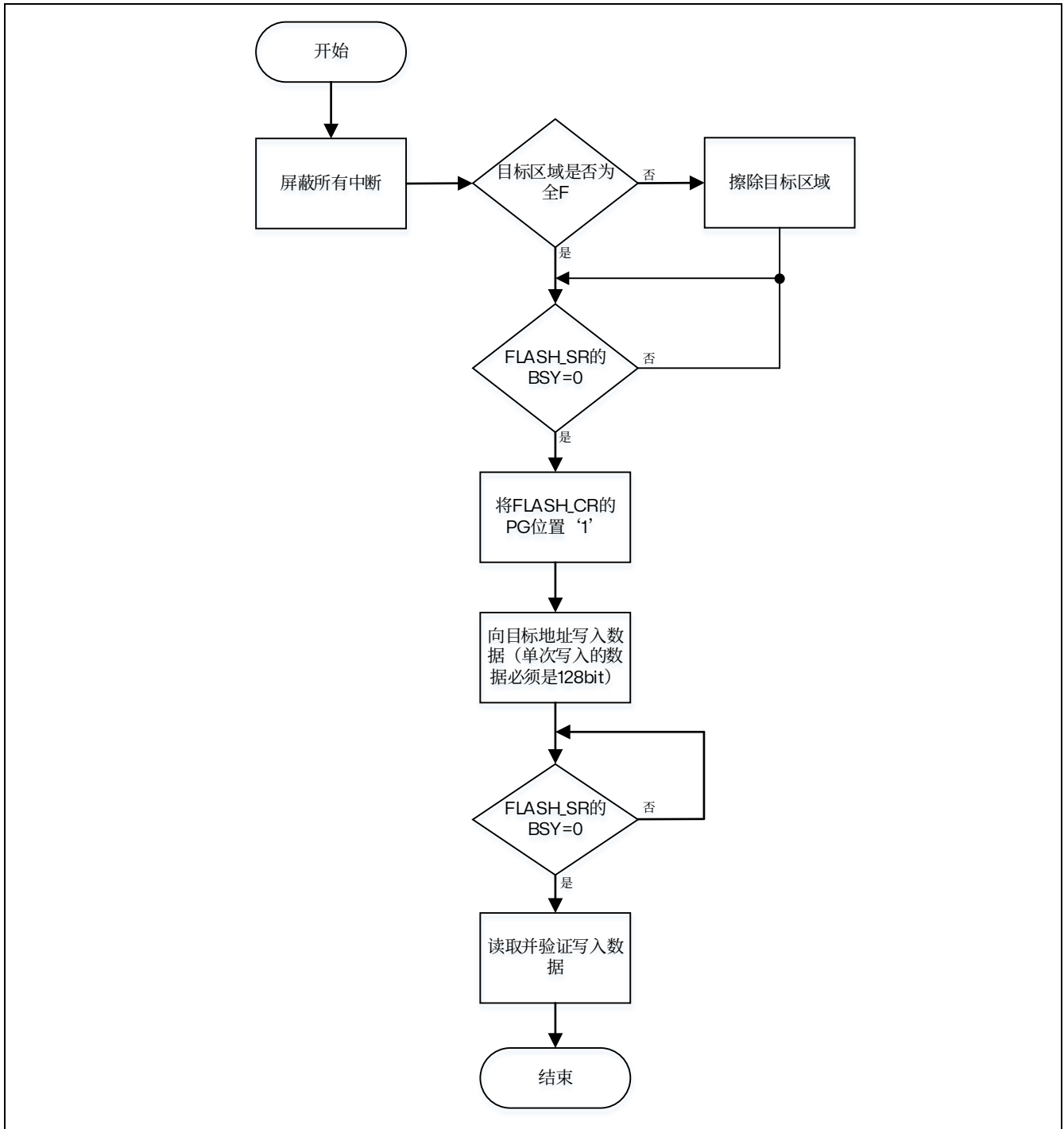
图 4.3 FLASH 写入流程
