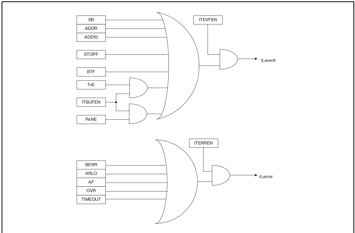
图 24.7 I 2 C 中断映射图
