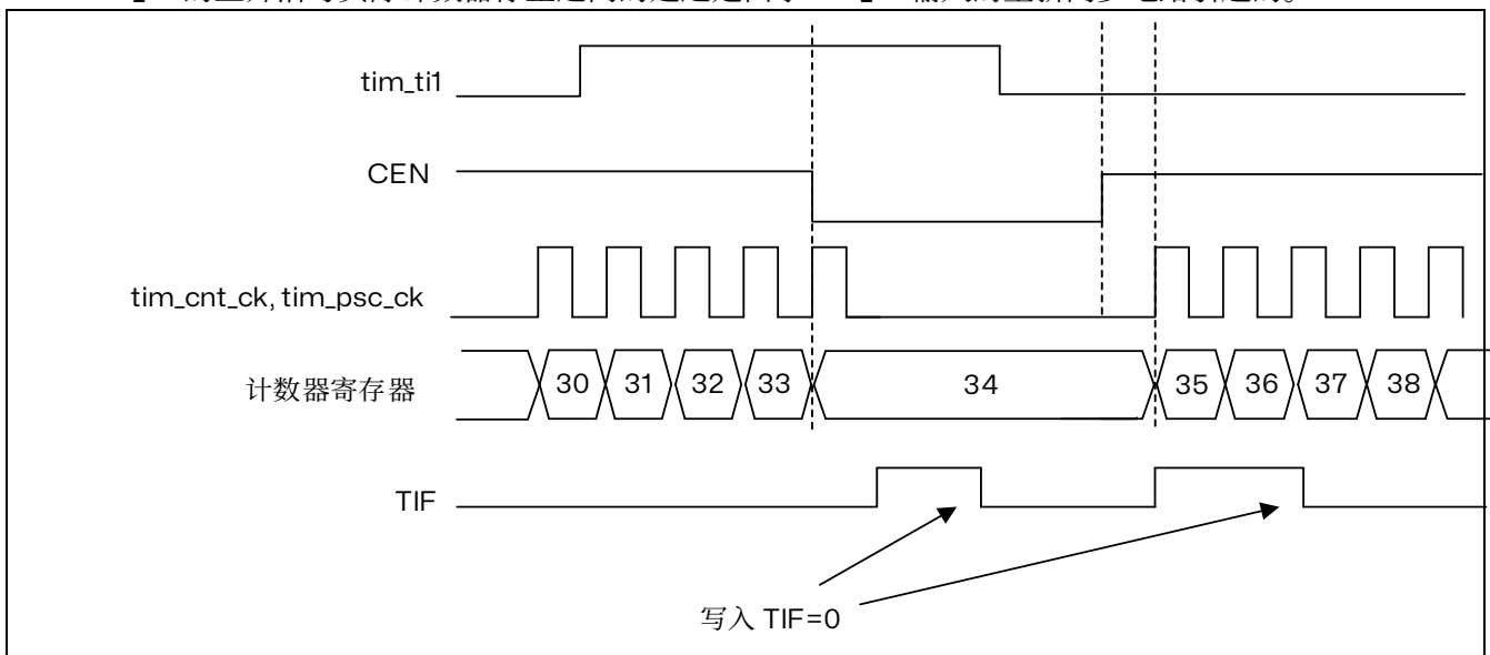
图 15.75 门控模式下的控制电路
