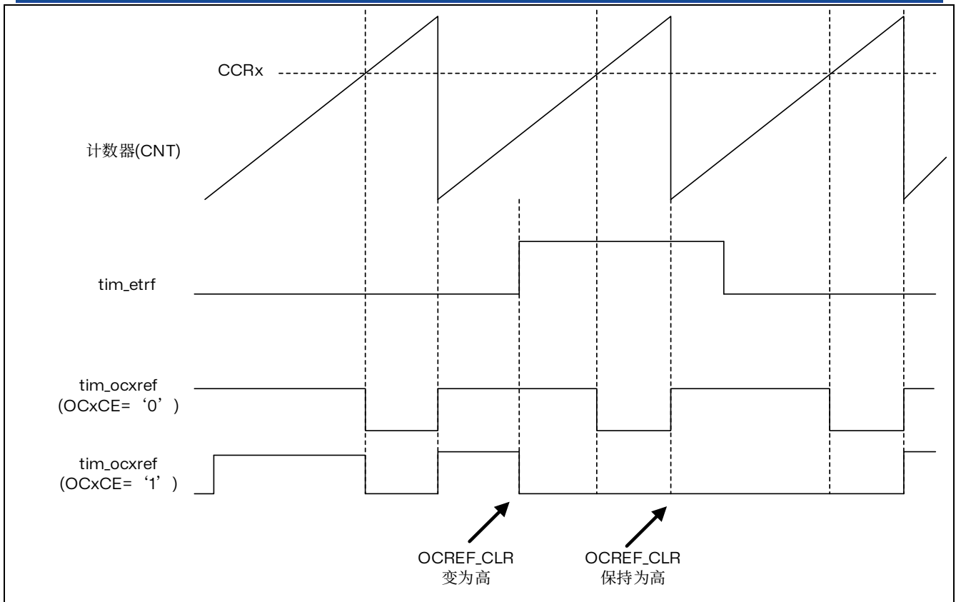
图 15.45 清除 TIMx 的 tim_ocxref
