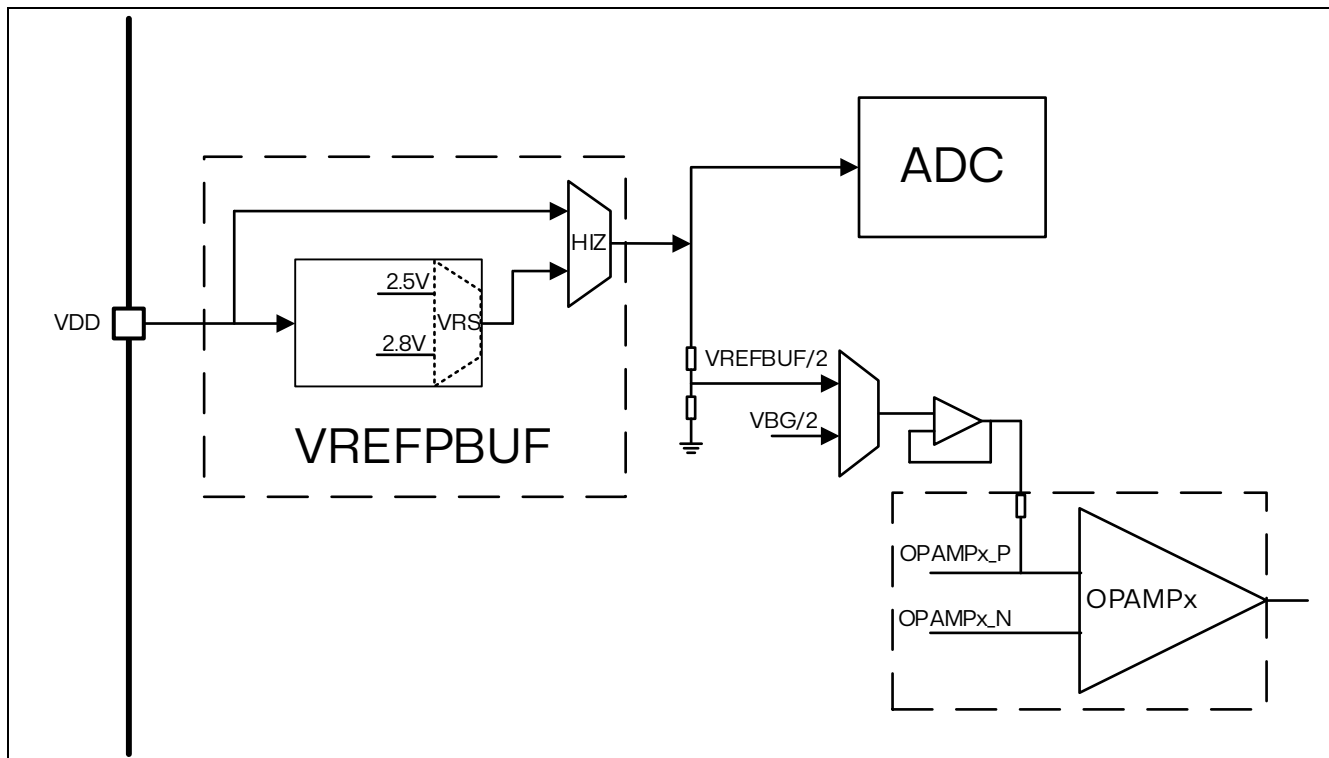
图 12.1 VREFBUF 框图
