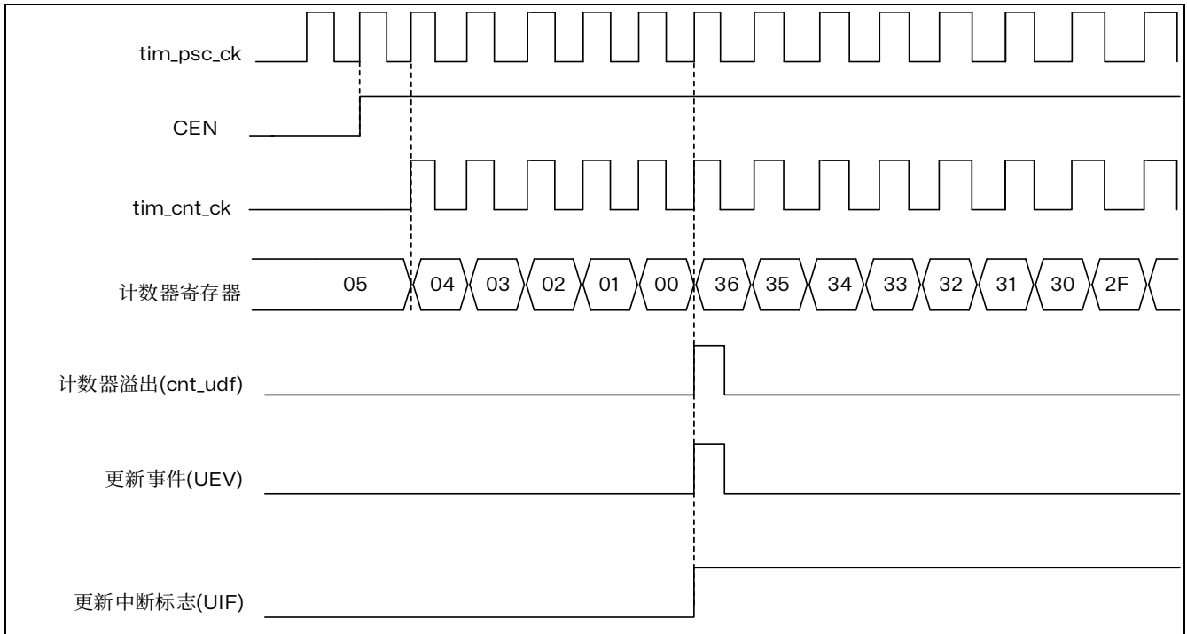
图 14.10 计数器时序图，内部时钟分频因子为 1
