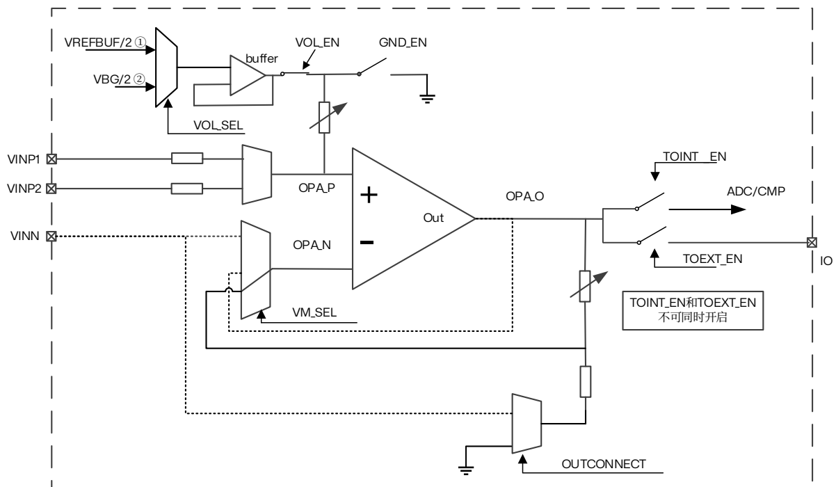
图 18.9 OPAMP3 PGA 模式 (P-偏置, N-GND)
