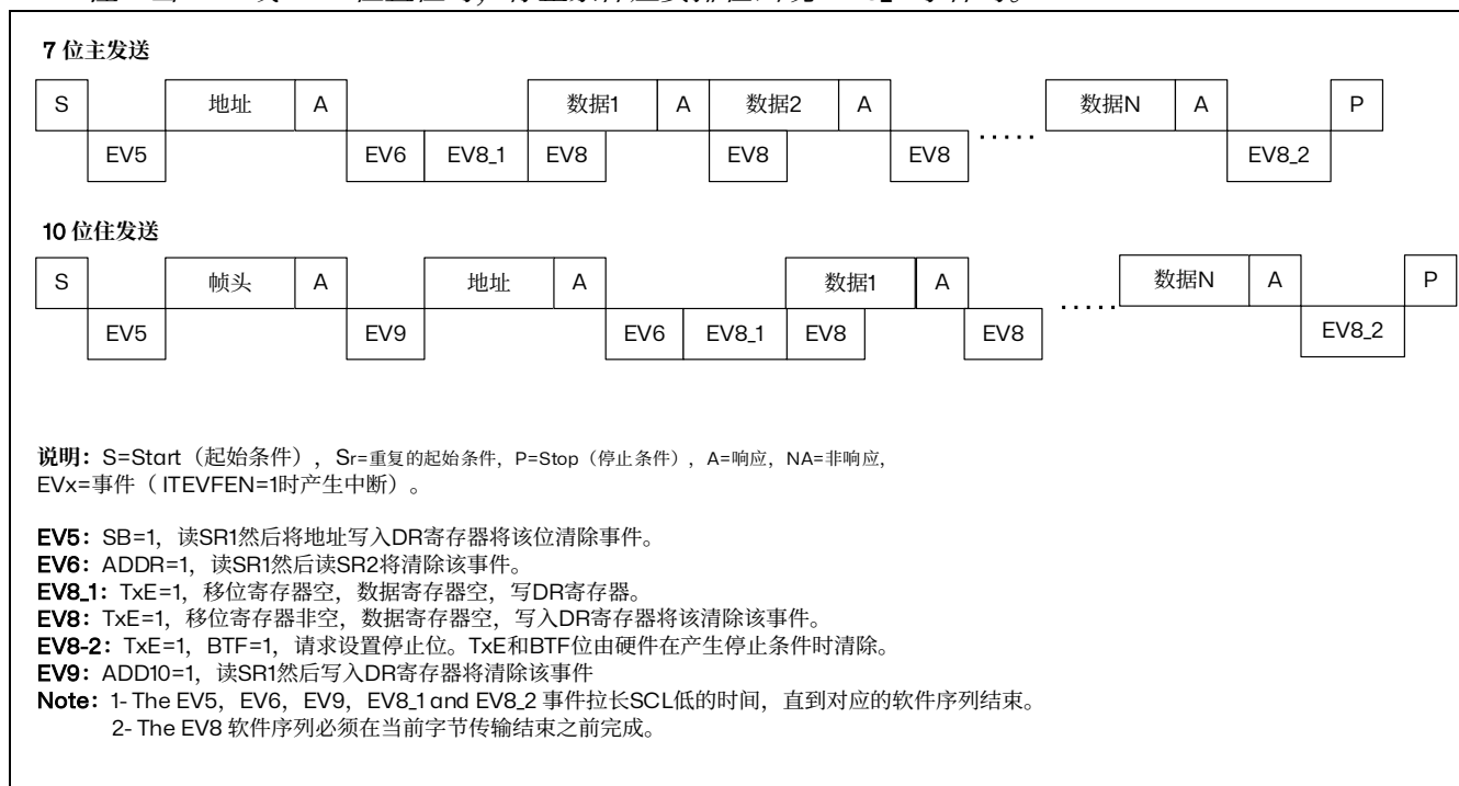
图 24.5 主发送器传送序列图
