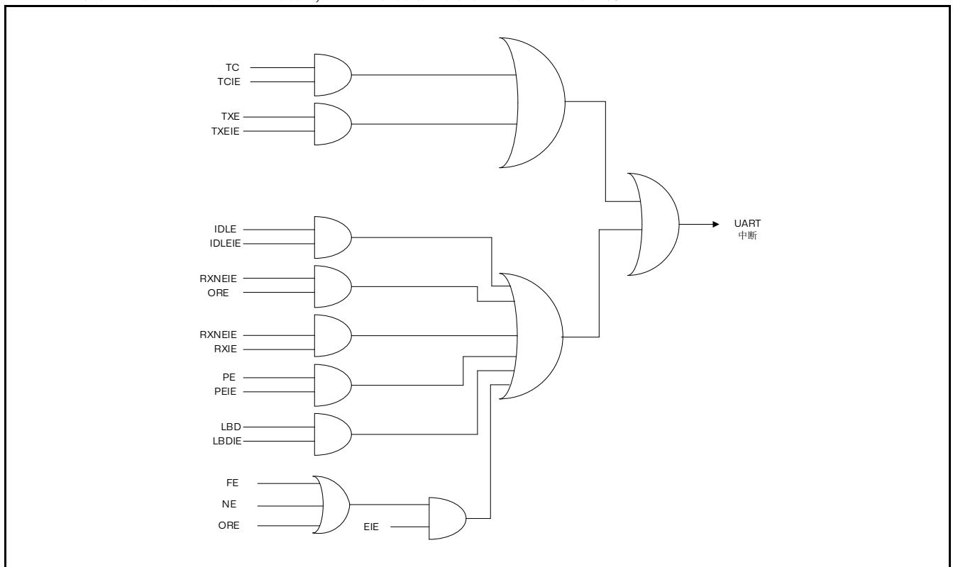
图 25.9 UART 中断映像图
