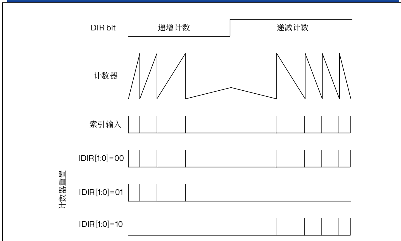
图 15.66 定向索引灵敏度
