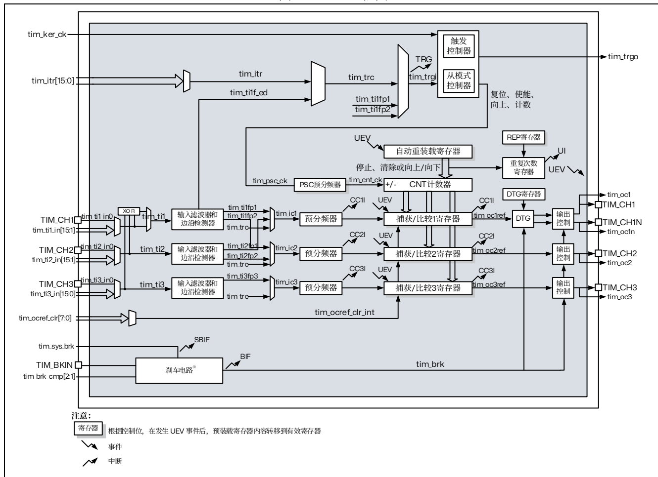
图 16.1 TIM15 框图
