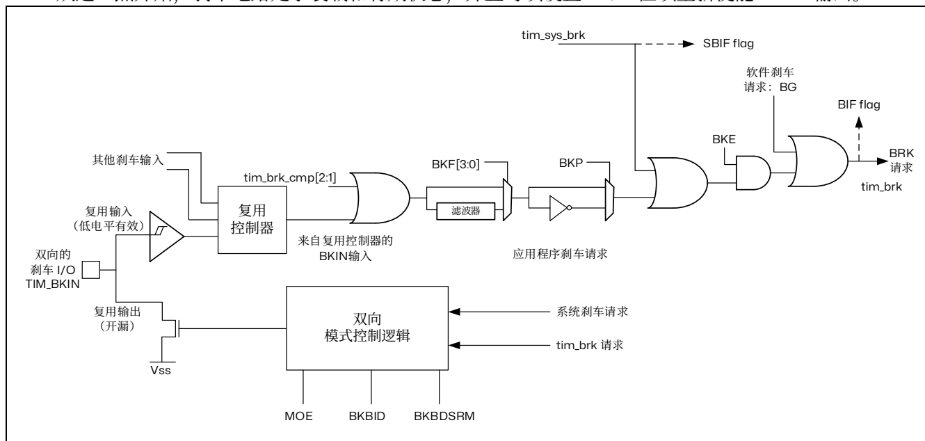
图 14.50 输出重定向（未表示 tim_brk2 请求）
