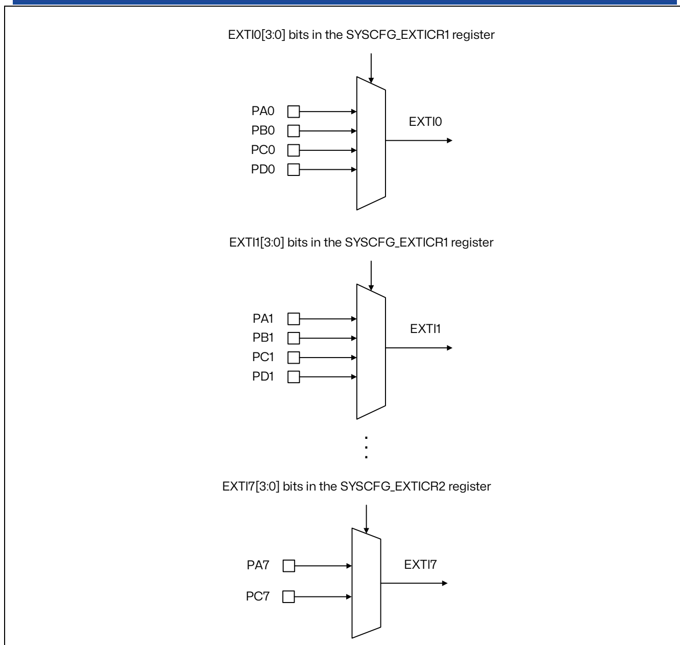
图 11.2 外部中断通用 I/O 映像
