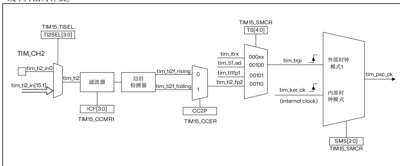
图 16.12 tim_ti2 外部时钟连接例子
