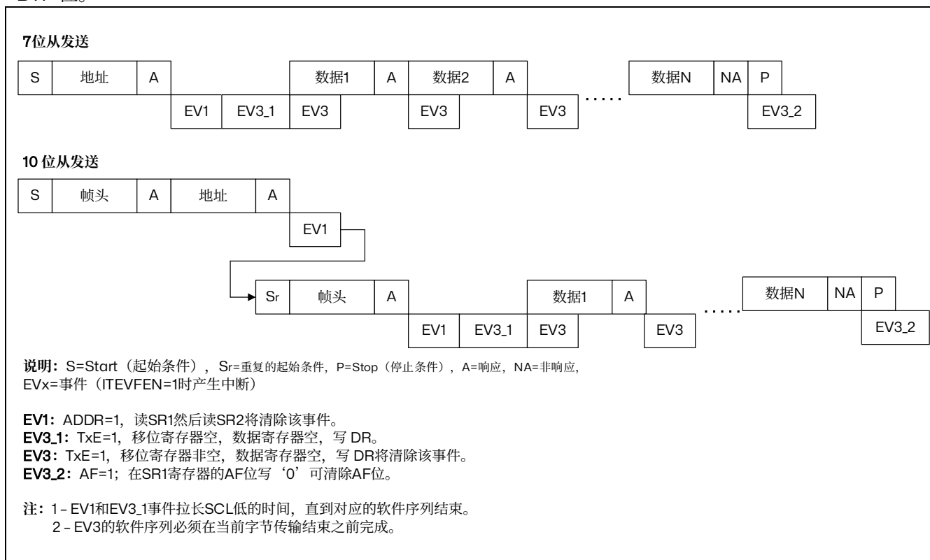
图 24.3 从发送器的传送序列图
