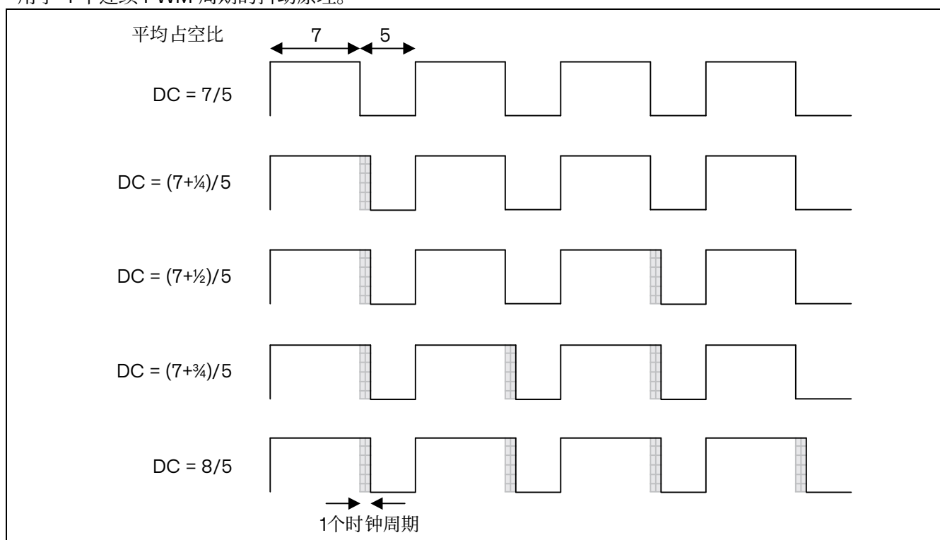
图 14.32 抖动原理
