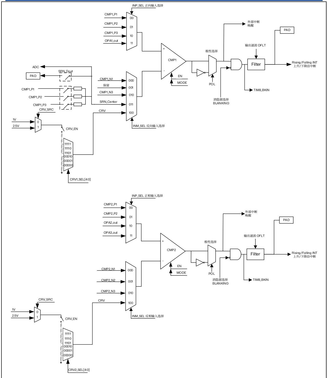
图 19.1 比较器框图
