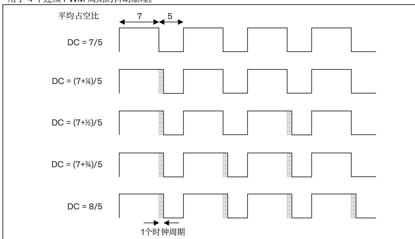
图 15.33 抖动原理
