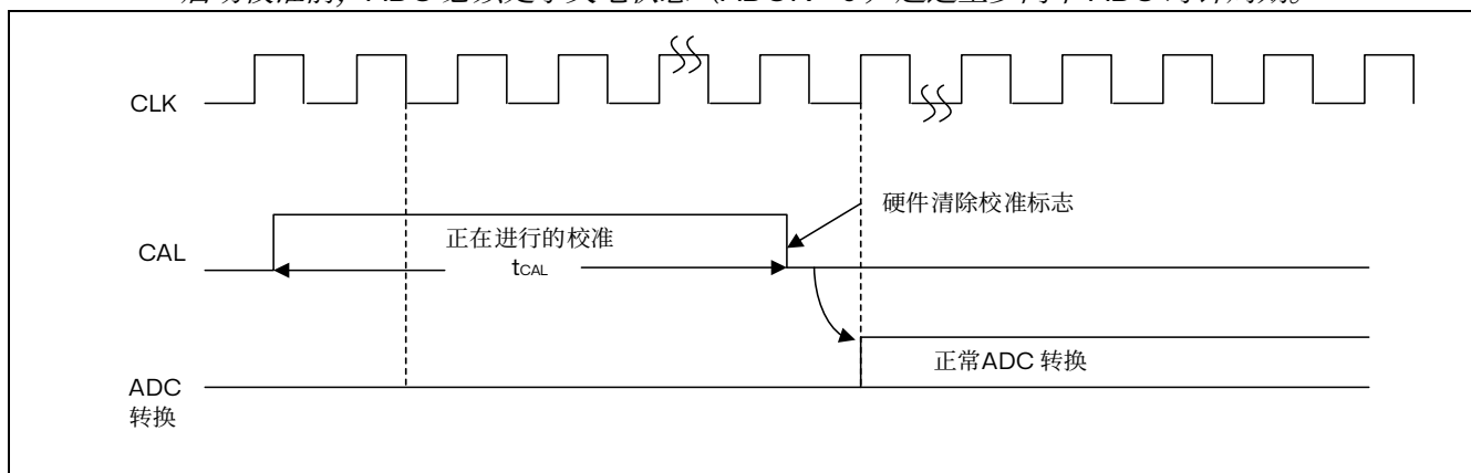
图 13.5 校准时序图
