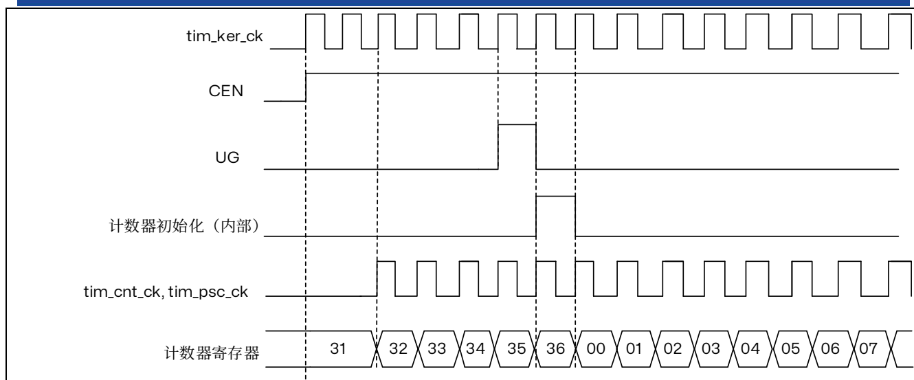
图 15.21 一般模式下的控制电路，内部时钟分频因子为 1
