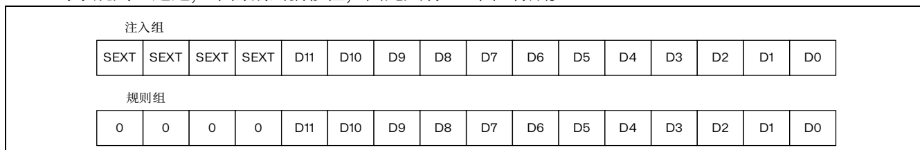
图 13.6 数据右对齐
