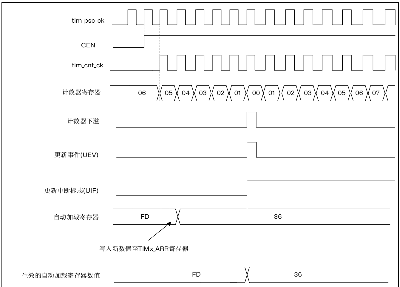
图 15.18 计数器时序图，内部时钟分频因子为 N
