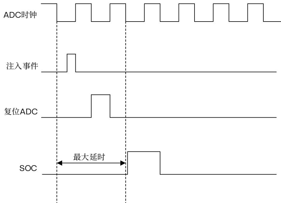
图 13.4 注入转换延迟
