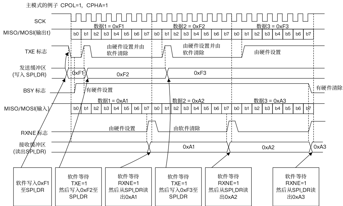
图 23.5 主模式、全双工模式下 (BIDIMODE=0 并且 RXONLY=0) 连续传输时, TXE/RXNE/BSY 的变化示意图
