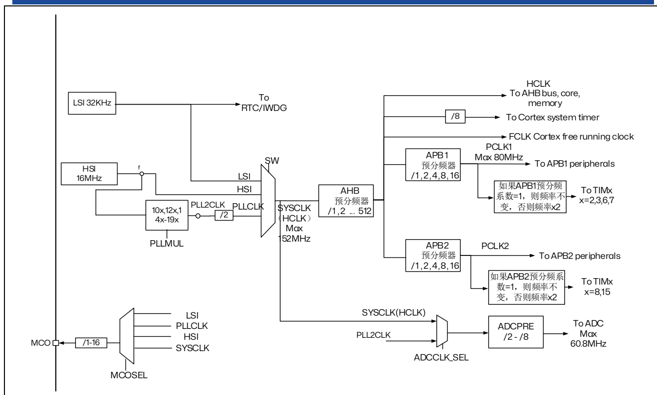
图 7.2 时钟树
