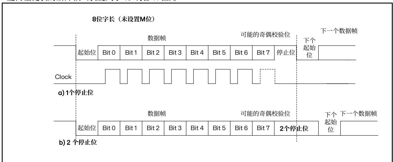
图 25.3 配置停止位
