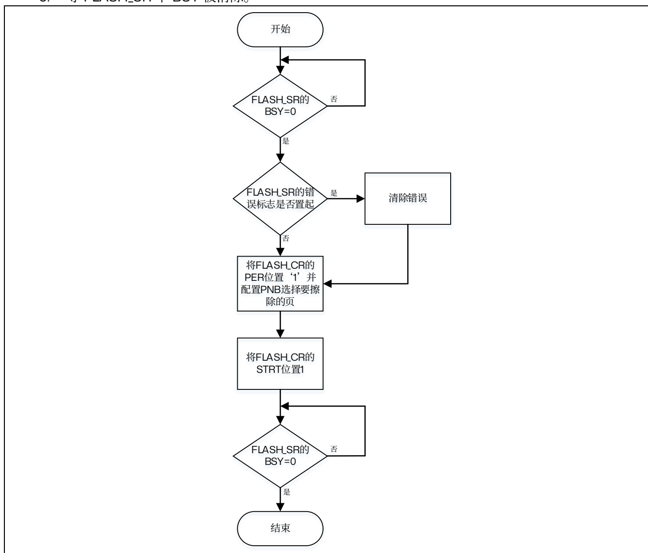
图 4.1 页擦流程
