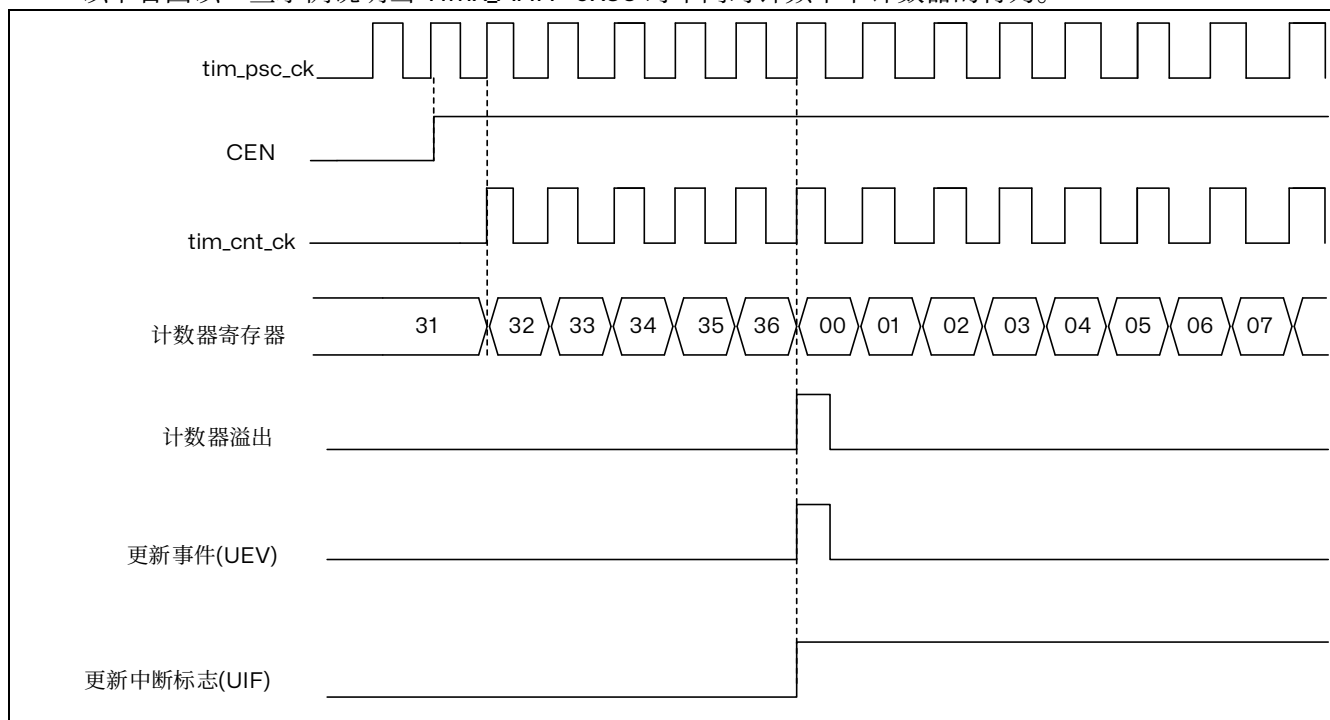
图 15.4 计数器时序图，内部时钟分频因子为 1
