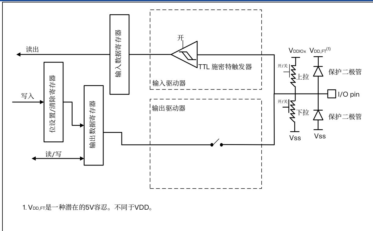
图 8.2 输入浮空/上拉/下拉结构
