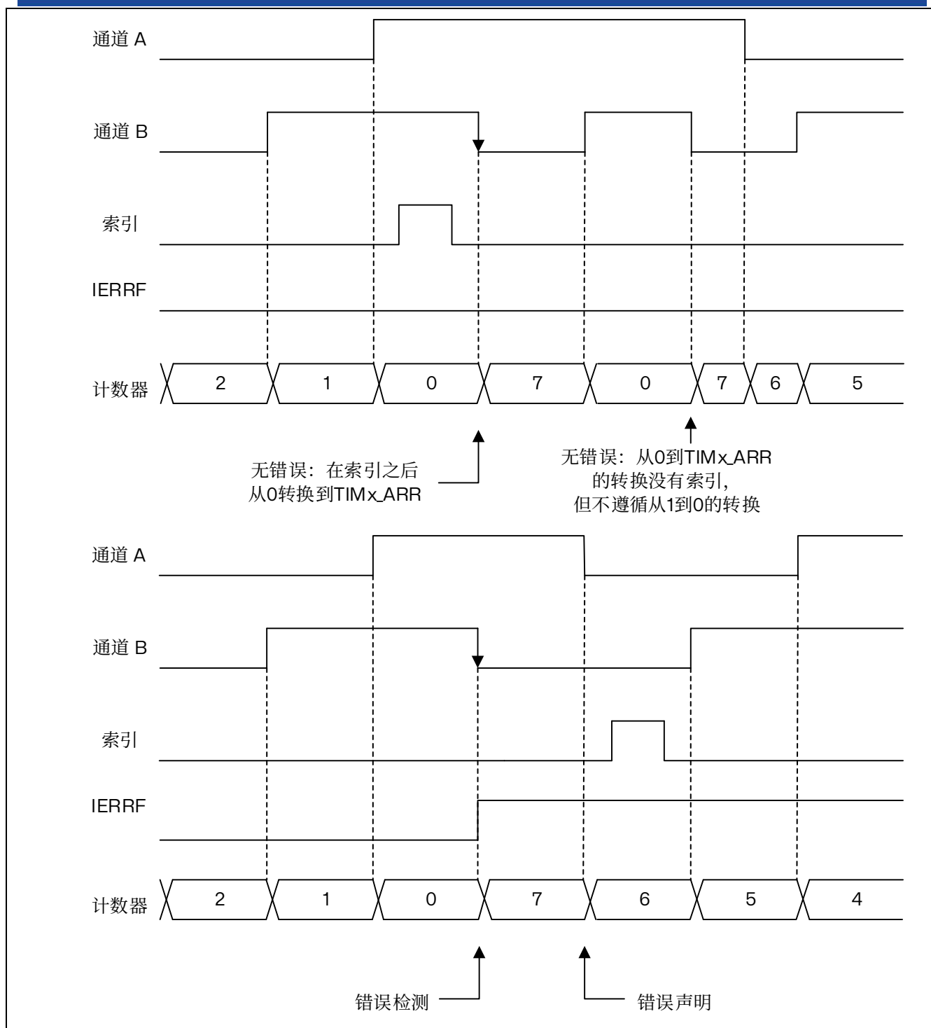
图 15.72 递减计数编码器错误检测
