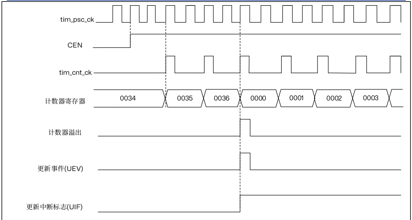
图 16.5 计数器时序图，内部时钟分频因子为 2
